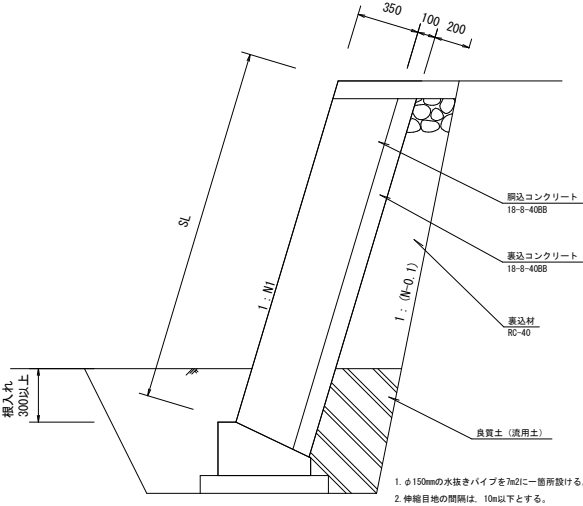
コンクリートブロック積工 (mあたり)
