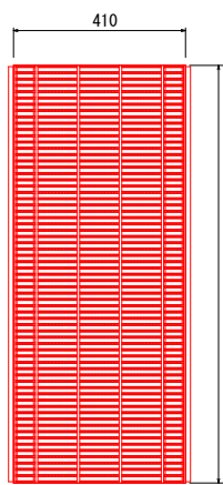
コンクリート蓋、グレーチング蓋 S=1:20 落ちふた式U型側溝3種ふた300 ノンスリップかさがあげ、T-25、細目ゴム付
