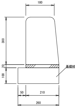
歩車道境界ブロック C S=1:10
