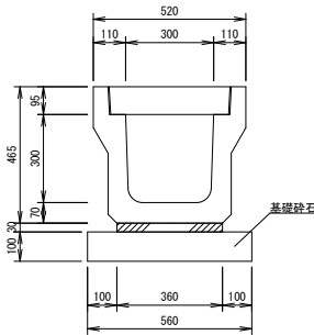
車線分離標 S=1:10
