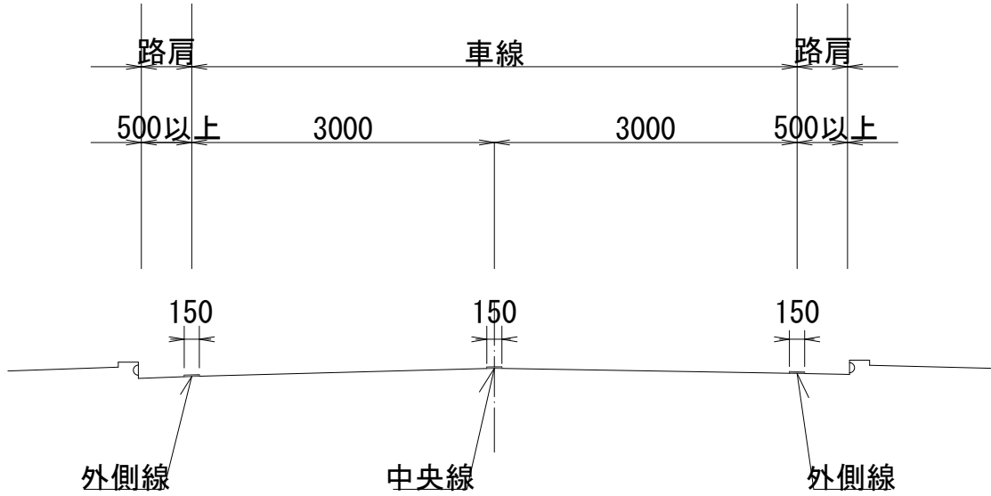
標 準 断 面 図
