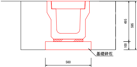
U型側溝掘付工 (mあたり)
