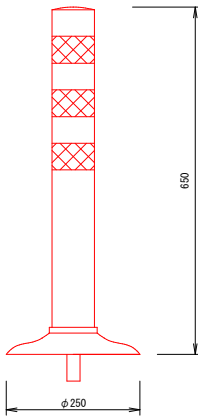
車線分離標 S=1:10
