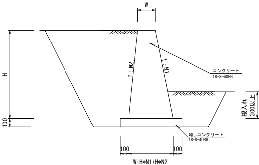
重力式擁壁工 (mあたり)
