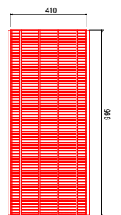
コンクリート蓋、グレーチング蓋 S=1:20 落ちふた式U型側溝3種ふた300 ノンスリップかきあげ、T-25、細目ゴム付
