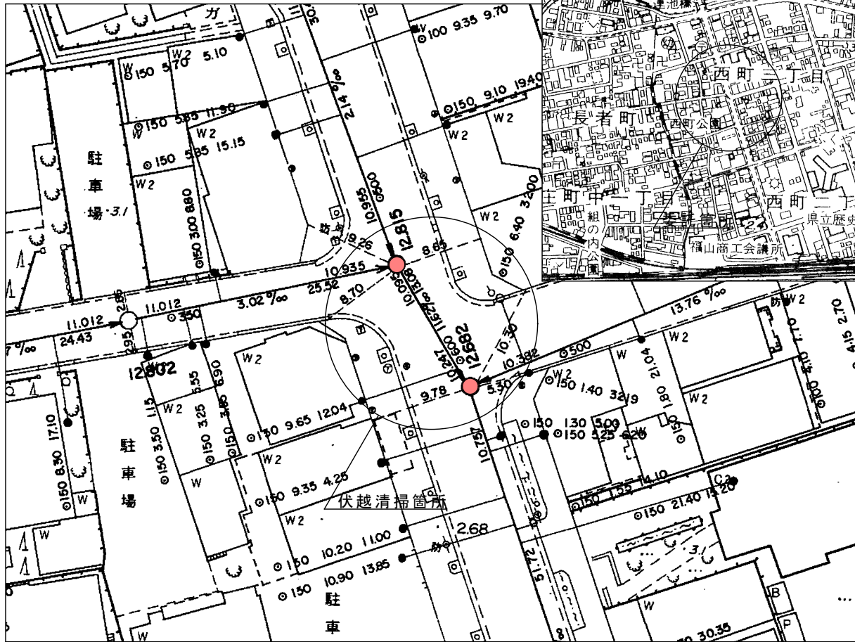
平面図 S=1:500
