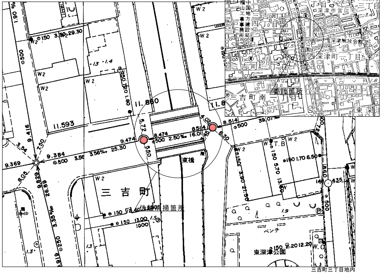
平面図 S=1:500
