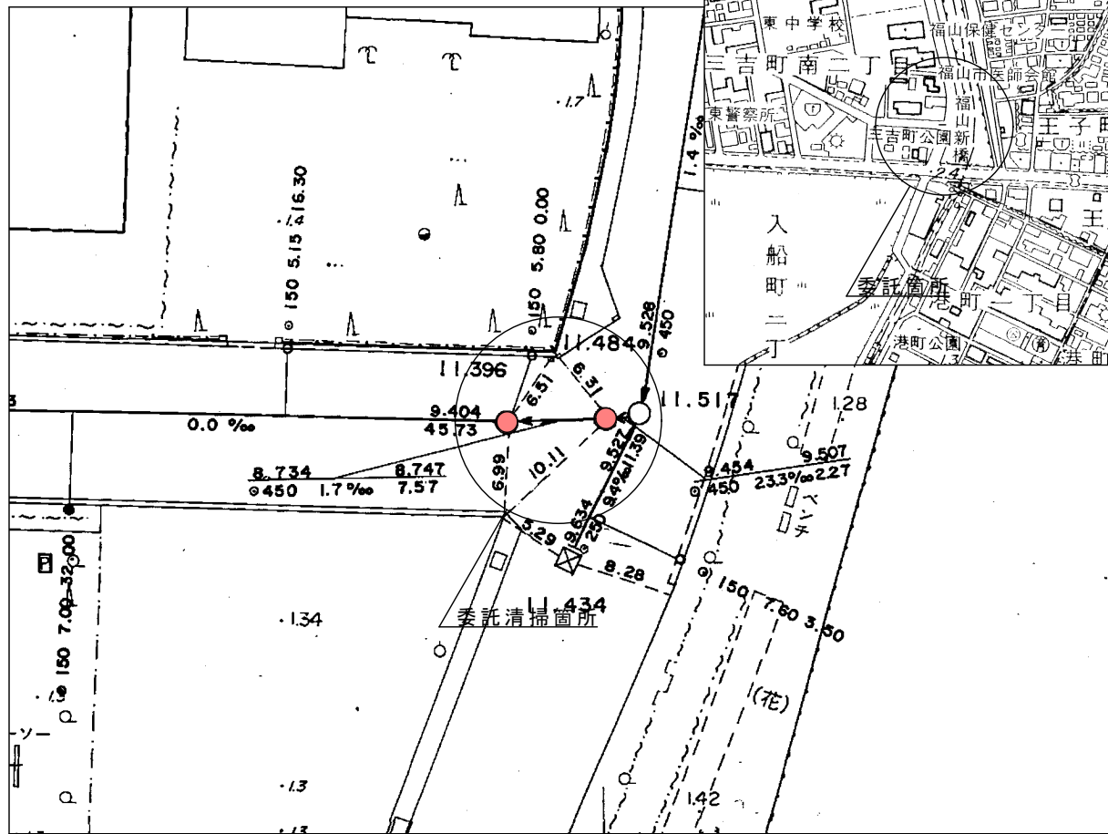
平面図 S=1:500
