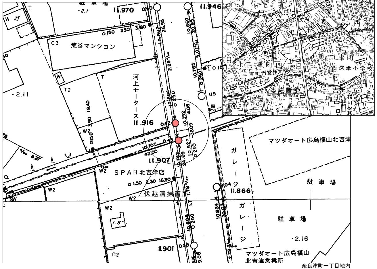
平面図 S=1:500
