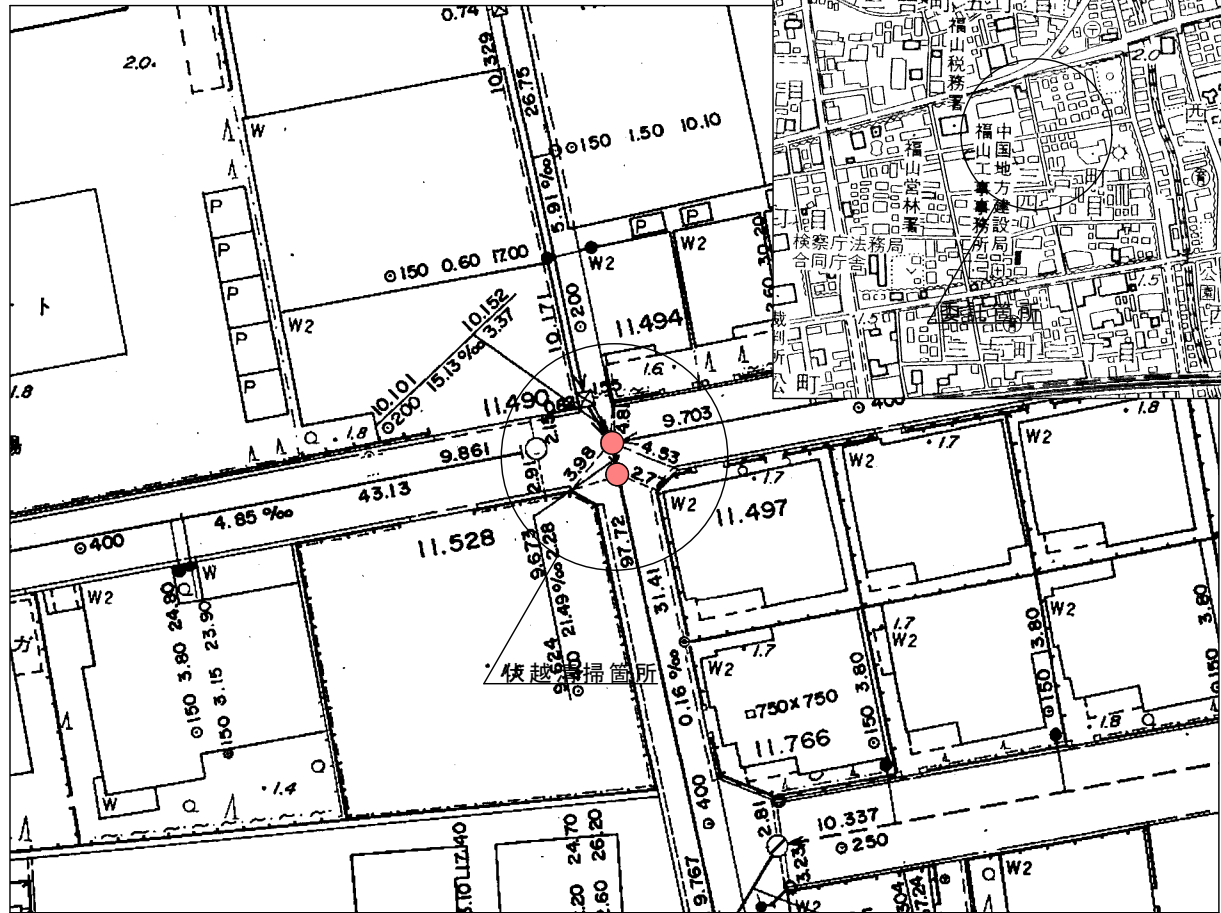
平面図 S=1:500
