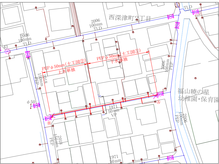
平面図 S=1/500
