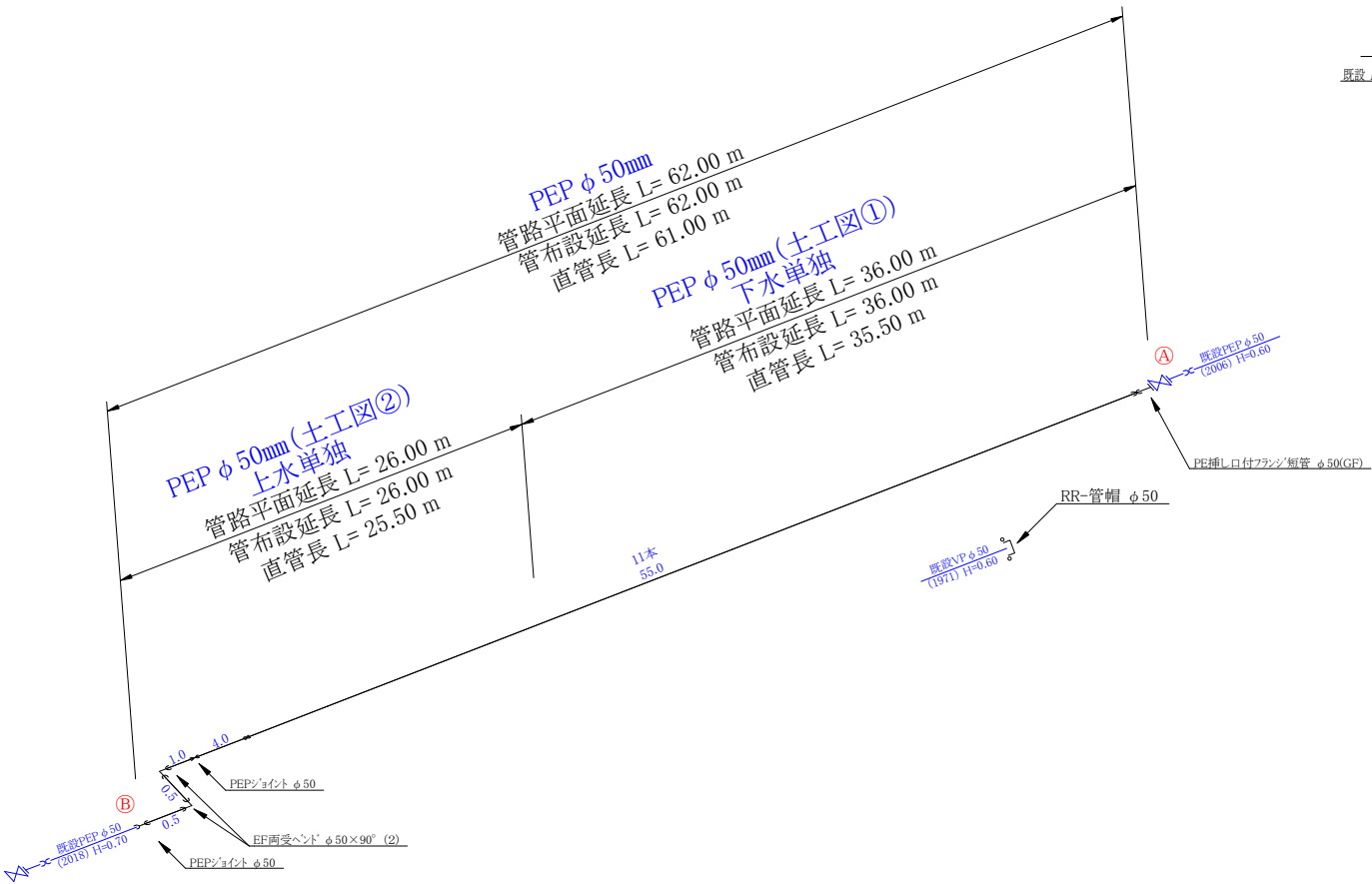
配管系統詳細図 S=NON
