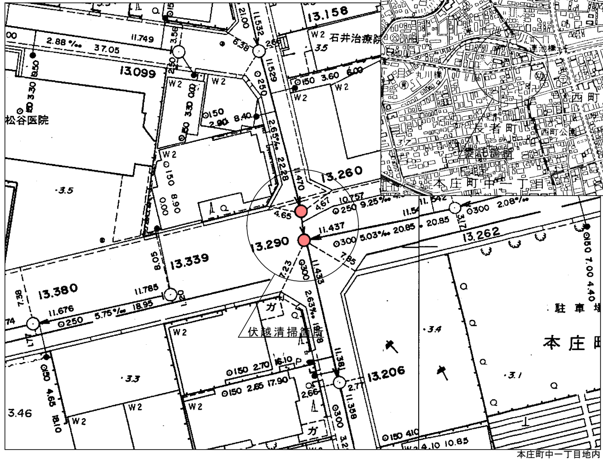
平面図 S=1:500
