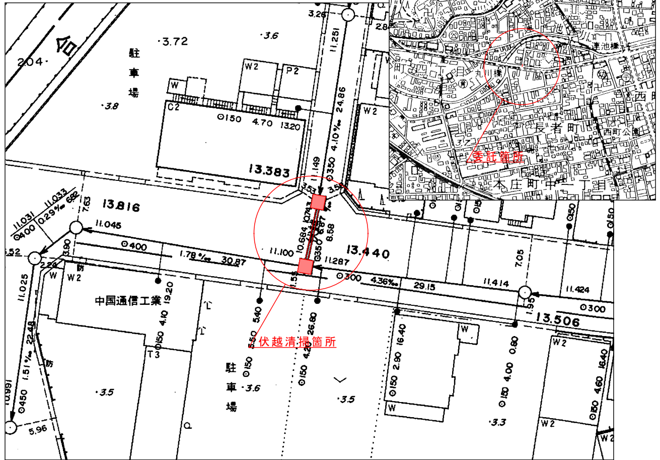
平面図 S=1:500
