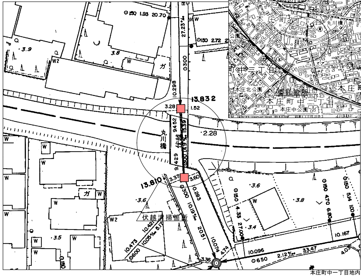
平面図 S=1:500
