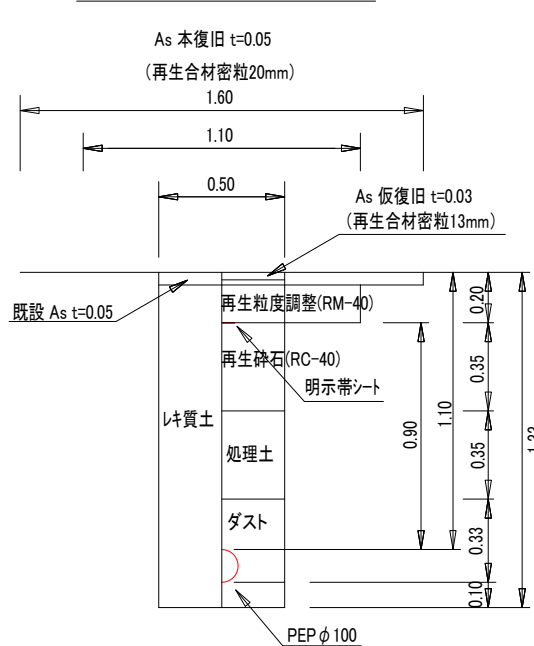
土工① PEPφ100土工図
