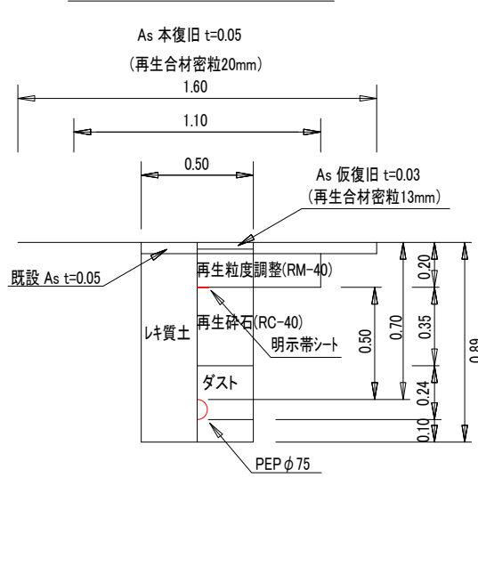
土工⑫ 消火栓土工図
