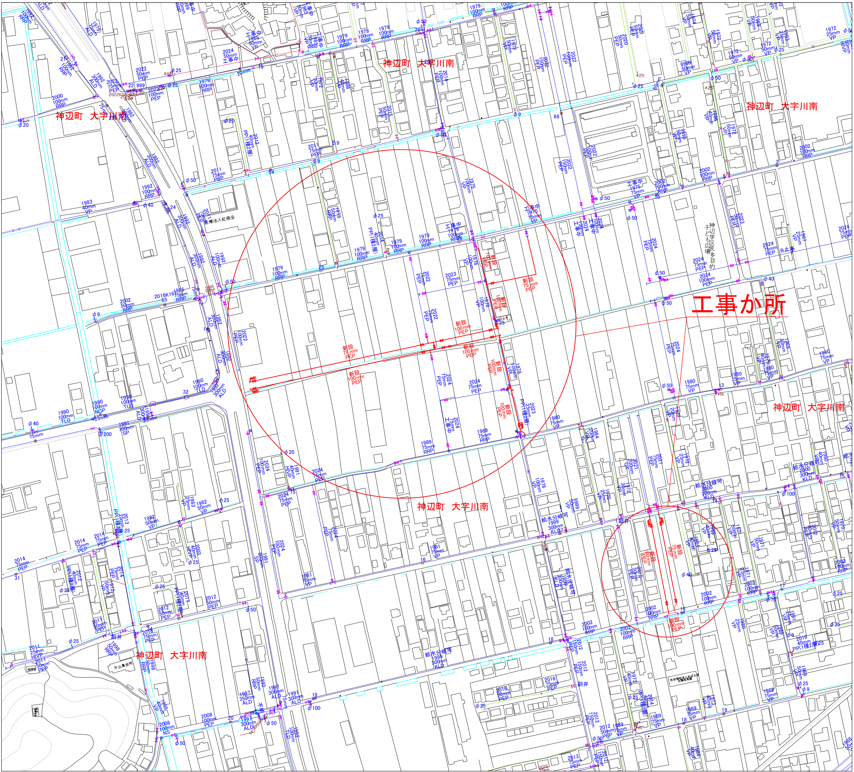
配管図 S=1:2500
