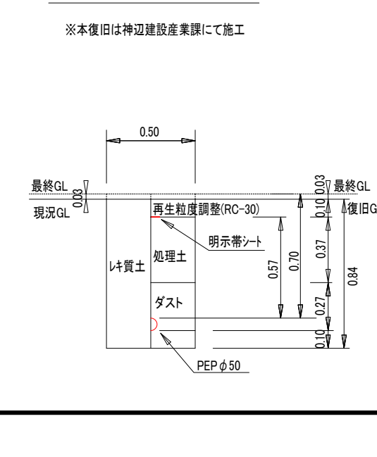
土工⑪ ドレンφ50土工図
