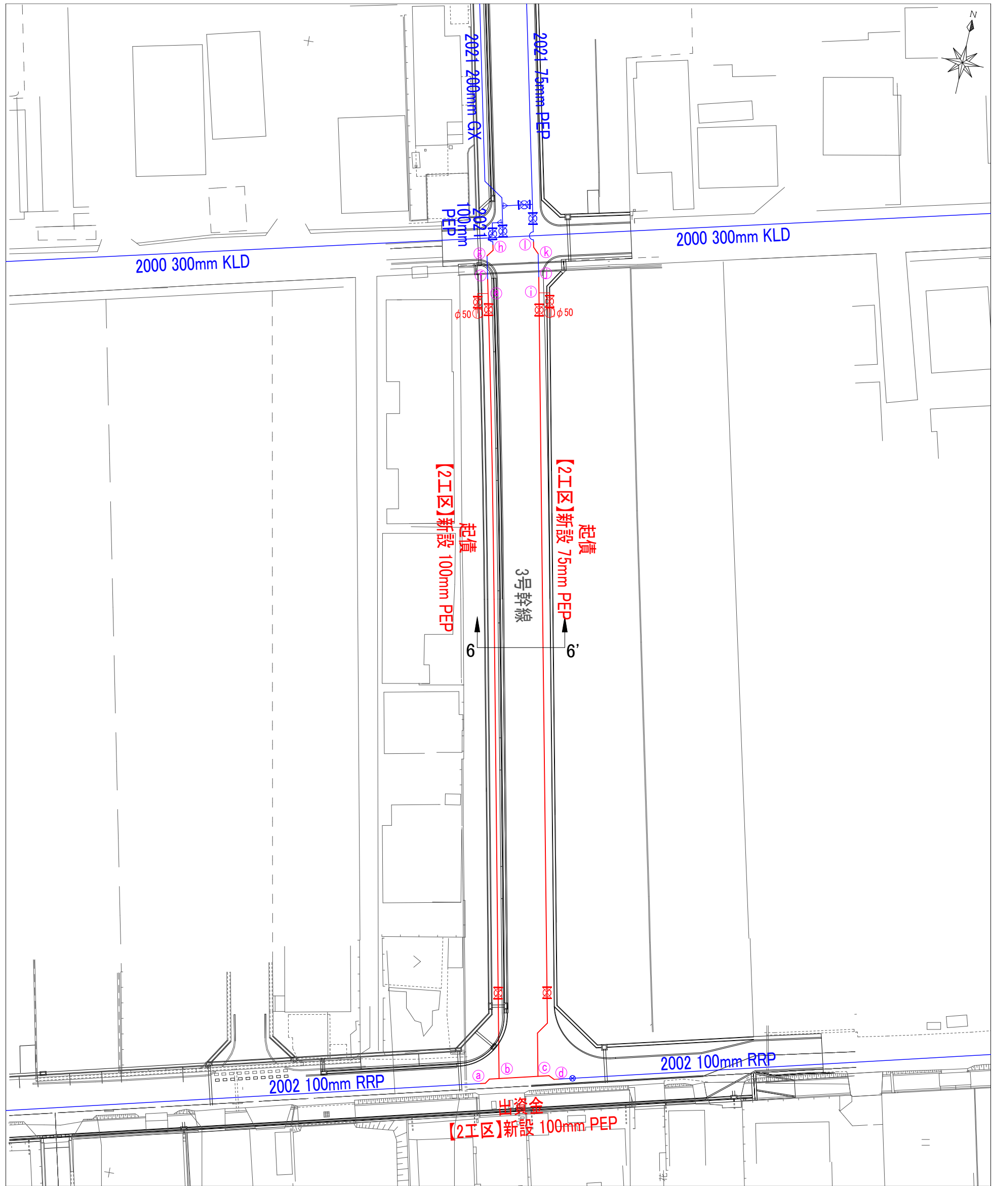
土工① PEPφ100土工図
