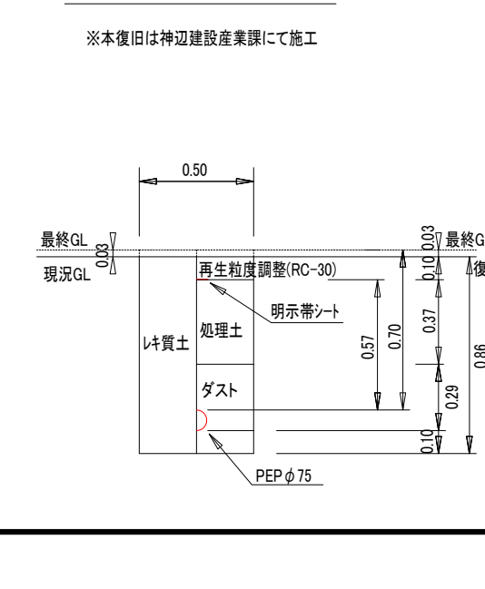
土工⑧ PEPφ75土工図
