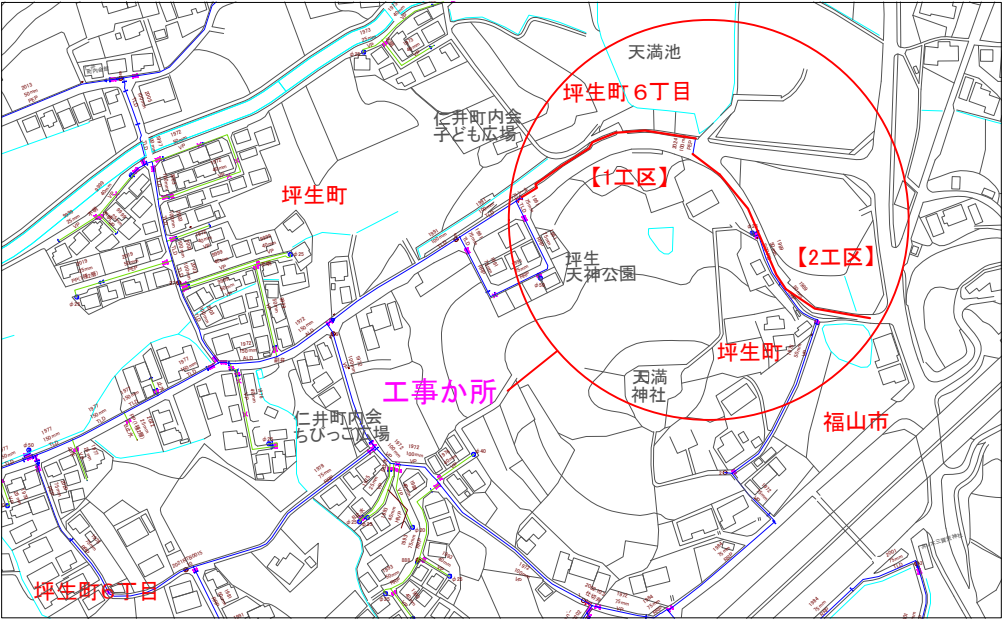
配管図 S=1/2500
