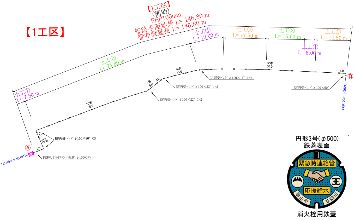
配管系統詳細図【1・2工区】 S=Non
