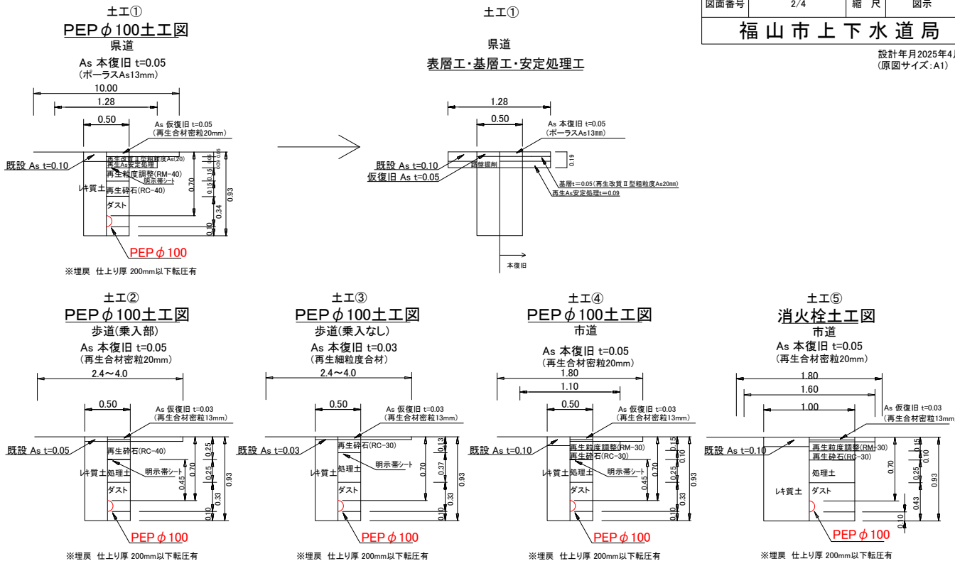
横断面図【1・2工区】 S=1/100
