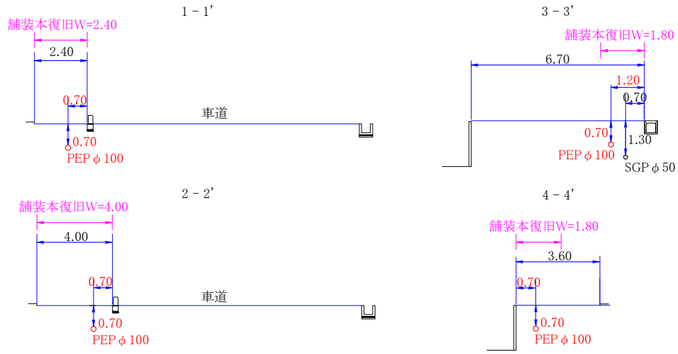
横断面図【1・2工区】 S=1/100
