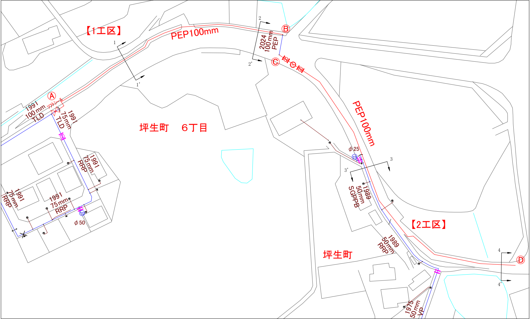
配管系統詳細図【1・2工区】 S=Non
