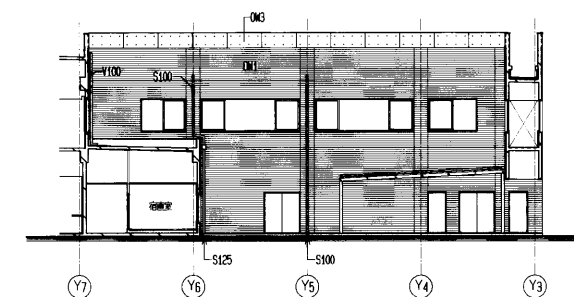
南面 立面図 (ライトコート)
