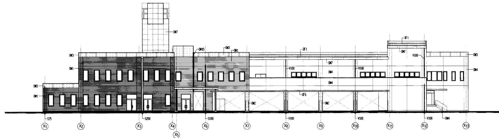
東面 立面図
