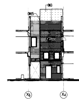
西面 立面図 (ライトコート)
