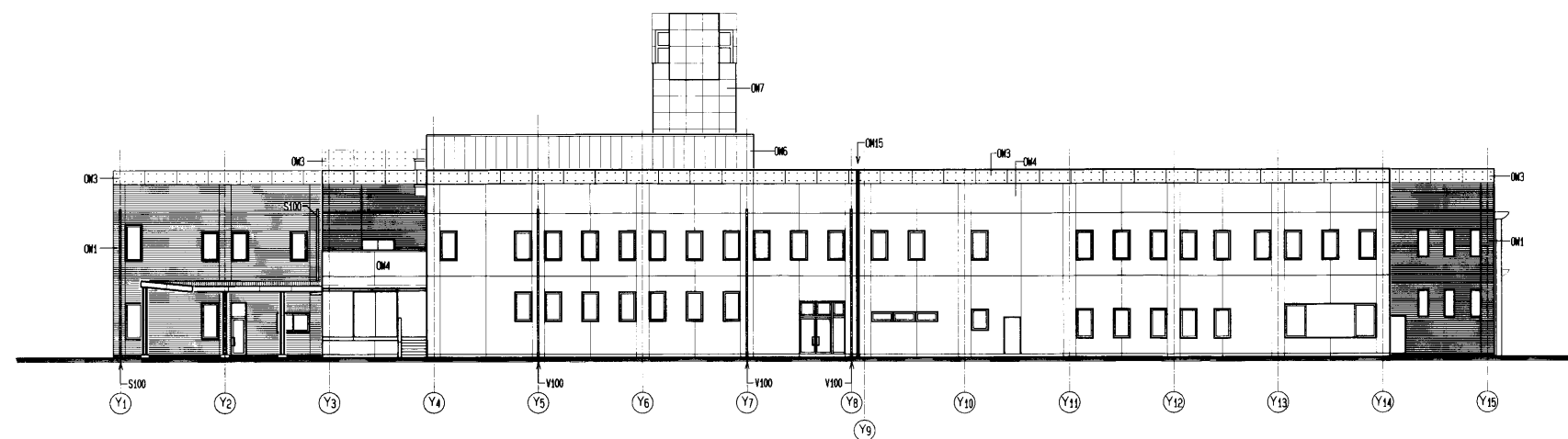
北面 立面図 S=1/200
