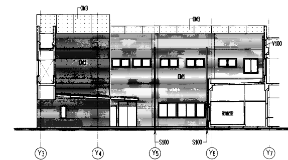
北面 立面図 (ライトコート)
