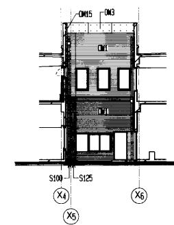
東面 立面図 (ライトコート)
