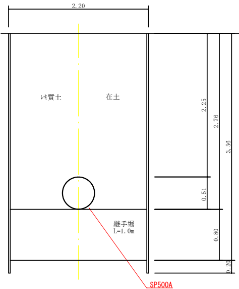
導水管SP500A撤去土工図
