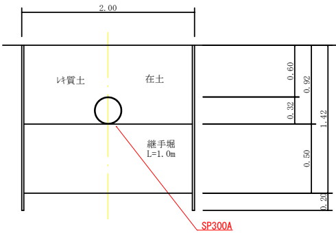
電線管①SP300A撤去土工図
