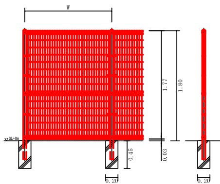
フェンス撤去再設置標準図
