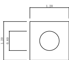
⑤電気マンホール詳細図
