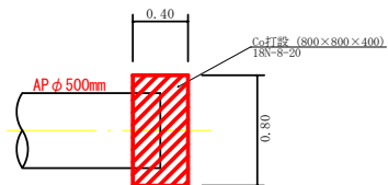
Co舗装部詳細図 S=1/30
