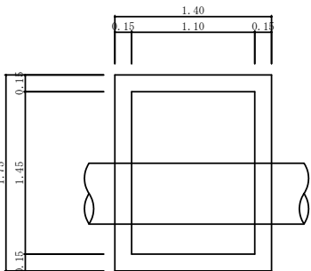
③流量計室詳細図
