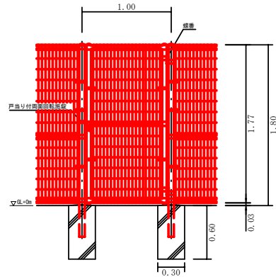
フェンス片開門扉撤去再設置標準図
