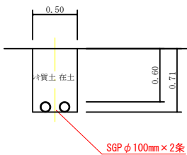
電線管④撤去土工図
