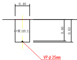
給水管VP \phi 25mm撤去土工図
