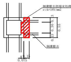
側溝撤去部端末処理図 S=1/30
