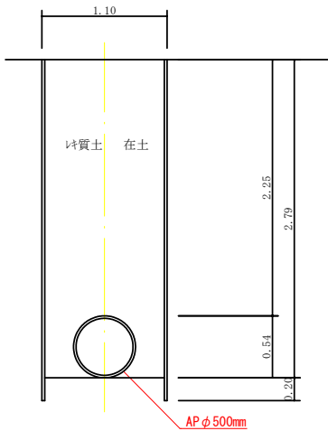
導水管AP \phi 500mm撤去土工図
