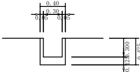
撤去側溝標準図(蓋無) S=1/30
