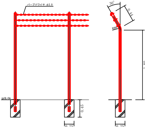
忍び返し部撤去標準図
