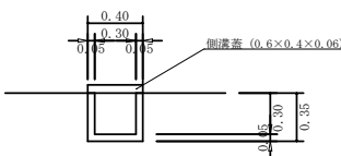
撤去側溝標準図(蓋有) S=1/30
