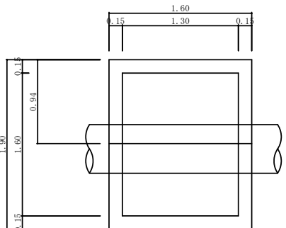
④弁室詳細図
