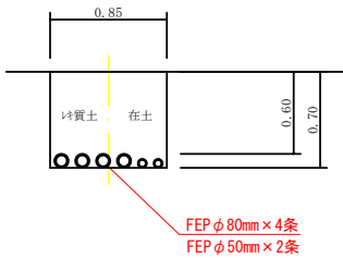
電線管④撤去土工図
