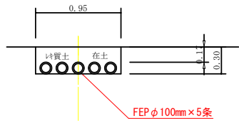
電線管③撤去土工図
