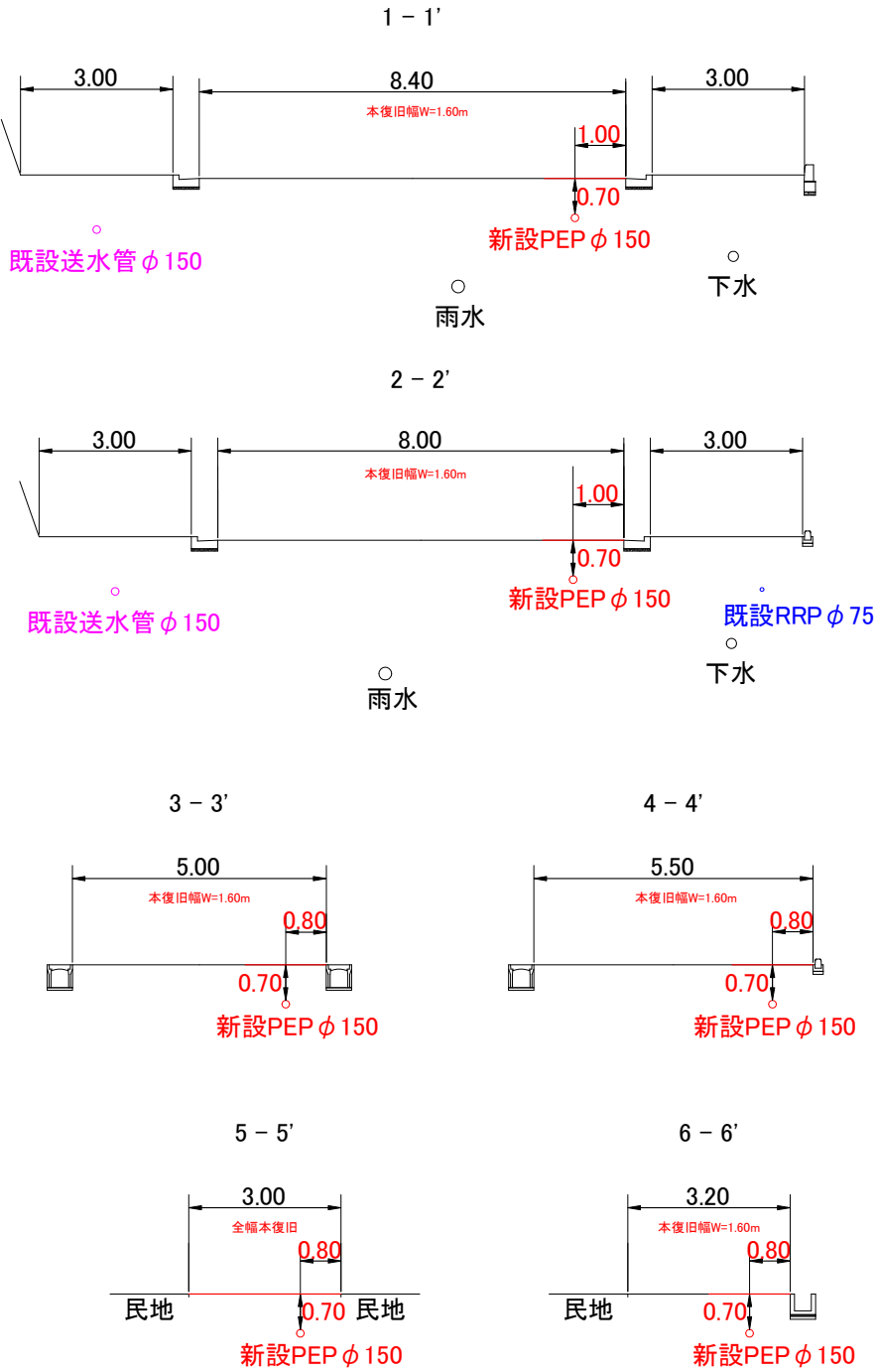
【横断面図】 S=1/75
