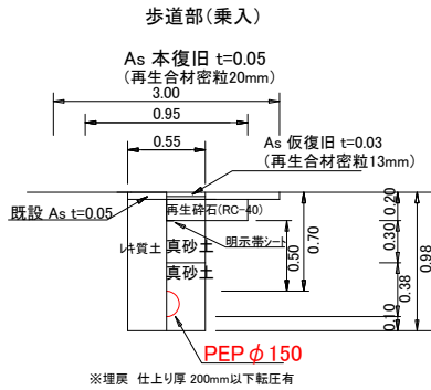
PEPφ150土工図 土工①
