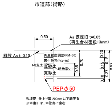
ドレンφ50土工図
