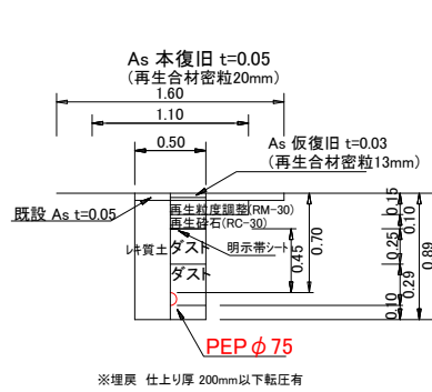
PEPφ75土工図 土工⑥
