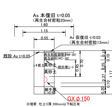
消火栓土工図
