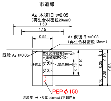
消火栓土工図
