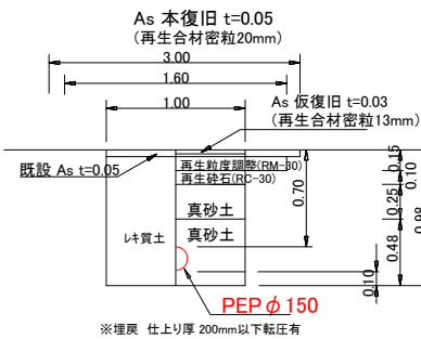
消火栓土工図
