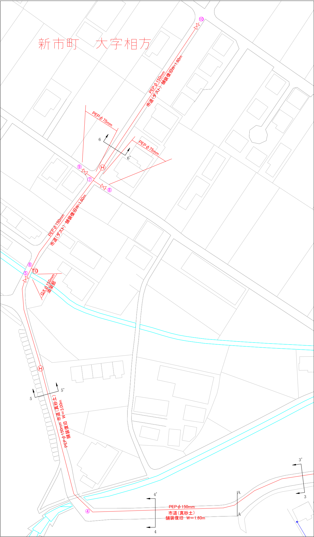
【平面図】 S=1/500
