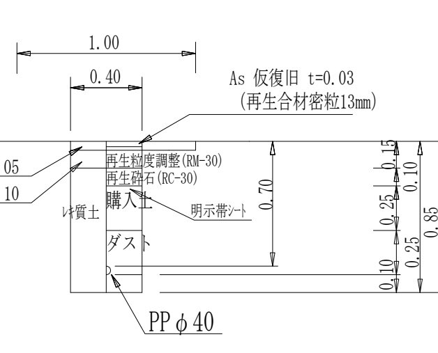
給水管 φ40土工図 (チズ分岐)
