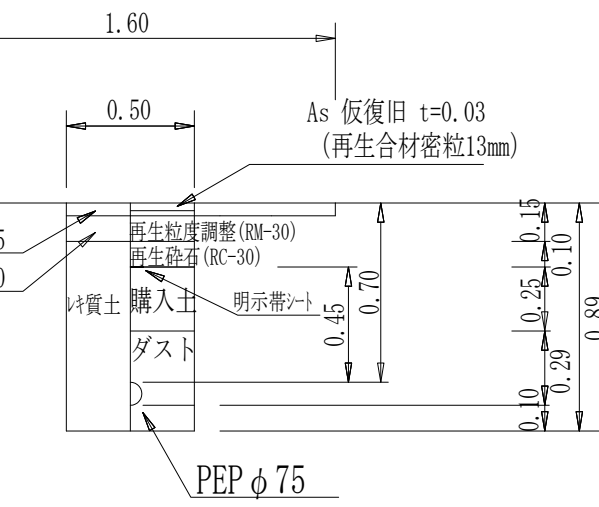
PEP φ75土工図②
