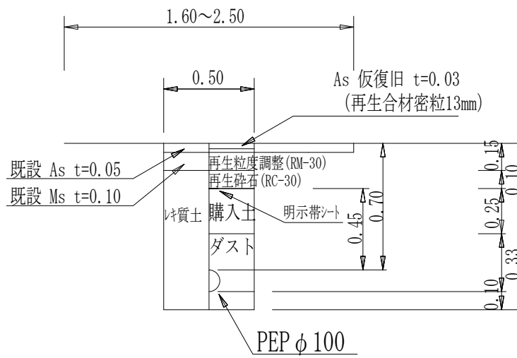
PEP φ100土工図①
