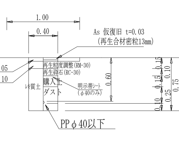
給水管 φ40以下土工図 (サドル分岐)
