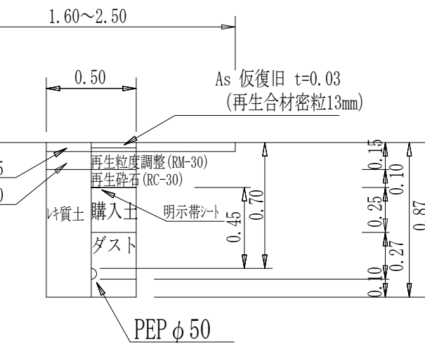
PEP φ50土工図③ (給水 φ50)
