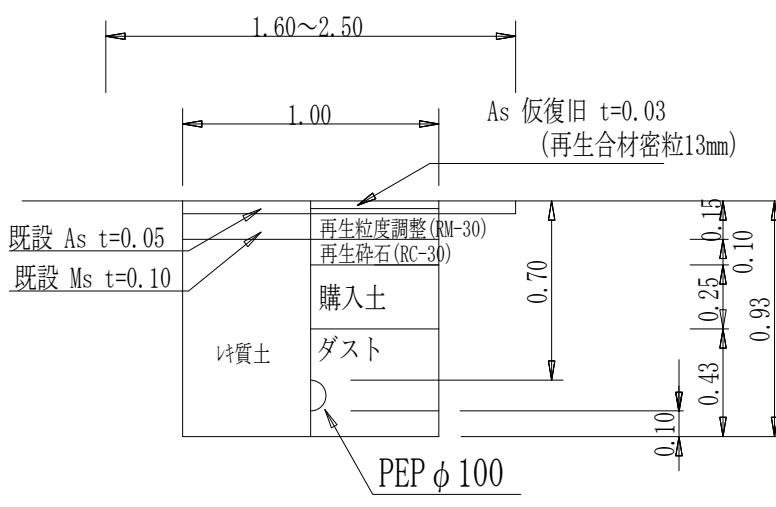
消火栓土工図④
