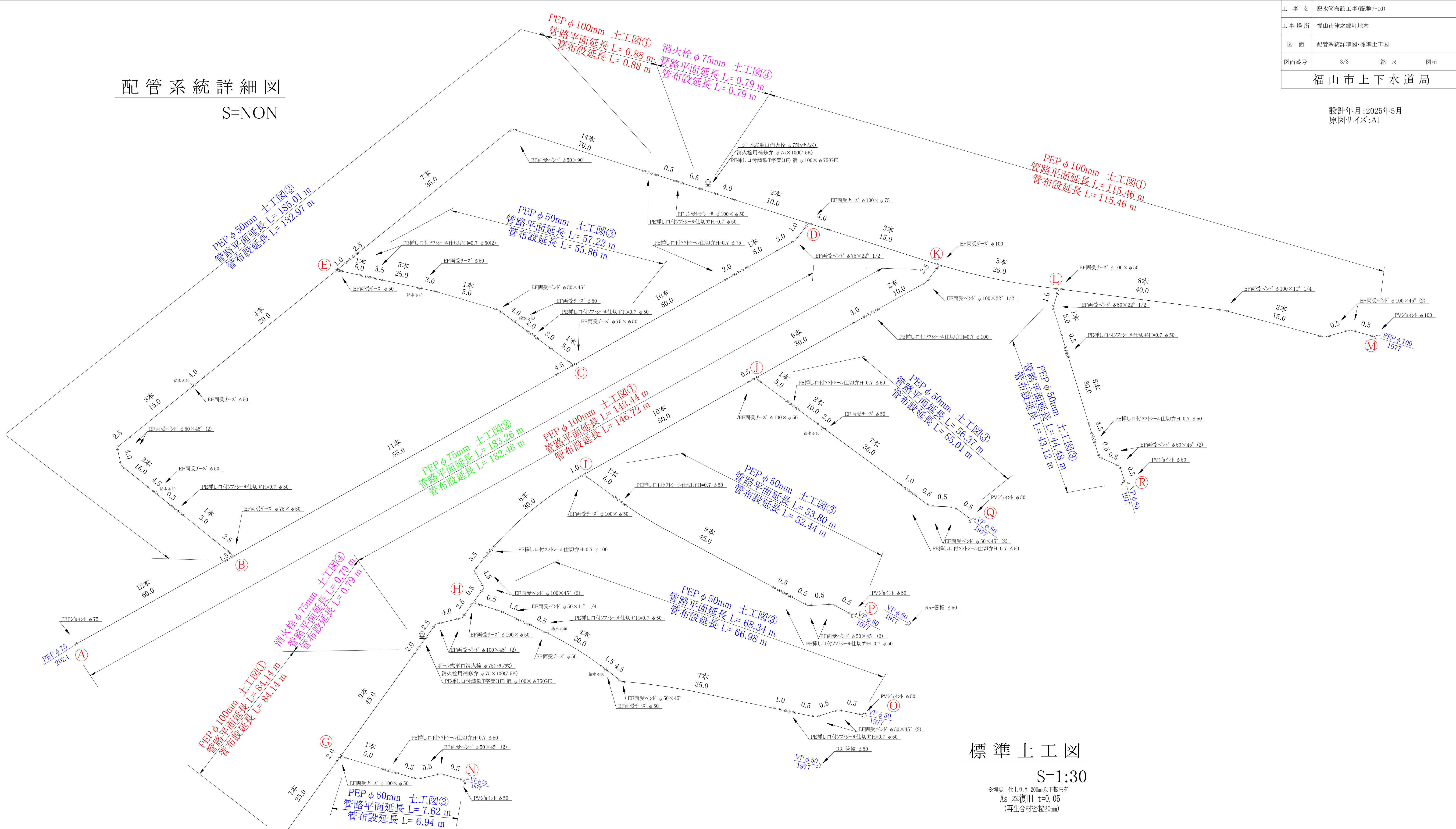
PEP φ100土工図①
