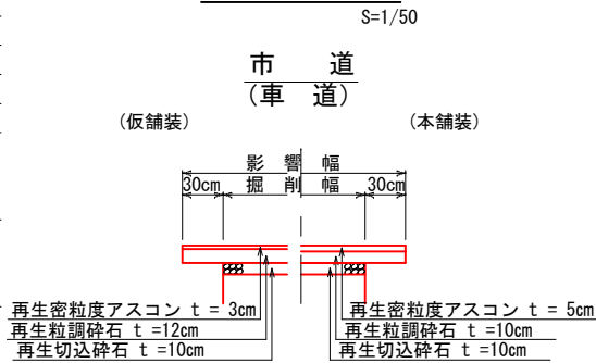
舗装断面図
