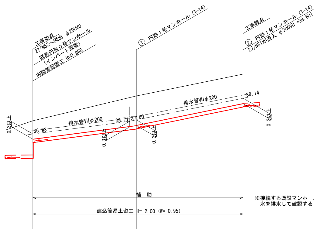
管渠埋設縦断面図 S=縦1/100 横1/500
