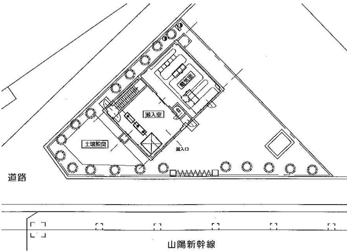
施設平面図
