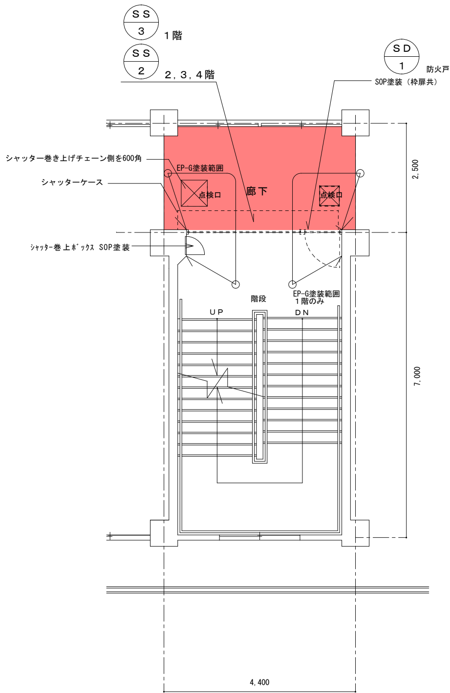
北棟 西側 平面詳細図 S=1/60
