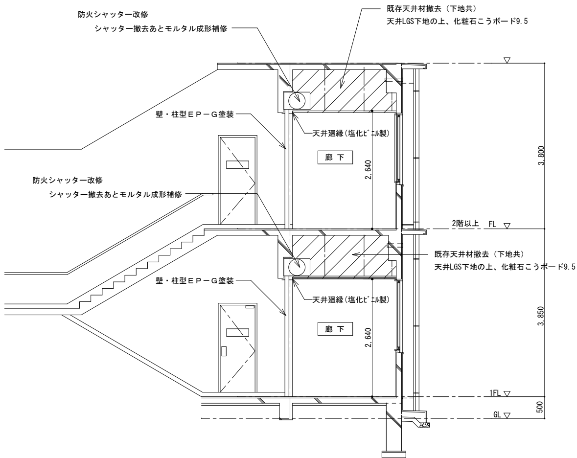
断面詳細図 S=1/60
