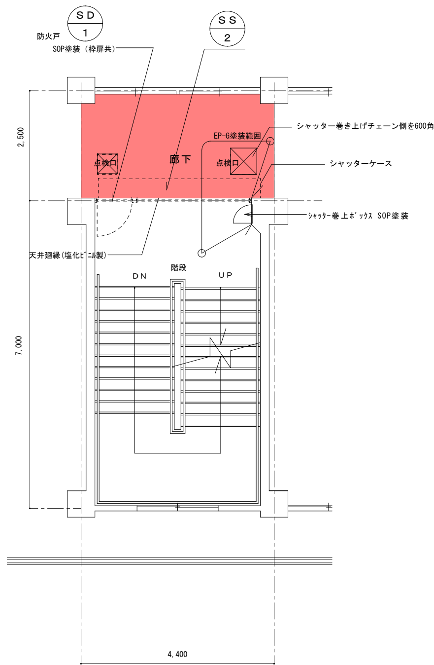
南棟 西側 平面詳細図 S=1/60
