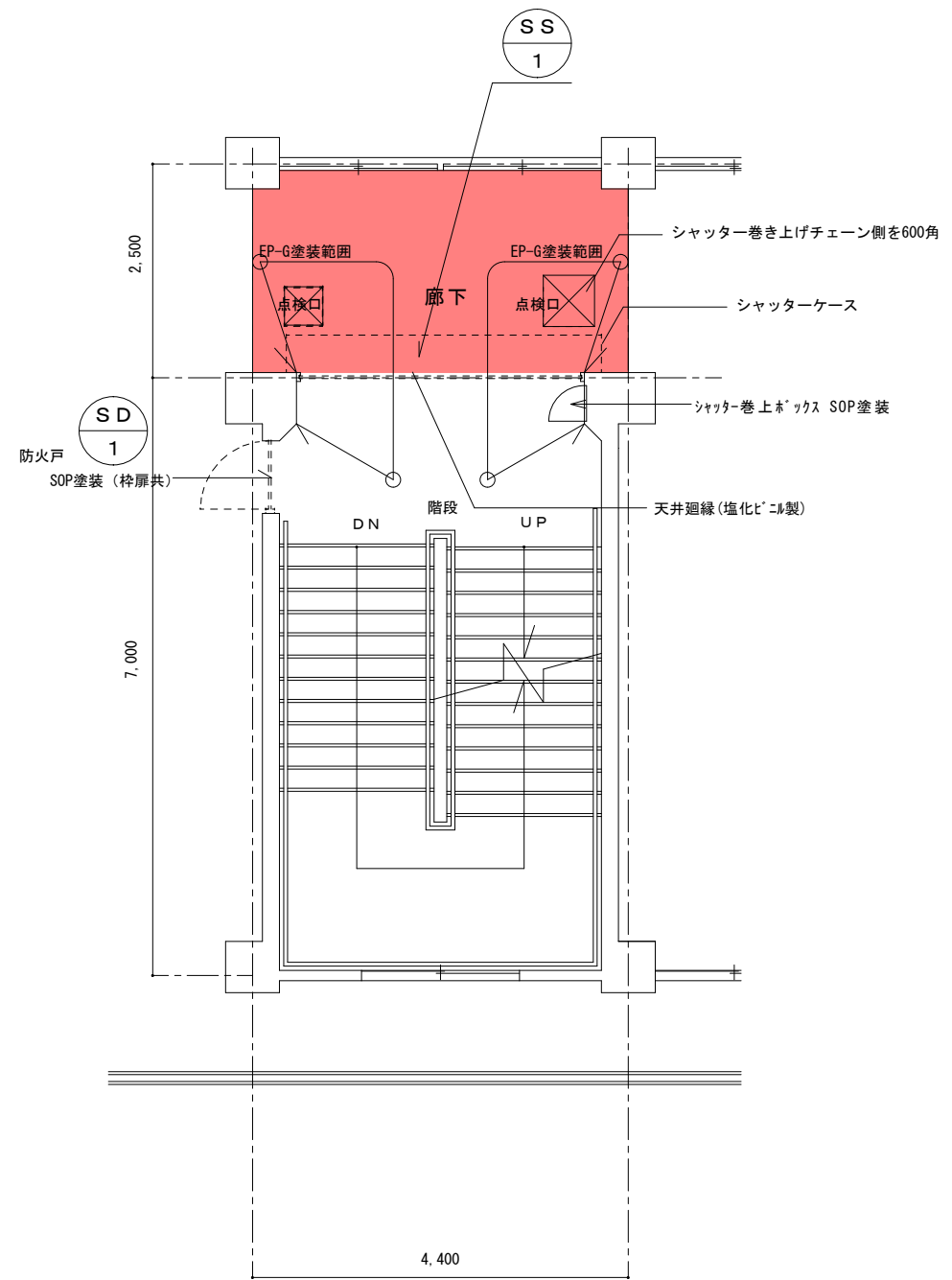
南棟 東側 平面詳細図 S=1/60
