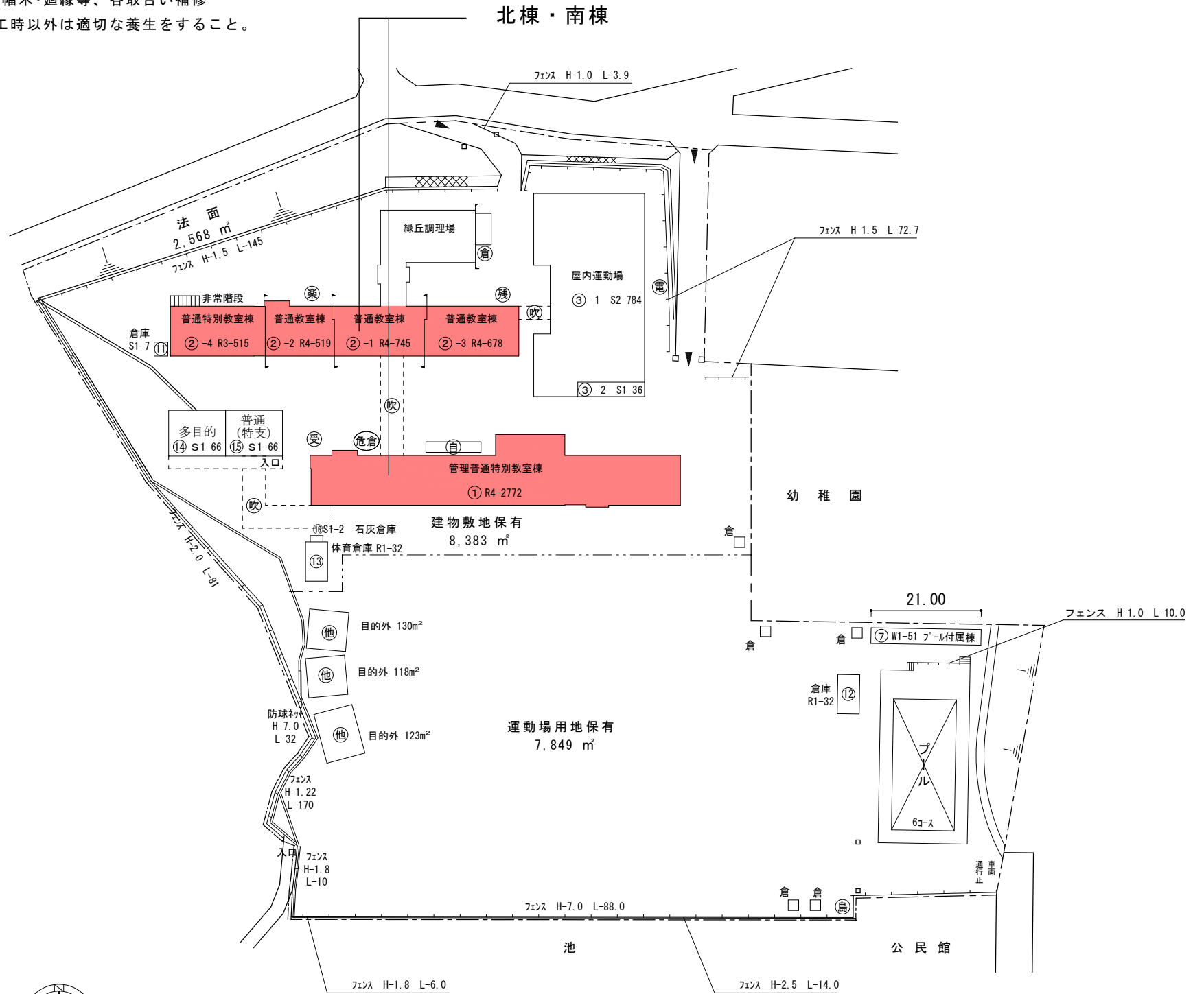
配置図 S=1/800
