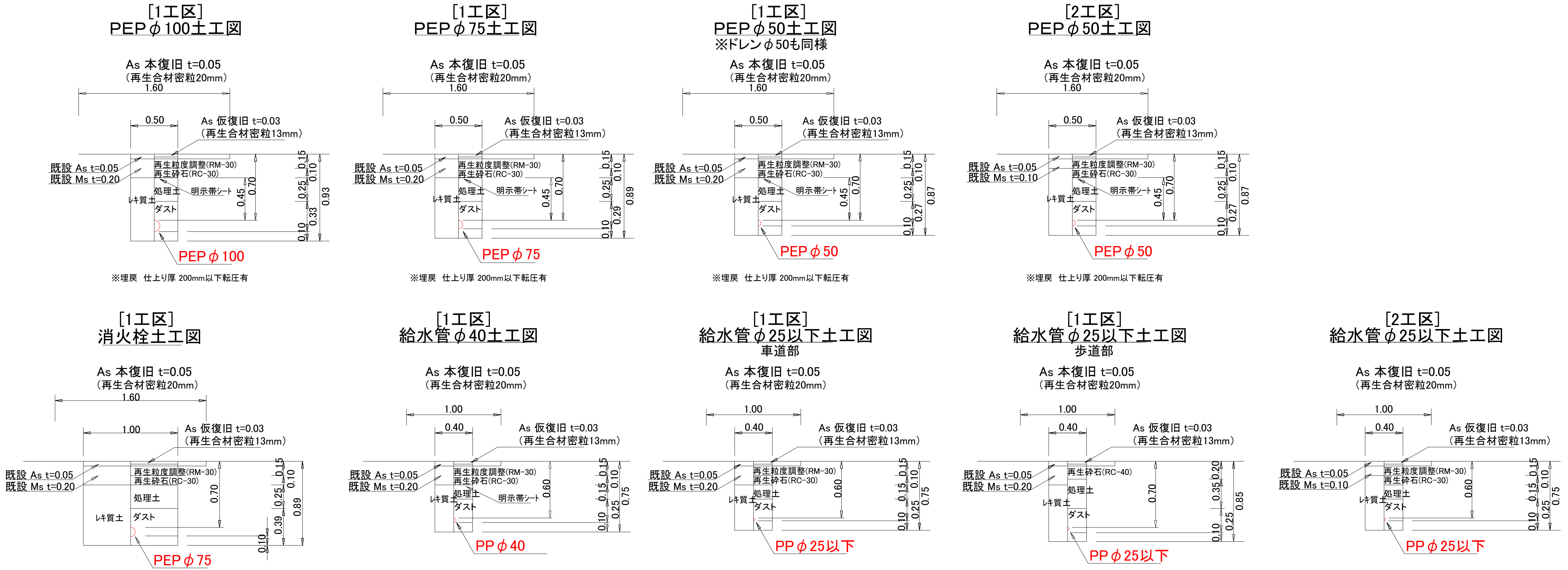
土工図 S=1:30
