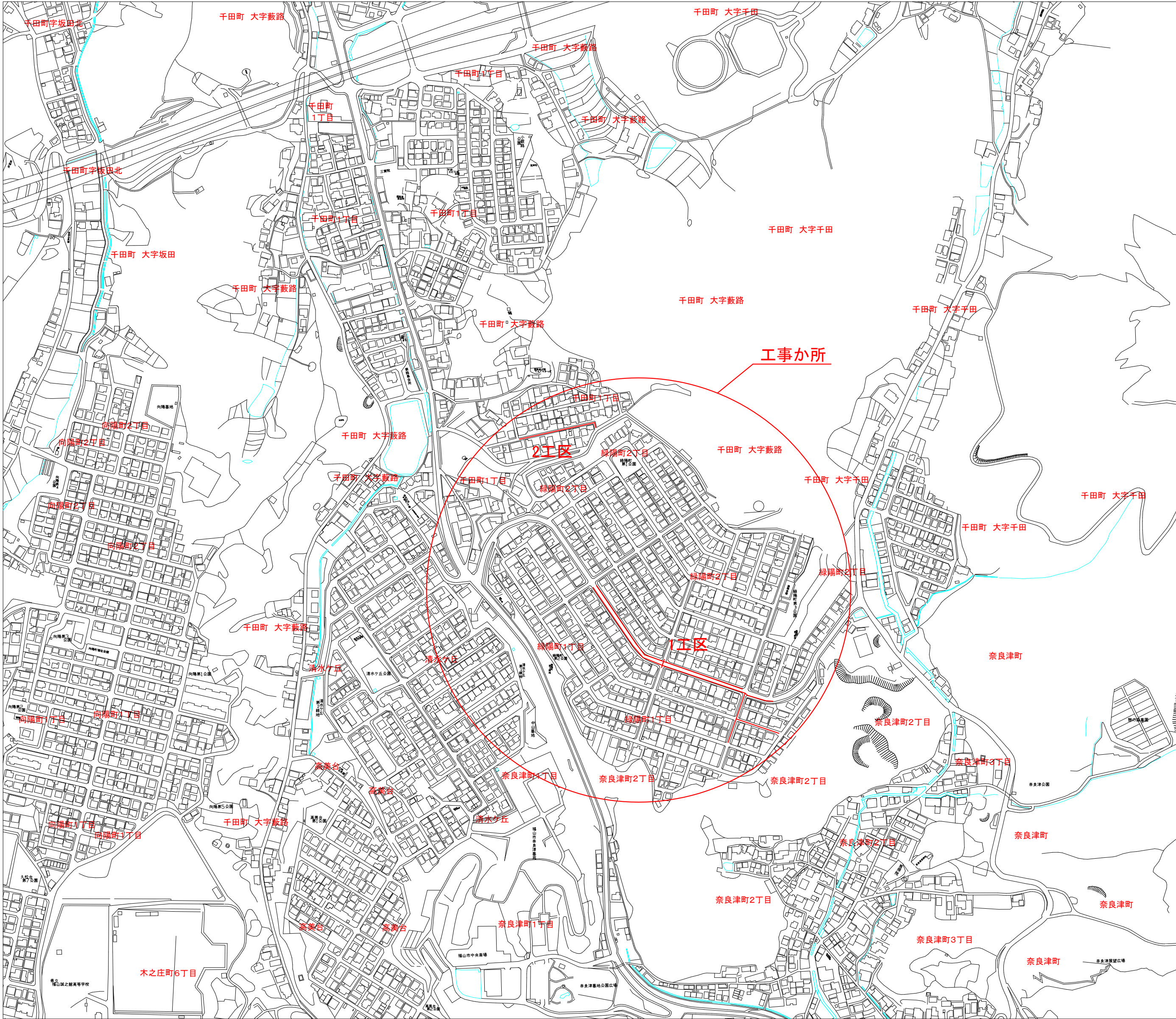
位置図 S=1:5000
