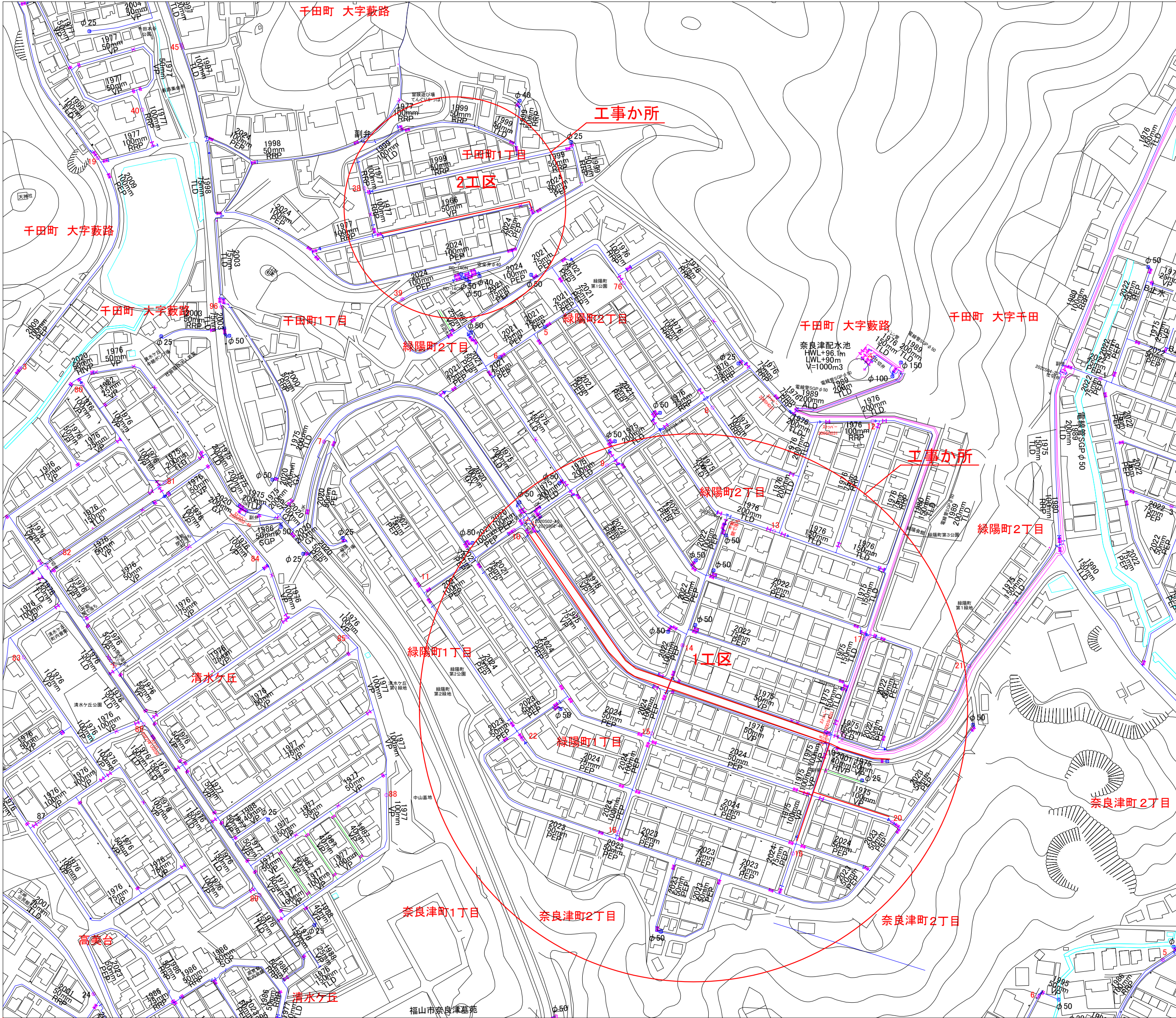
配管図 S=1:2500
