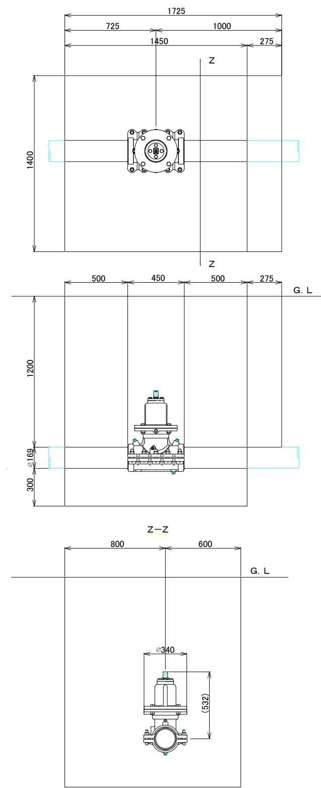
不断水簡易仕切弁土工図 S=1:NON
