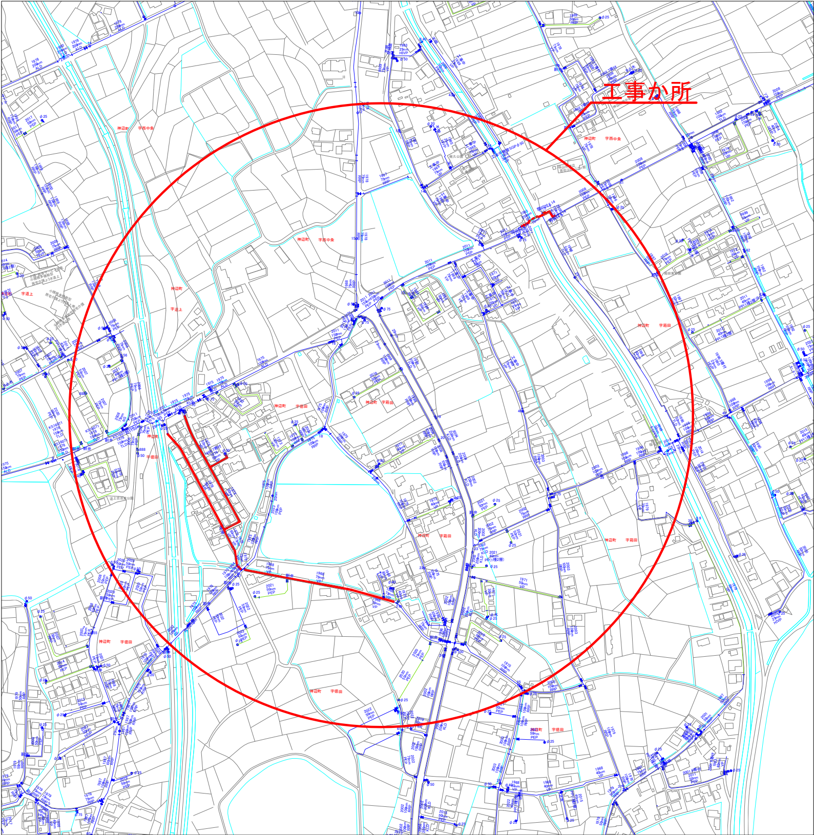
配管図 S=1／2500
