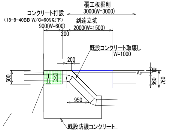
右岸側土工図 S=1／50
