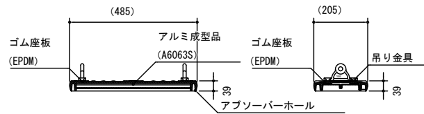
ゴム座板断面図 S= 1 : 20
