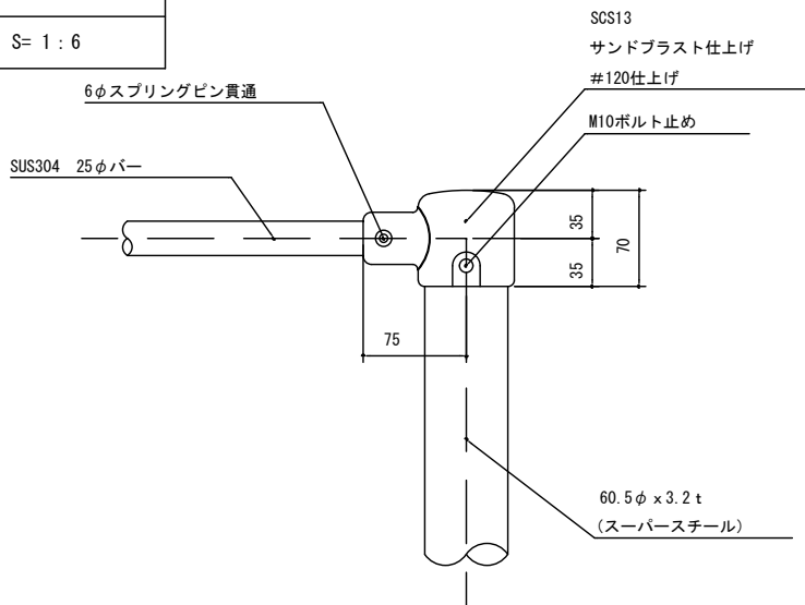
イ部詳細図 S= 1 : 6
