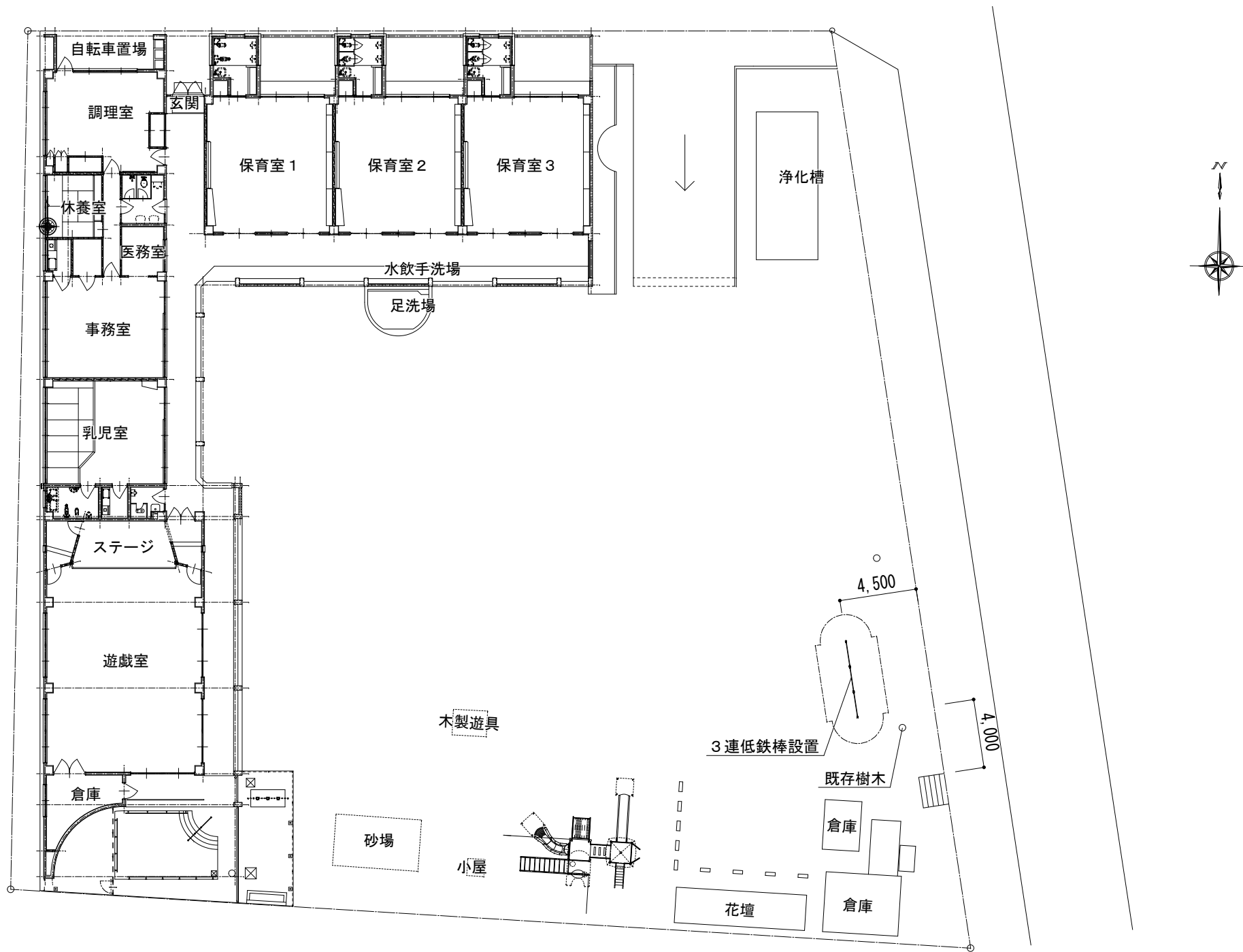
配置図 S = 1 / 3 0 0
