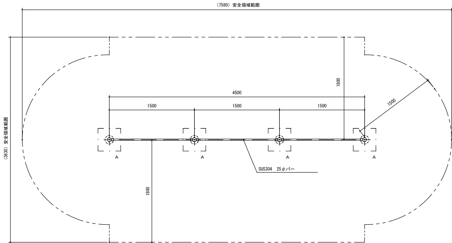
平面図 S= 1 : 40
