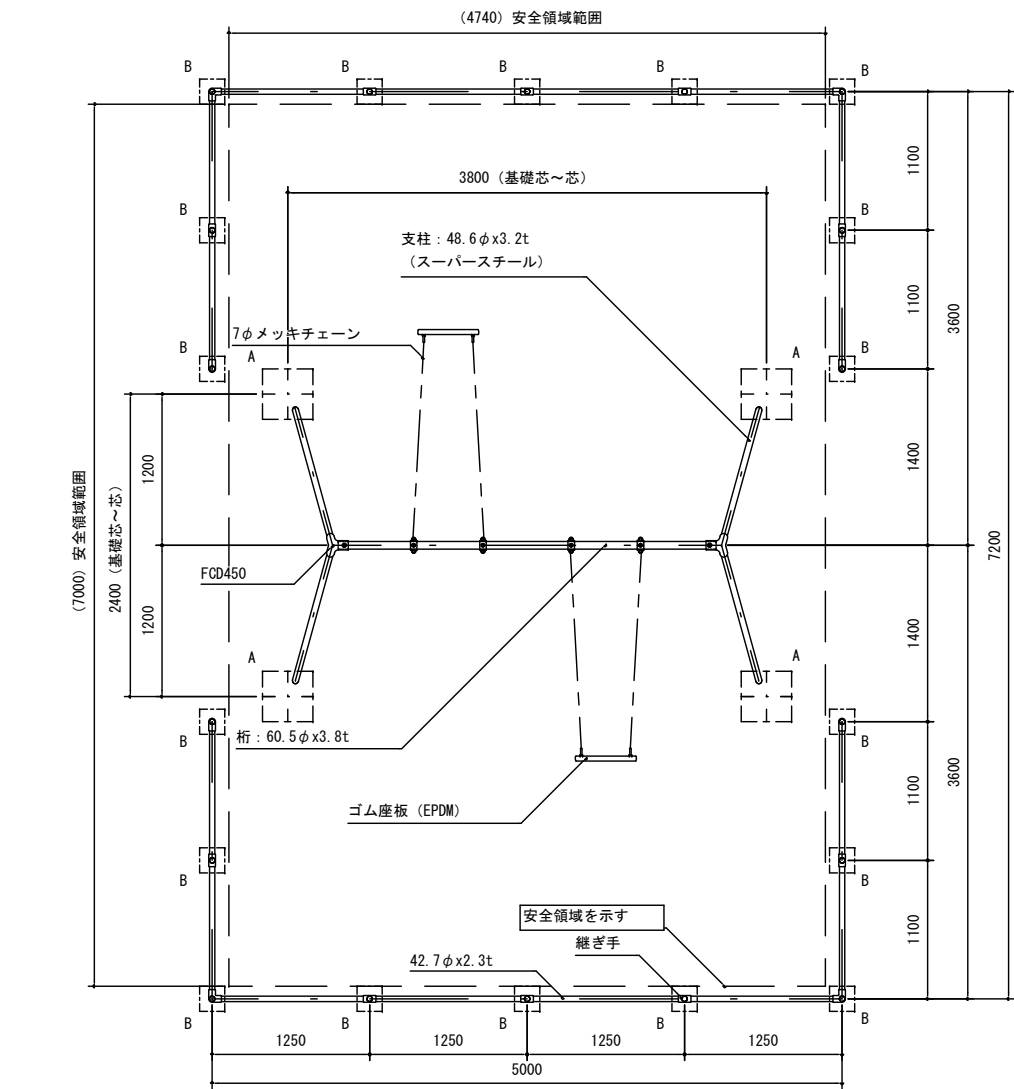
平面図 S= 1 : 60
