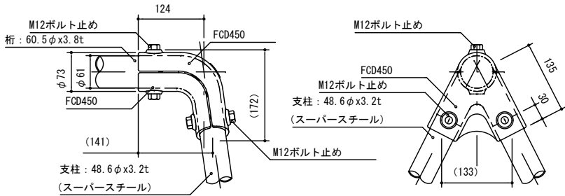
ブランコハンガー詳細図 S= 1 : 10
