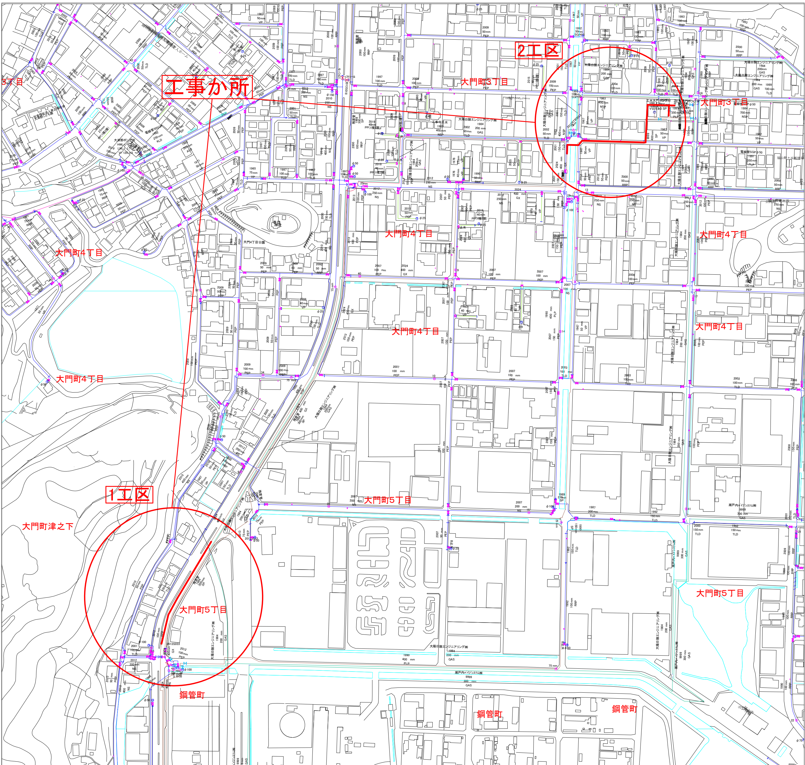
配管図 S=1/2,500
