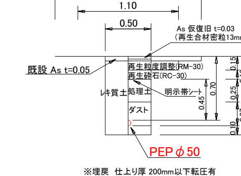
土工⑫ 消火栓土工図
