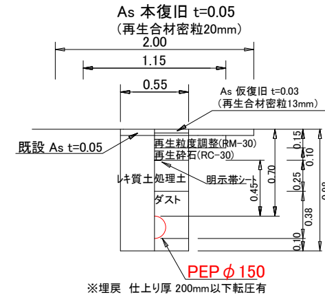
土工② PEPφ150土工図
