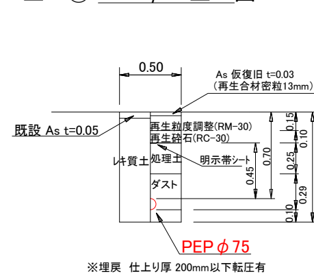
土工⑥ PEP \phi 75 土工 Ⅹ
