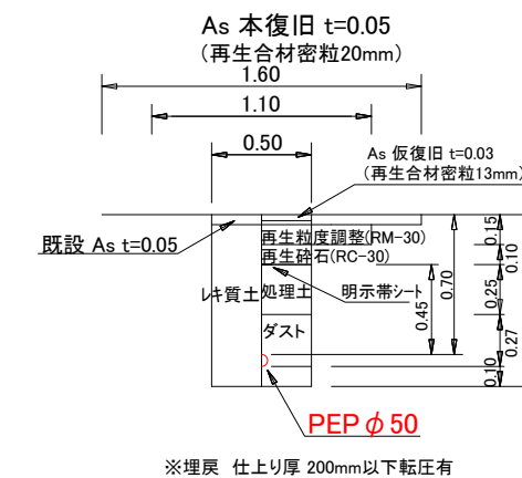
土工⑫ 消火栓土工図
