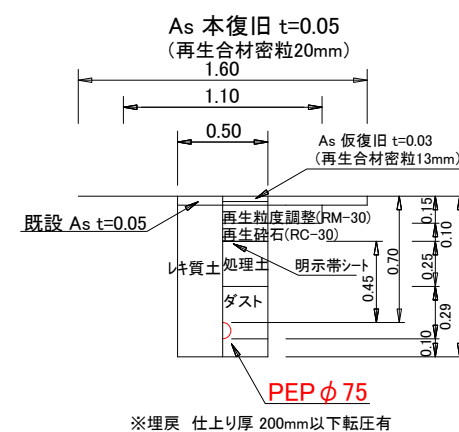
土工⑤ PEP \phi 75 土工 図
