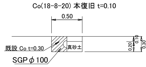
土工⑭ 既設管撤去土工図
