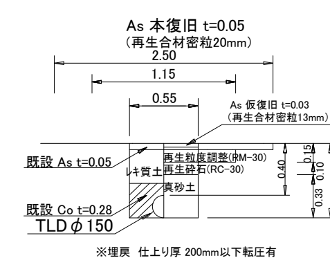
港湾区域 土工⑬既設管撤去土工図
