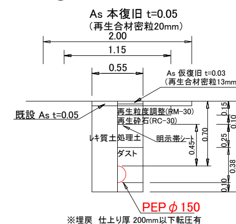
土工② PEP \phi 150 土工 図
