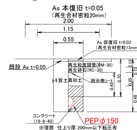
法面部 土下② DEF 土 150 土下 70
