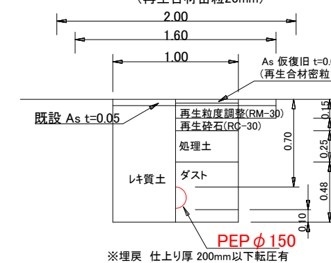
土工⑫ 消火栓土工図
