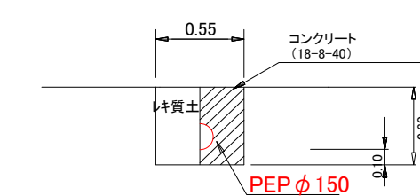
土工③ PEPφ150土工図
