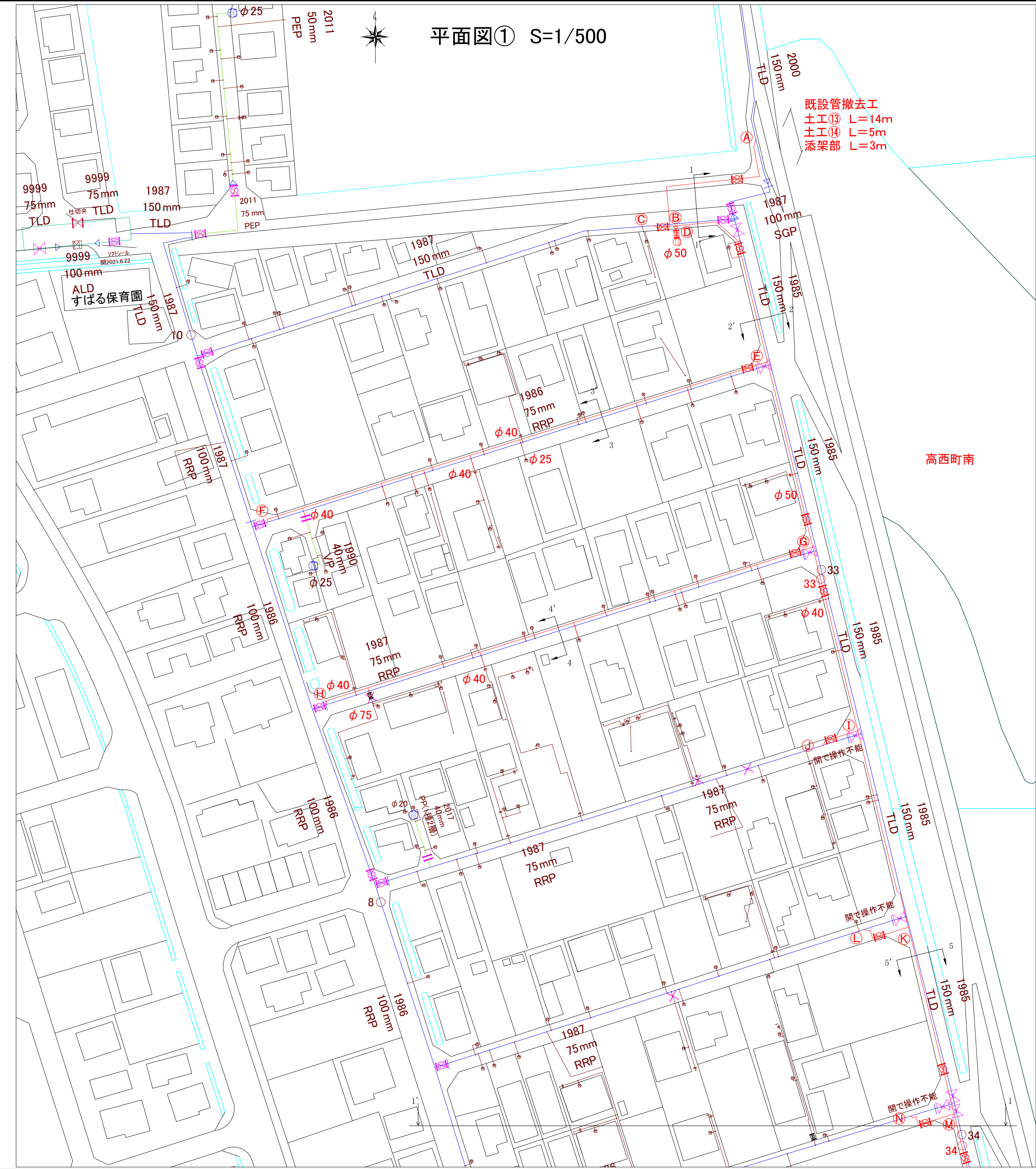
土工① PEPφ150土工図
