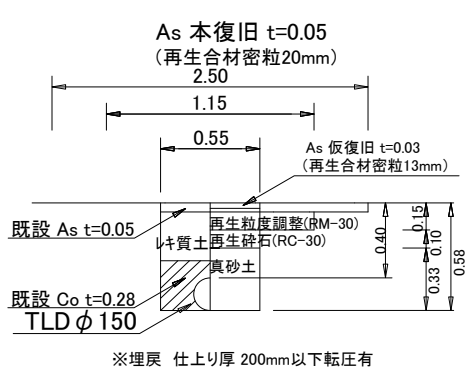
土工⑬ 既設管撤去土工図
