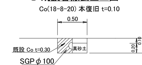
港灣区域(法面部) 土工⑭ 既設管撤去土工Ⅹ
