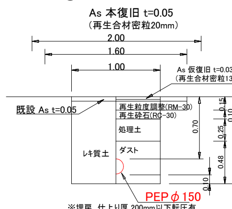
土工⑫ 消火栓土工図
