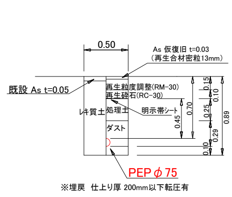
土工⑥ PEPφ75土工図
