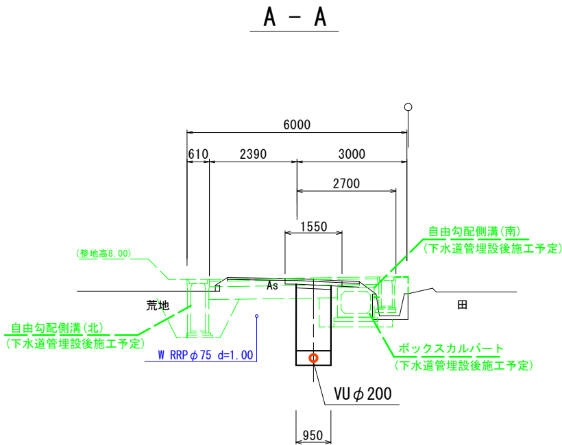
標準横断面図 S=1/100
