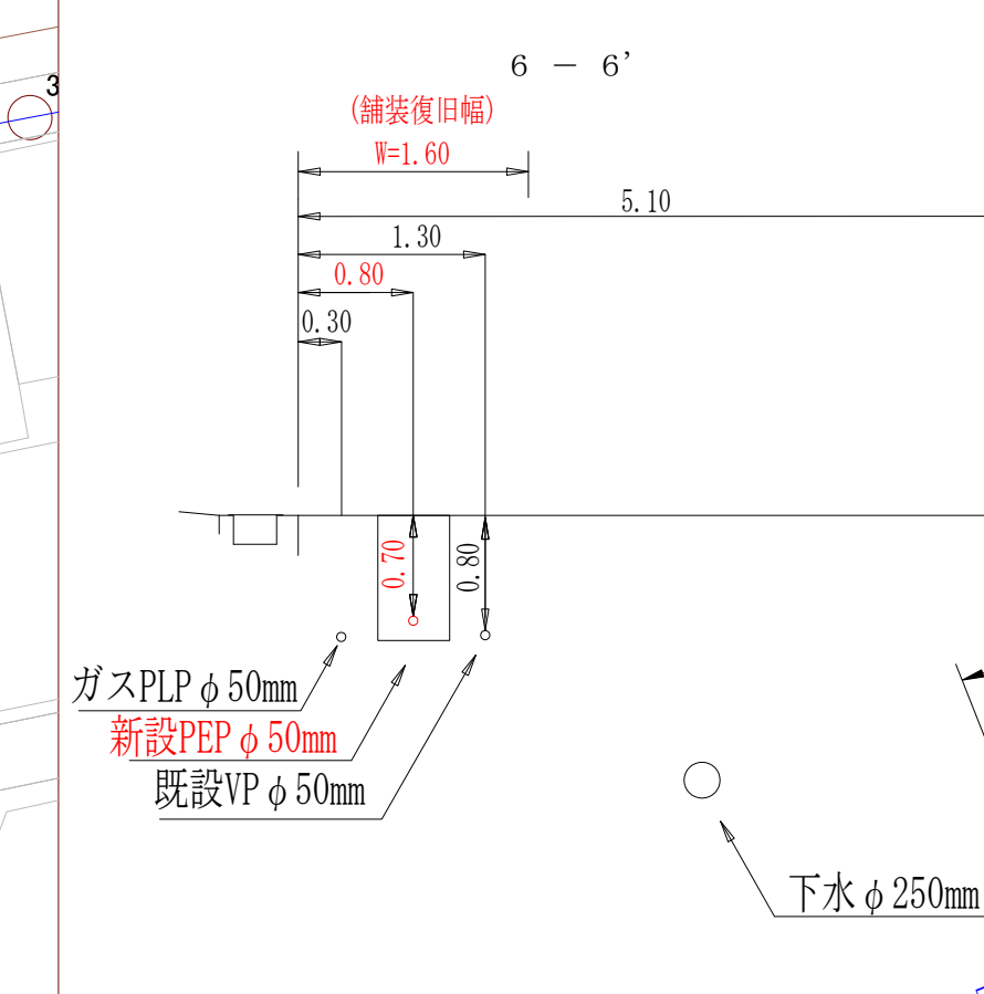
横断面図 S=Non 【5工区】
