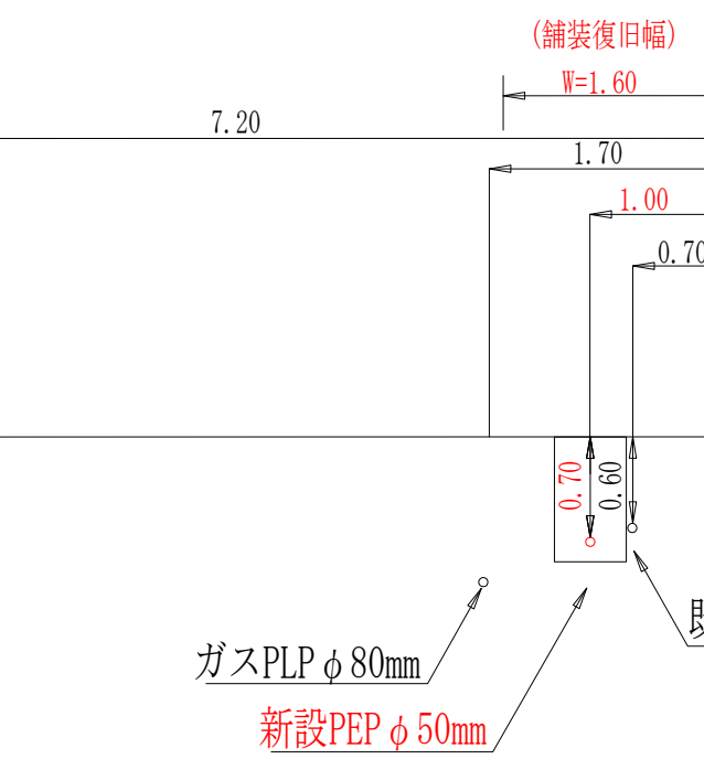
横断面図 S=Non 【7工区】
