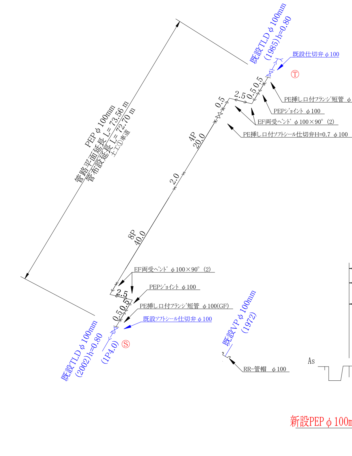
配管系統詳細図 S=Non 【6工区】
