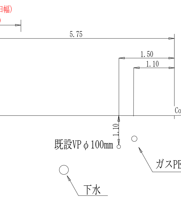
横断面図 S=Non 【6工区】
