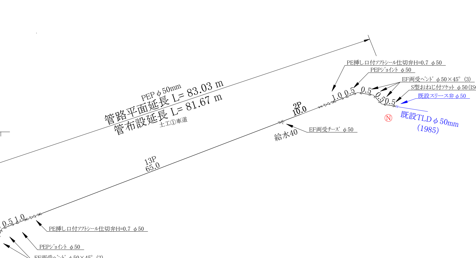
配管系統詳細図 S=Non 【4工区】
