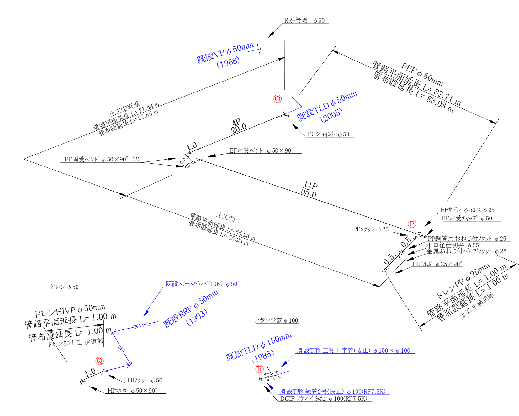
配管系統詳細図 S=Non 【5工区】
