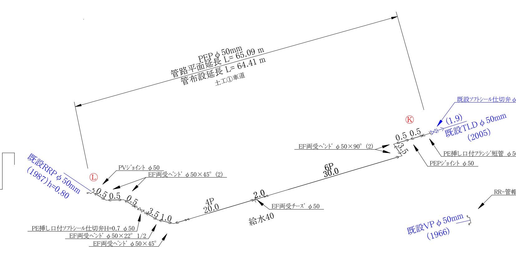
配管系統詳細図 S=Non 【3工区】
