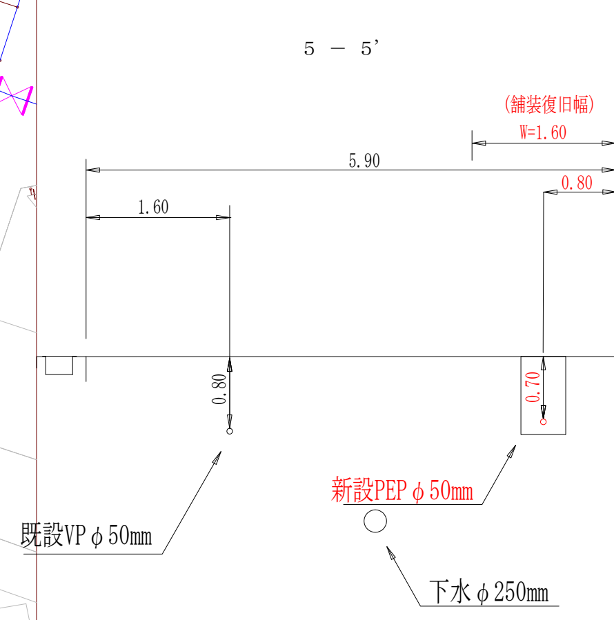
横断面図 S=Non 【3工区】
