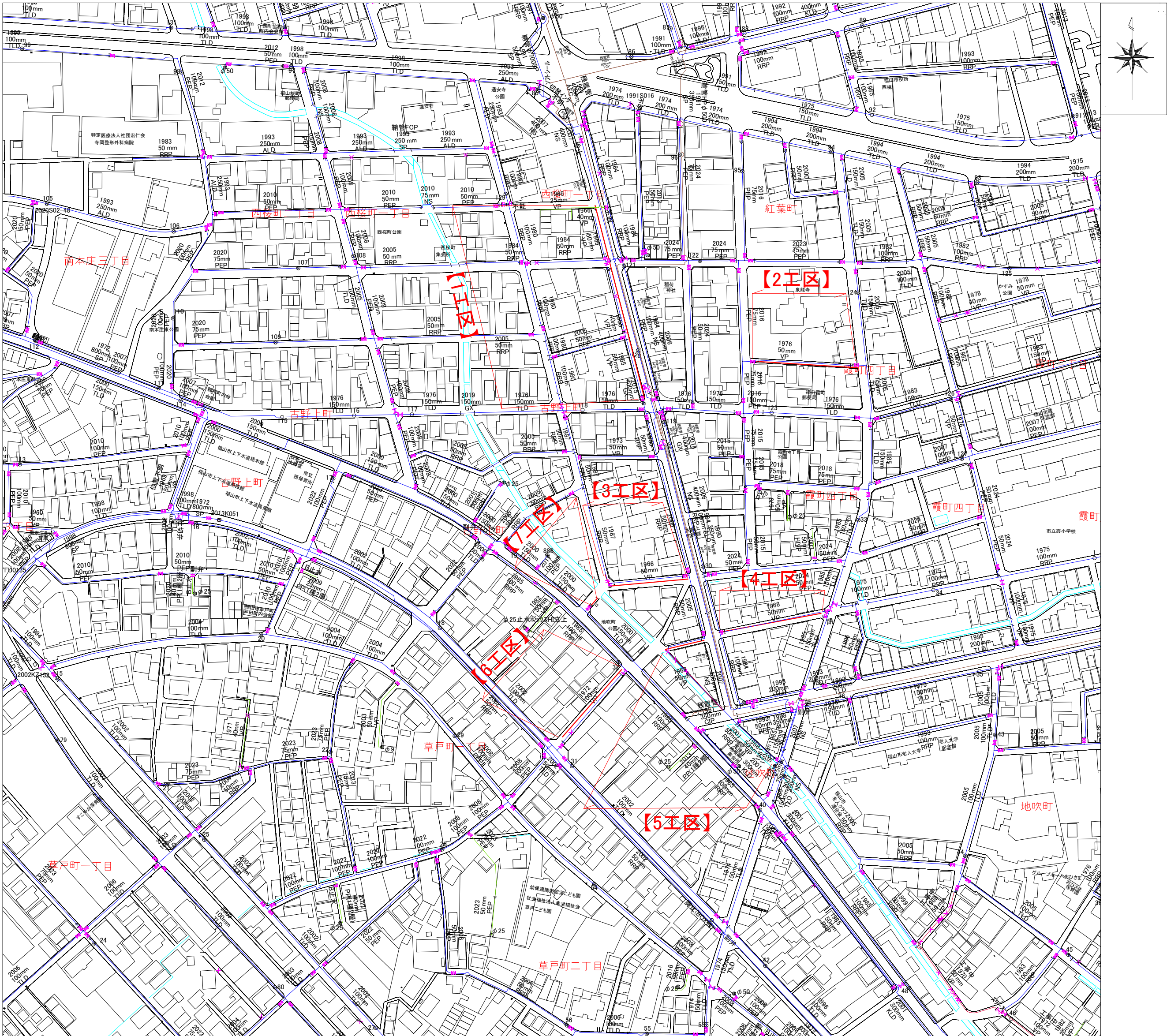
配管図 S=1/2,500
