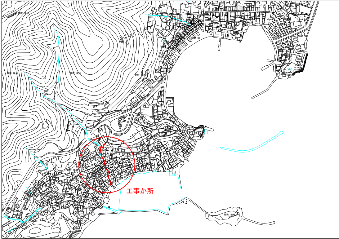
位置図 S=1/5000
