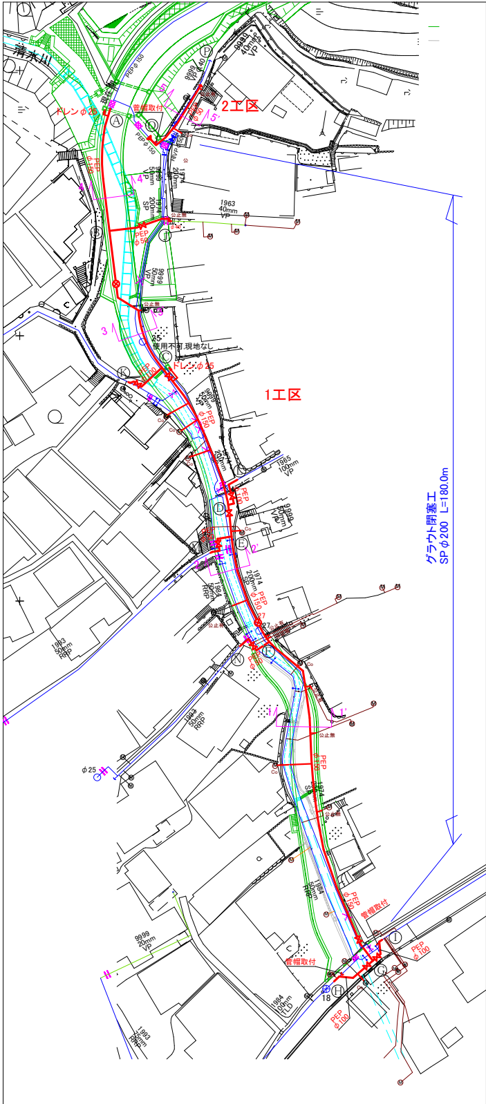
平面図 S=1/500
