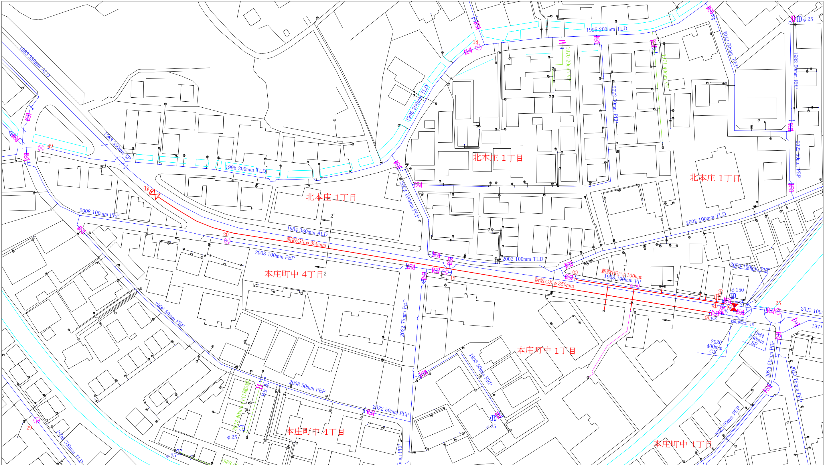
平面図 S=1/500
