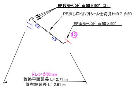
【ドレン③】
