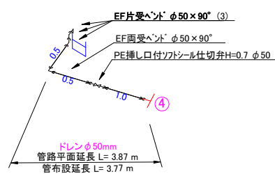
【ドレン①】
