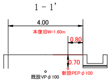
横断面図 S=1/100
