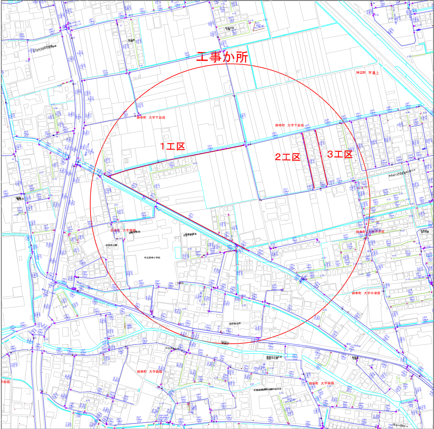
配管図 S:1/2500
