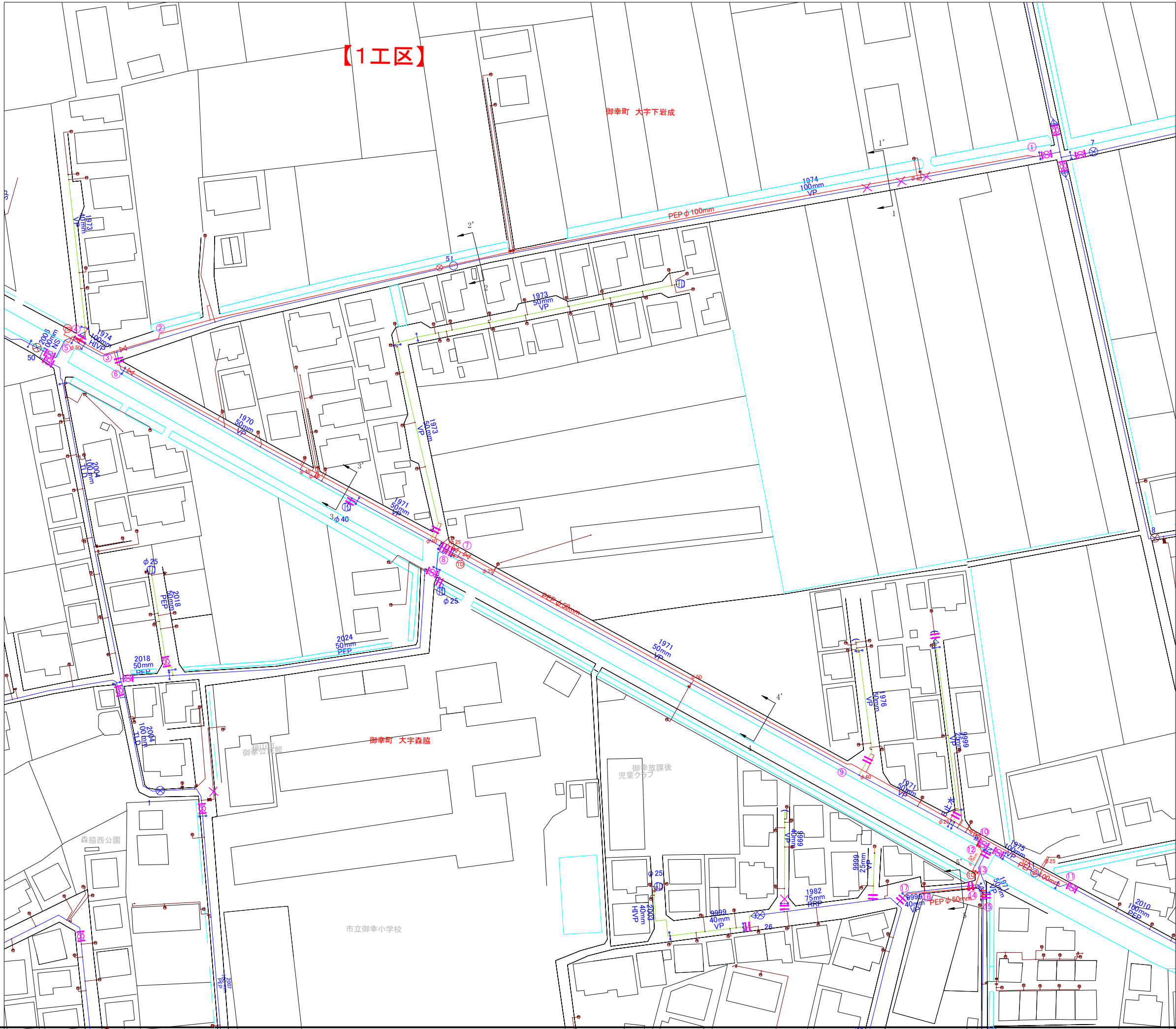
平面図 S=1/500 【1工区】
