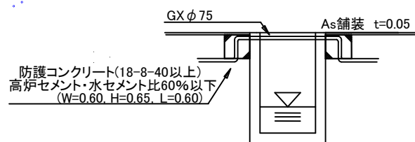
防護コンクリート標準施工図 S=NON
