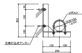
【ドレン②】
