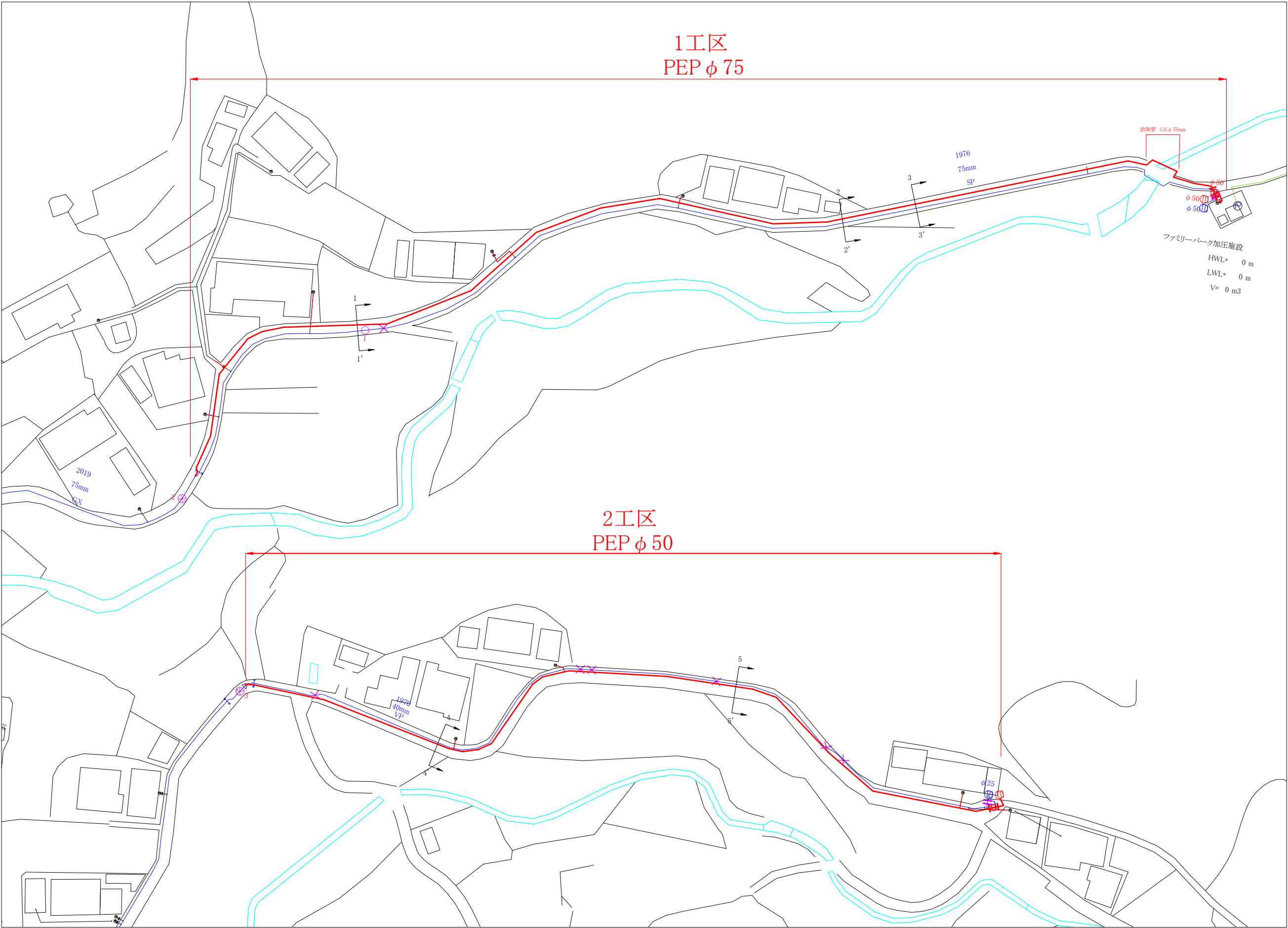
平面図 S=1/500
