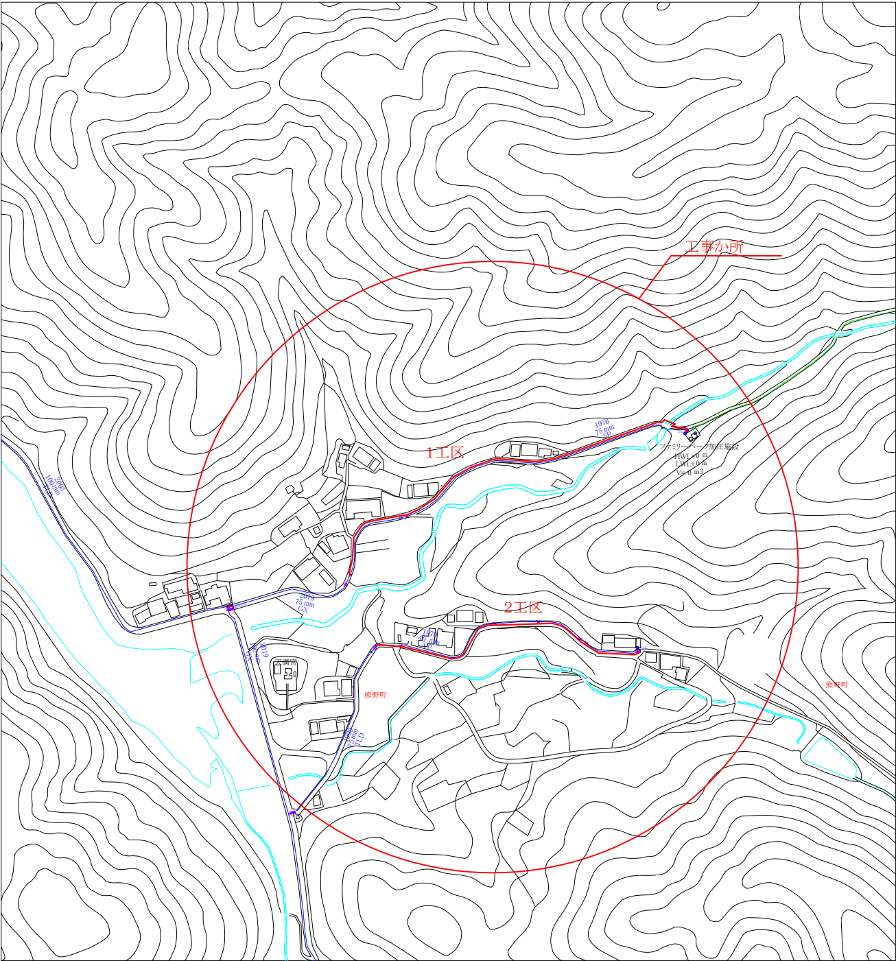
配管図 S=1/2500
