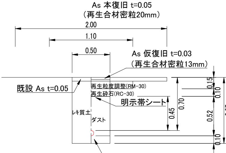
PEPφ50土工図③
