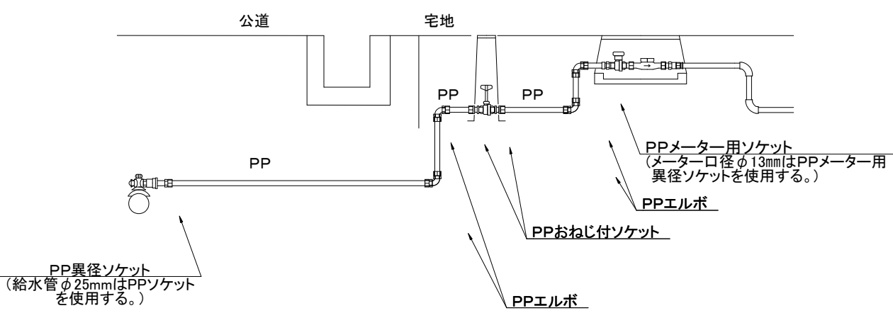
給水管切替標準施工図 S=NON
