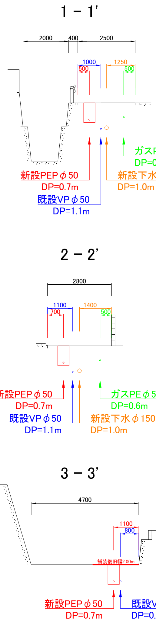
横断面図 S=1/100
