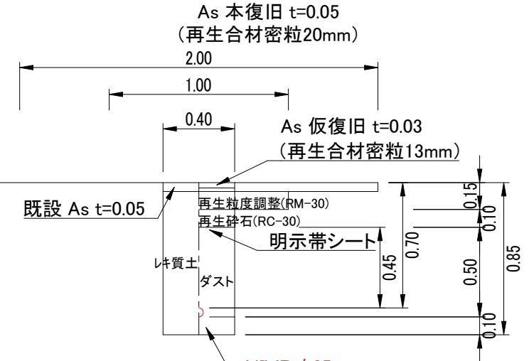
HIVPφ25土工図
