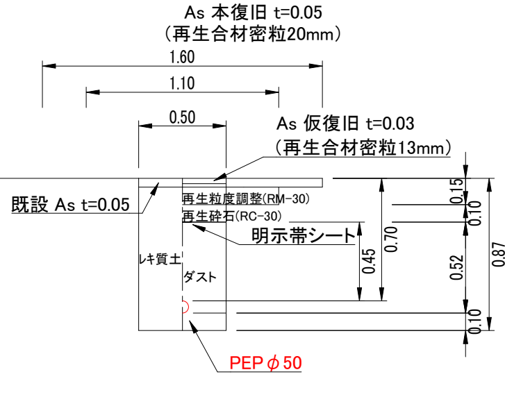
PEPφ50土工図②
