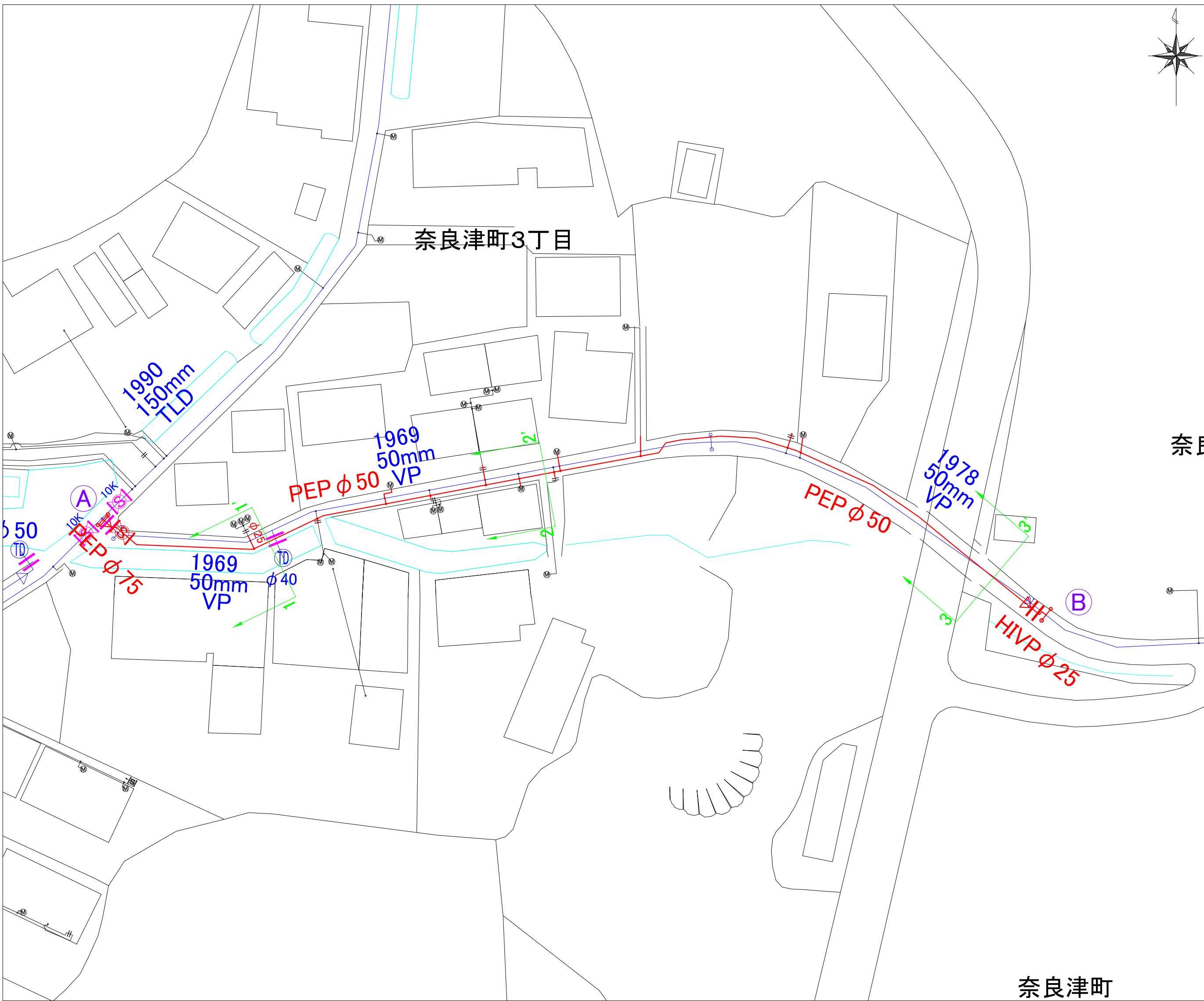
平面図 S=1/500
