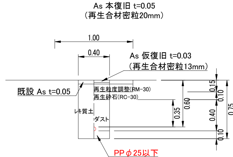
給水管φ25以下土工図②
