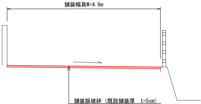
標準横断面 S=1/150
