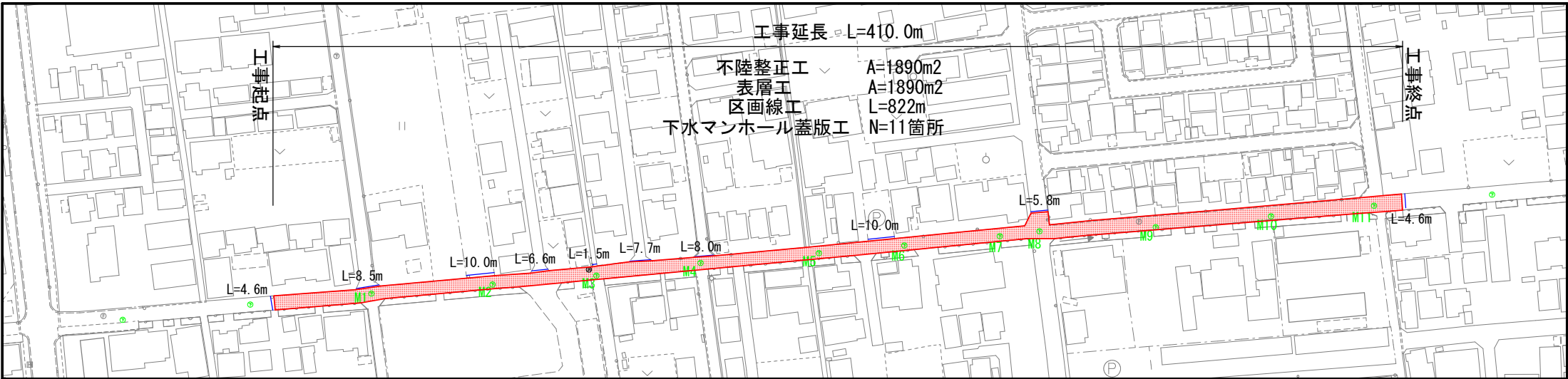
平面図 S=1/2000
