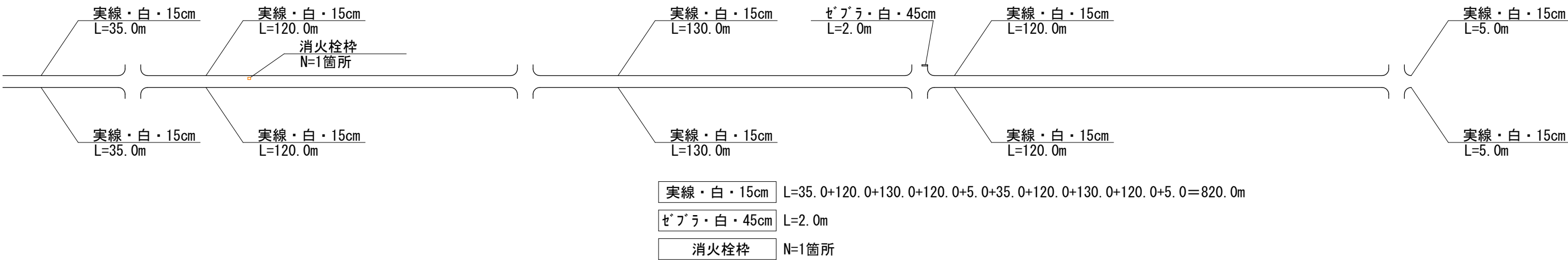
区画線展開図 S=1/500
