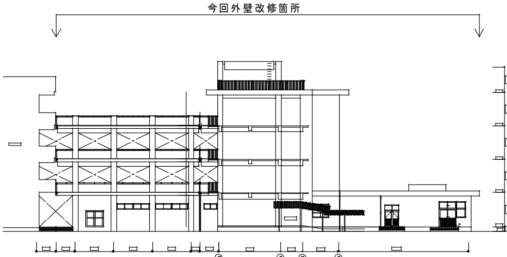
東面立面図（北棟） S=1/300
