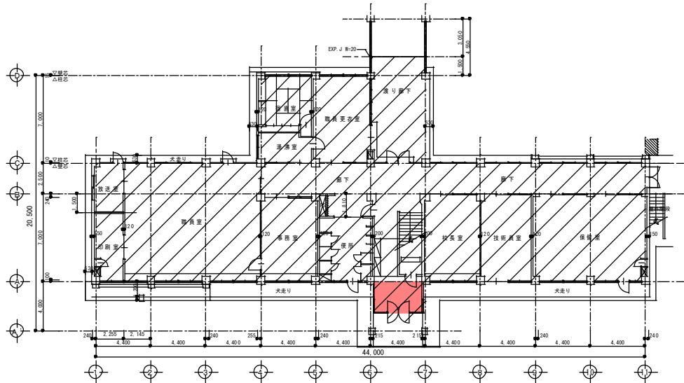
1階平面図 S=1/300
