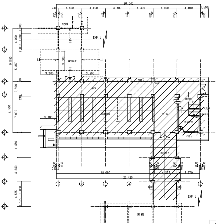
1階平面図 S=1/300
