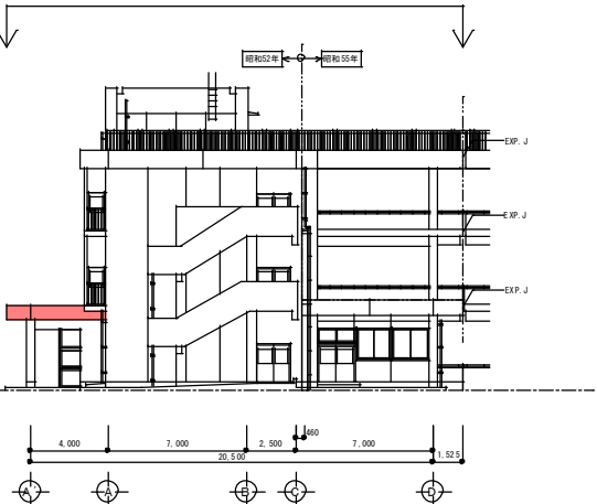
東立面図 S=1/300
