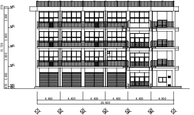
南面立面図 S=1/300
