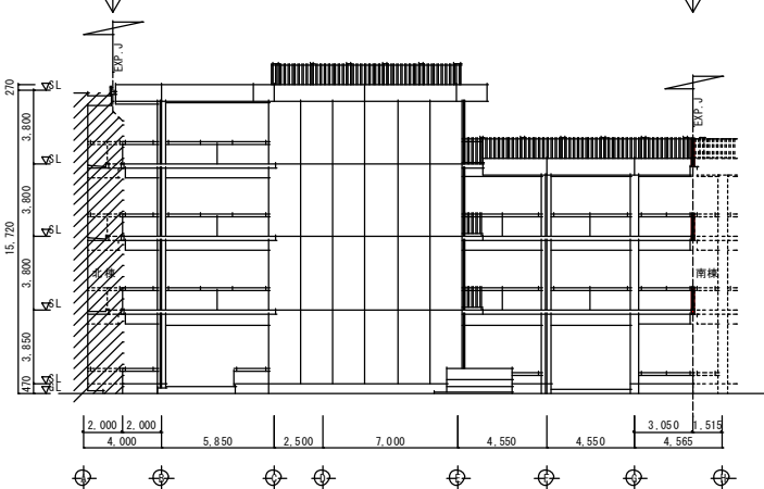
西面立面図 S=1/300
