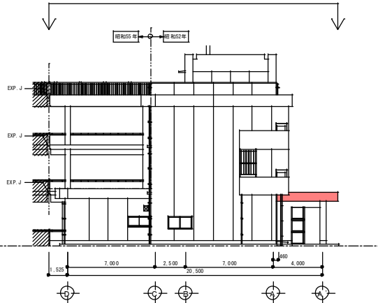
西面立面図 S=1/300
