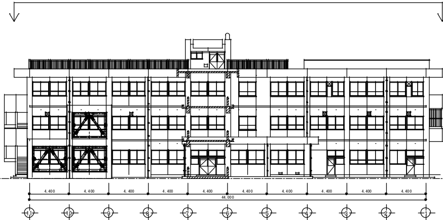
北面立面図 S=1/300
