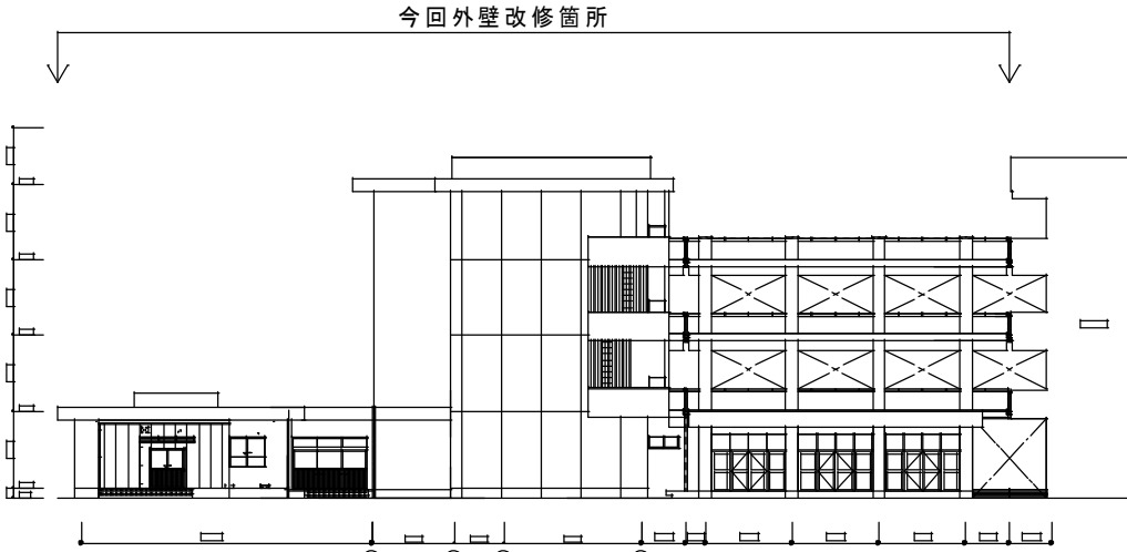
西面立面図 S=1/300
