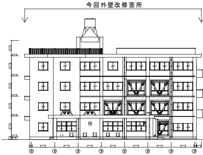
北面立面図（北棟） S=1/300
