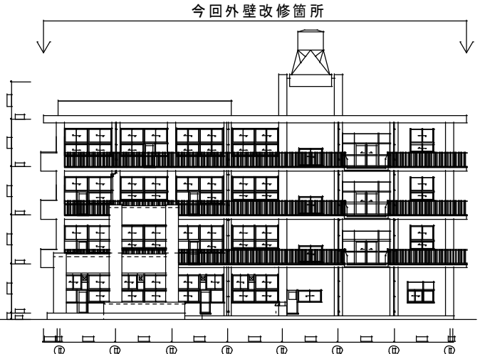
南面立面図 S=1/300
