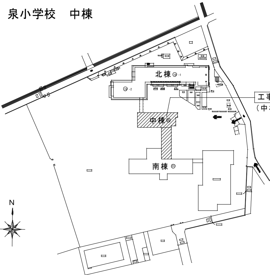
配置図 S=1:1000
