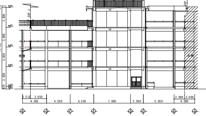
東立面図 S=1/300
