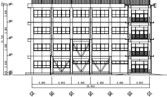
北面立面図 S=1/300
