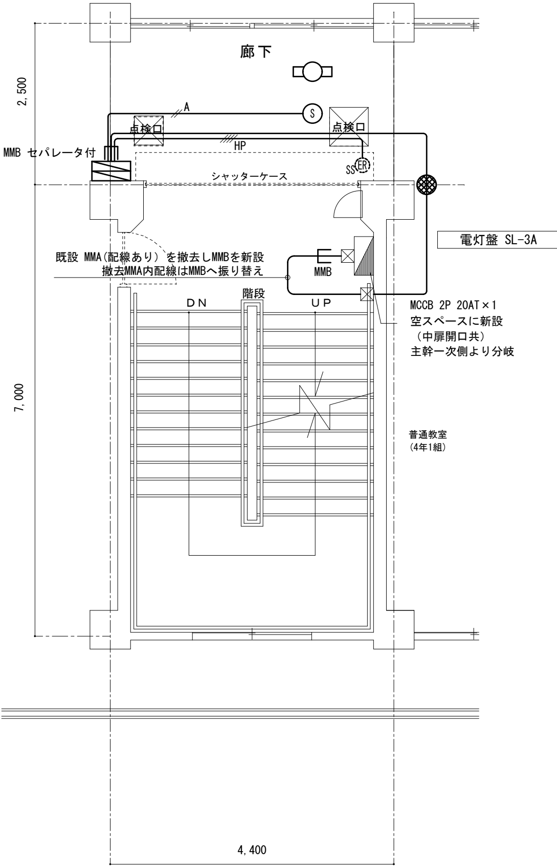
南棟 3 階 東側 平面詳細図 S=1/60
