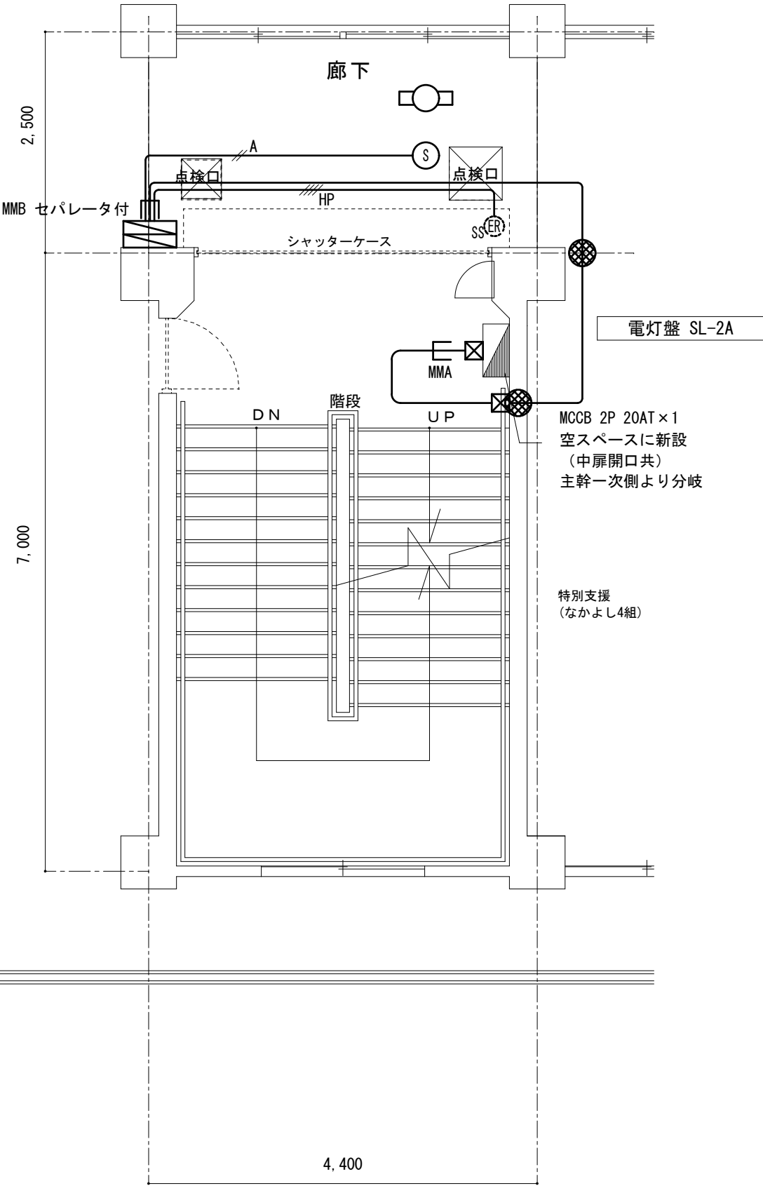
南棟 2 階 東側 平面詳細図 S=1/60
