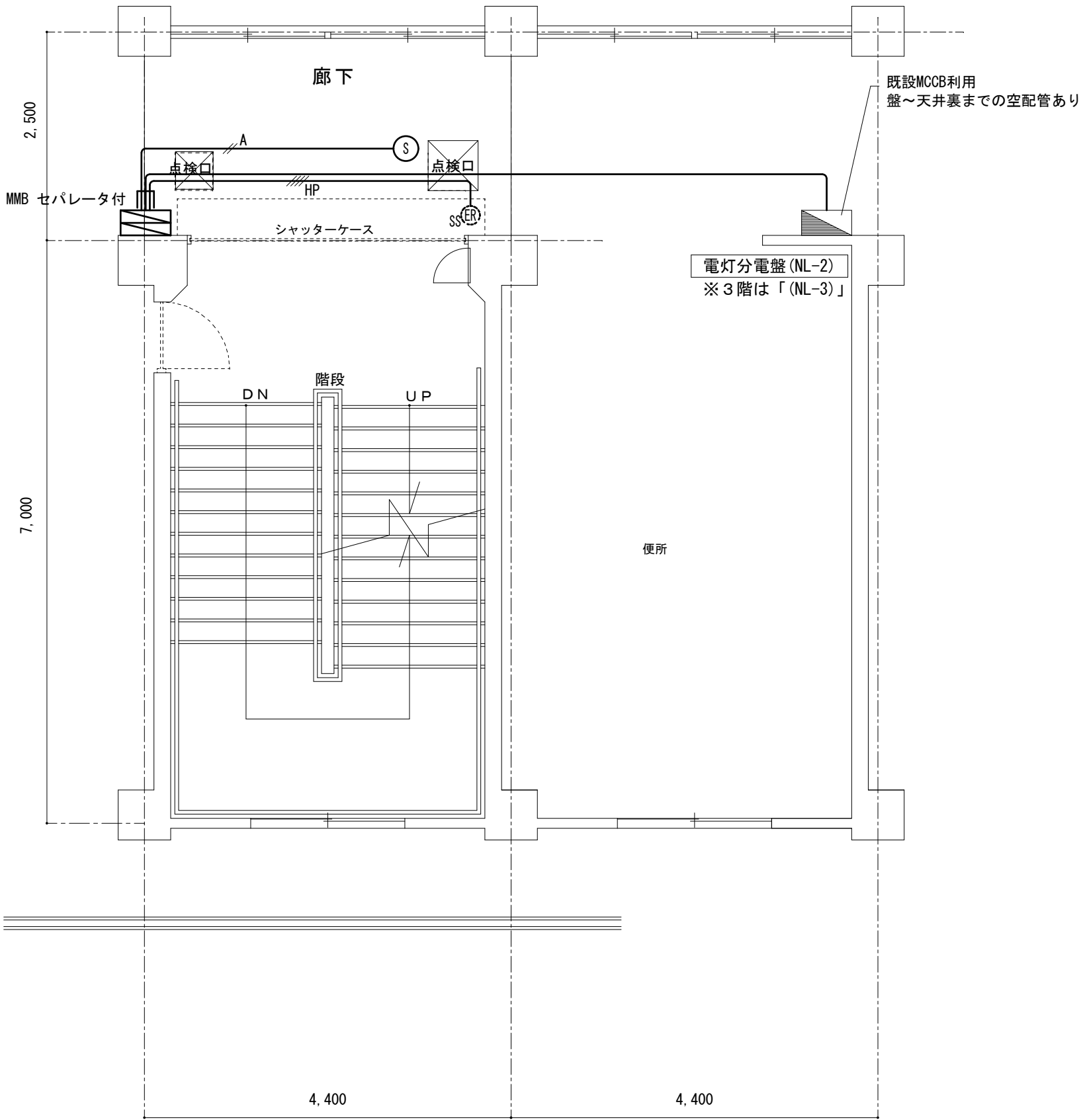
北棟 2, 3 階 平面詳細図 S=1/60
