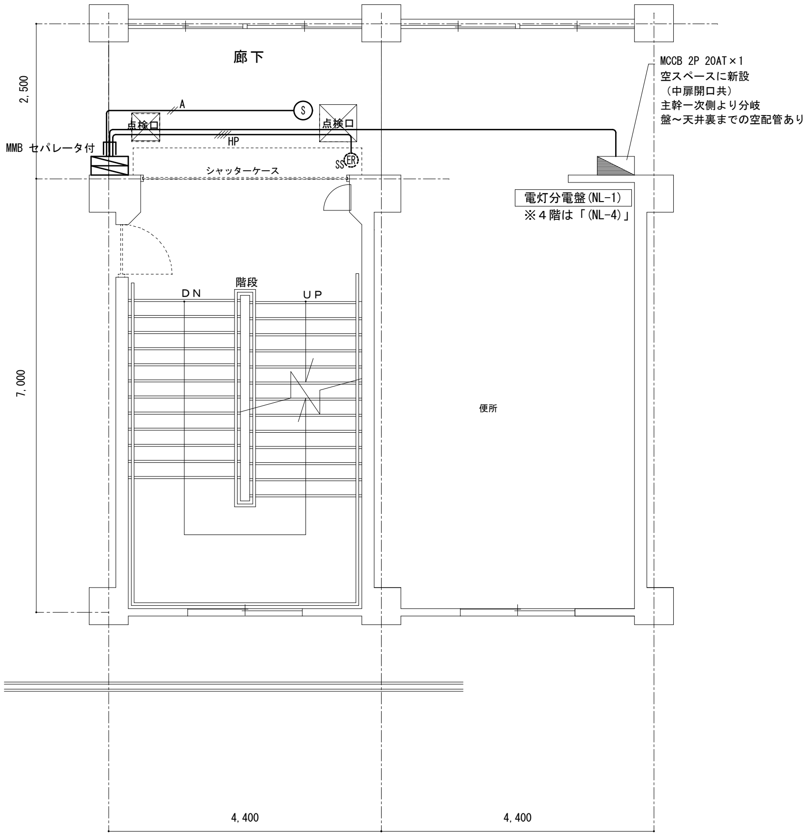
北棟 1, 4 階 平面詳細図 S=1/60 ※ 4 階は防火戸が便所側
