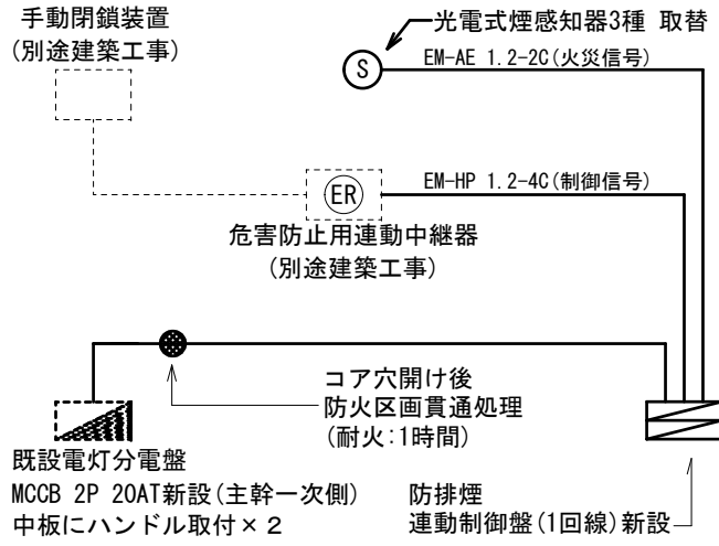
系統図 S=NonScale
