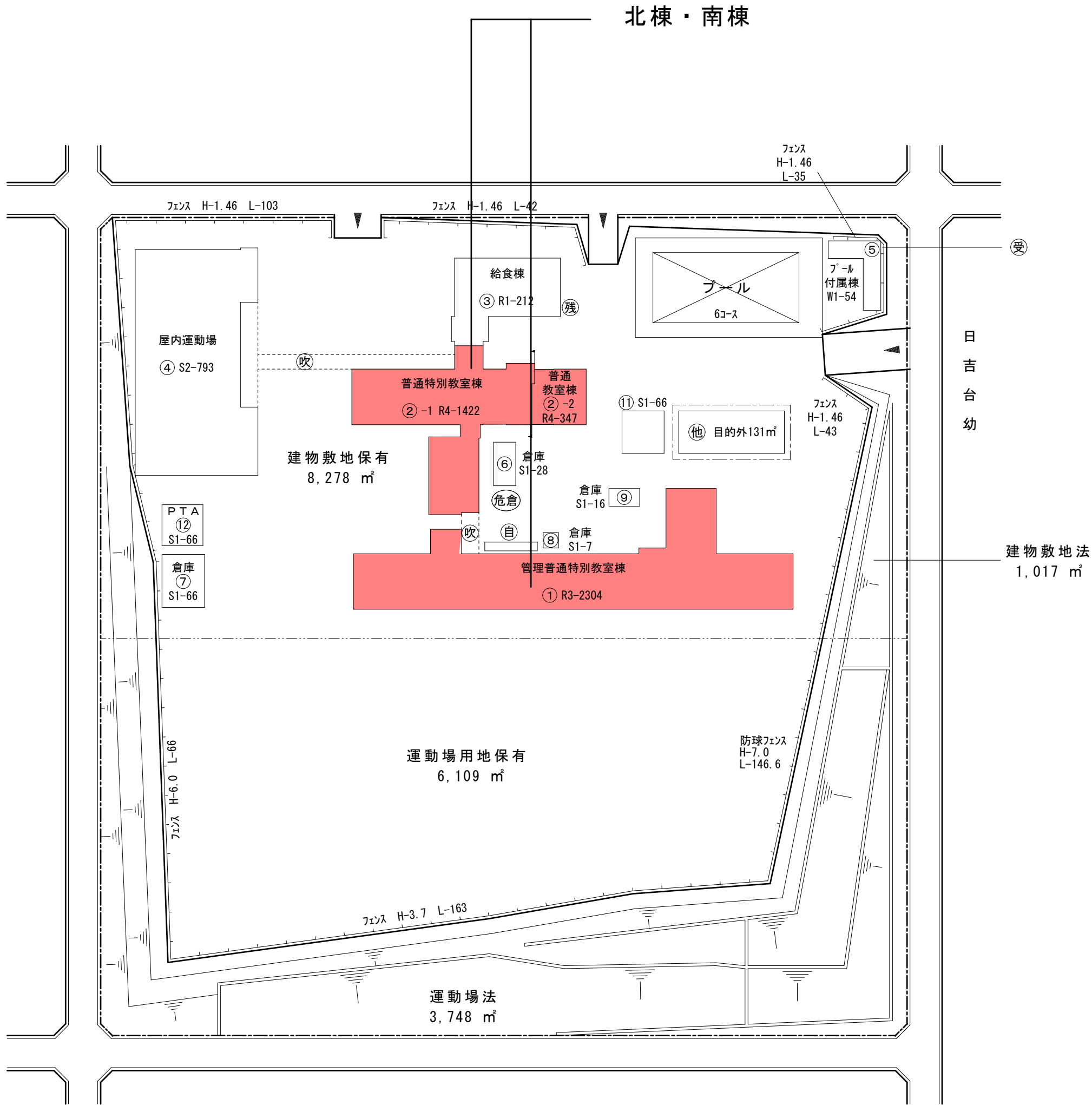
配置図 S=1/800
