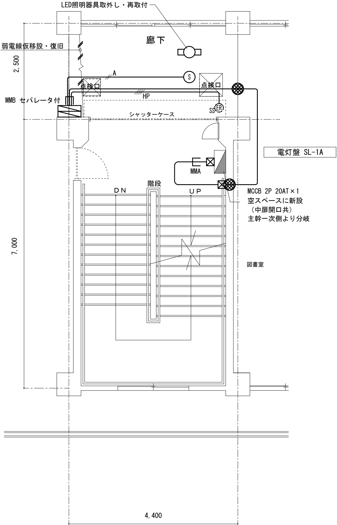
南棟 1 階 東側 平面詳細図 S=1/60
