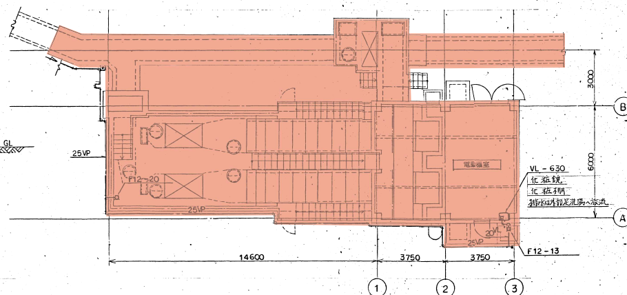
平面图 1/100
