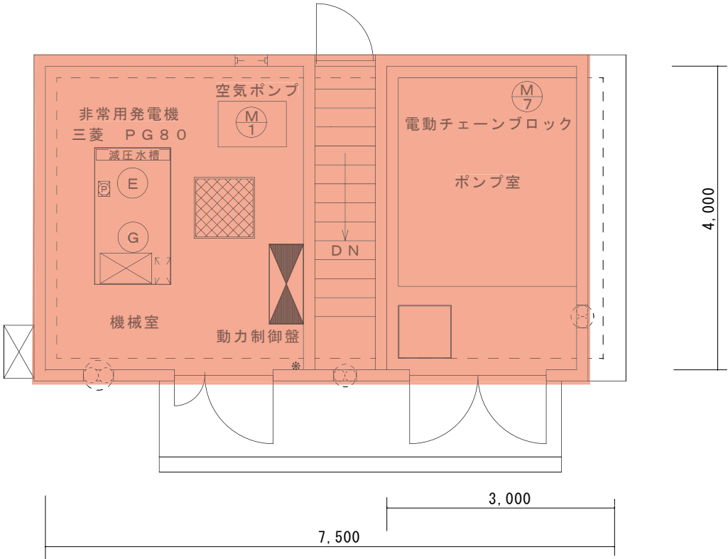
1 階平面図 S : 1 / 50
