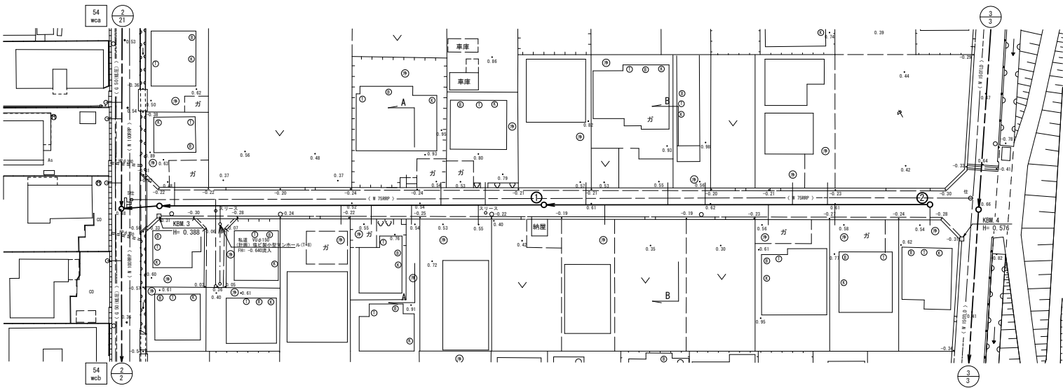
管渠埋設平面図 S = 1:500
