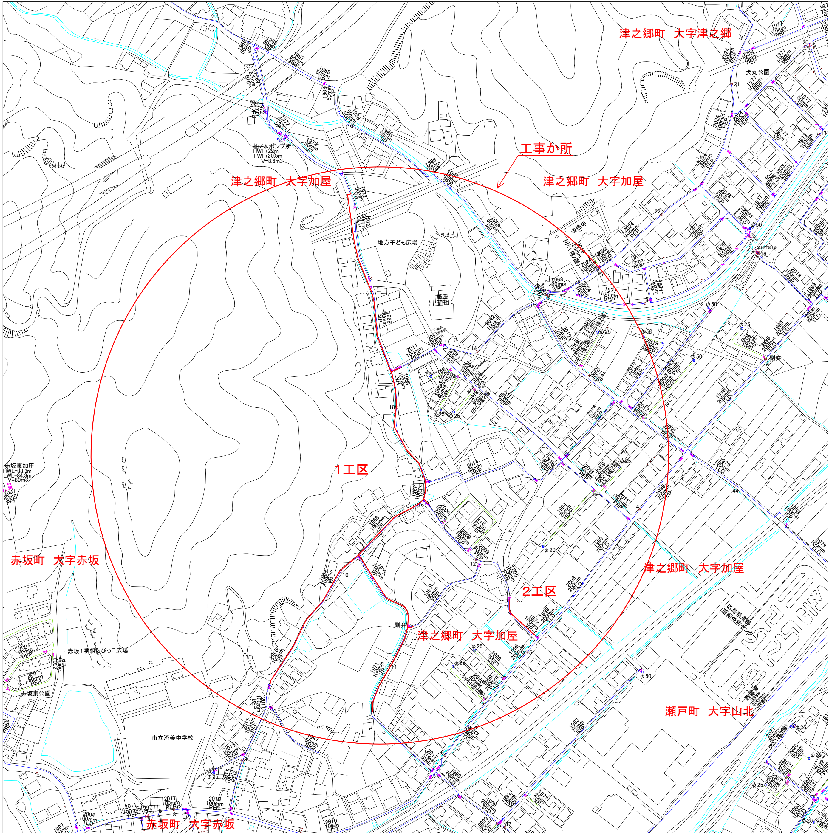
配管図 S=1:2500
