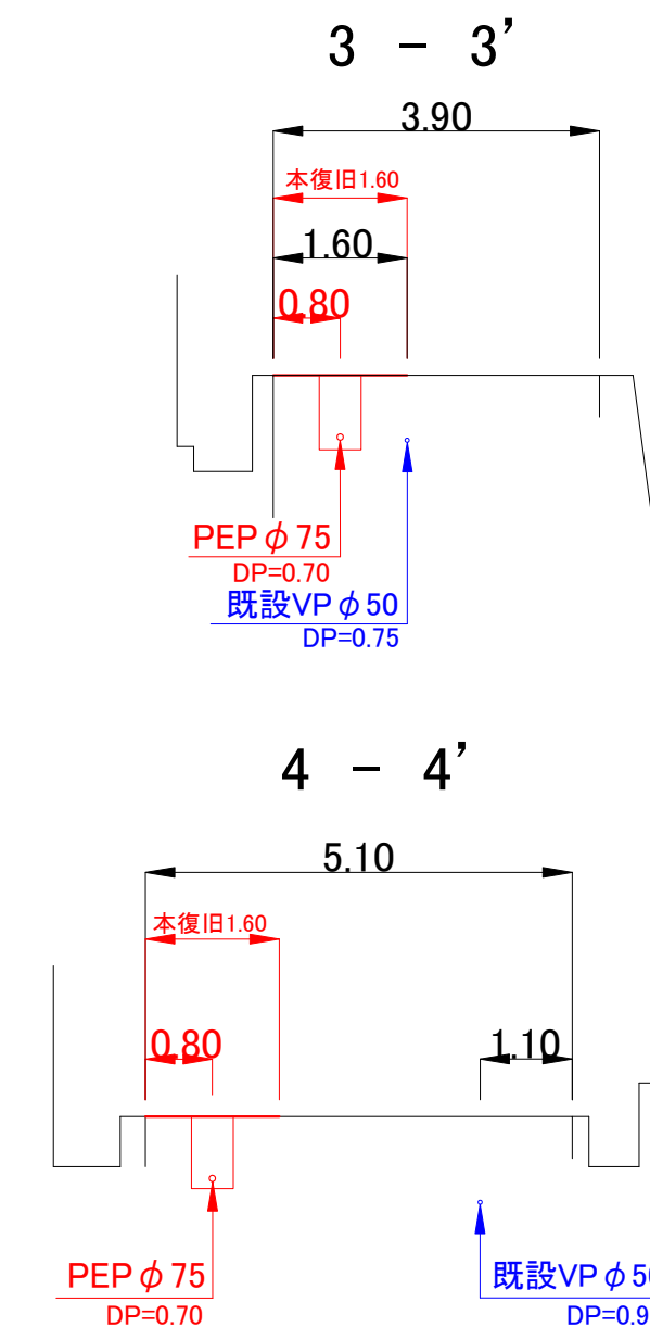
横断面図(2) S=1:100
