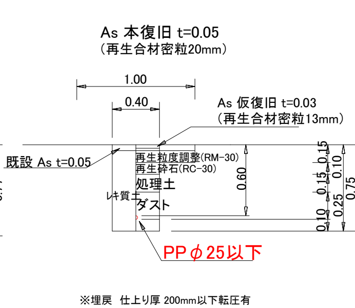
給水管 φ 25以下土工図
