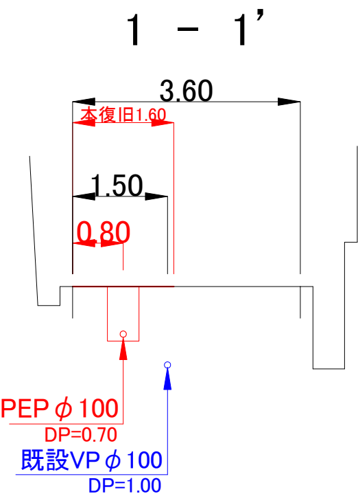
横断面図(1) S=1:100
