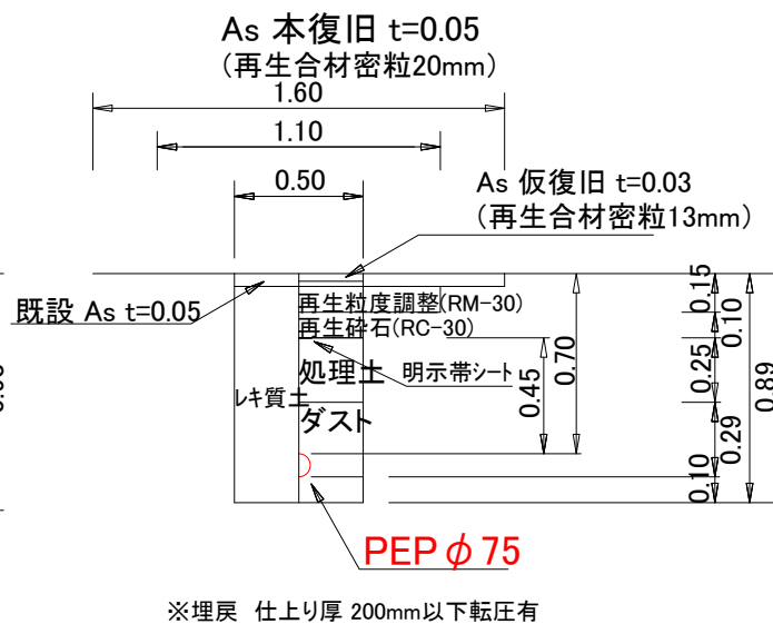
給水管 φ 25以下土工図
