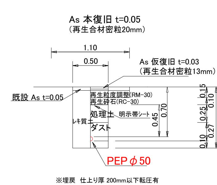
ドレン φ 50土工図
