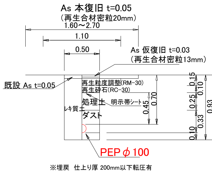
給水管 φ 50土工図
