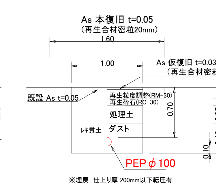
消火栓土工図
