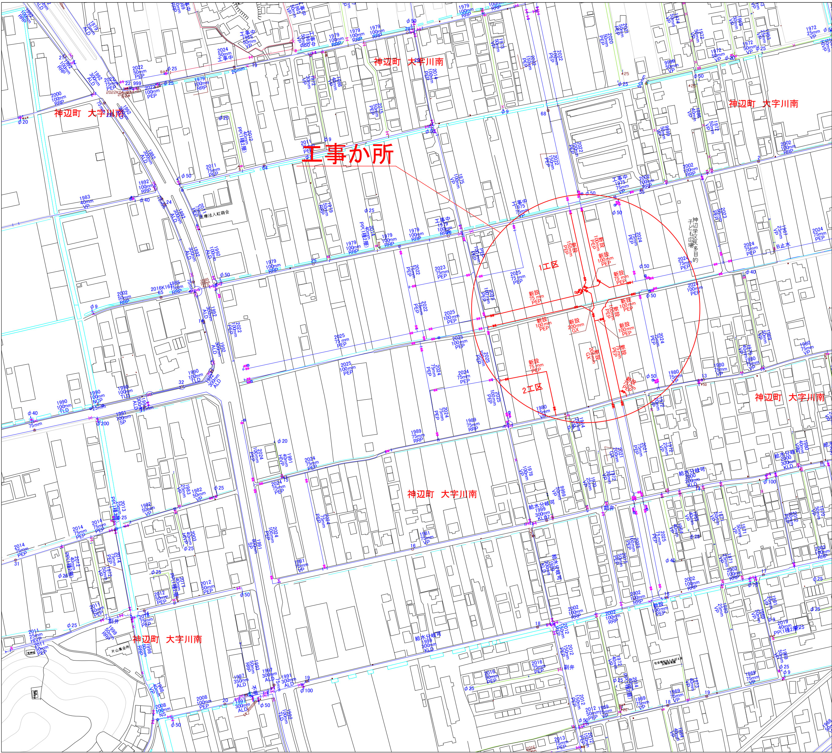
配管図 S=1:2500
