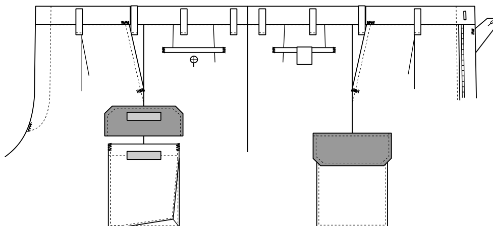
ズボン詳細図
