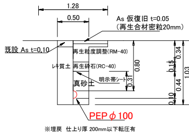
PEPφ100土工図
