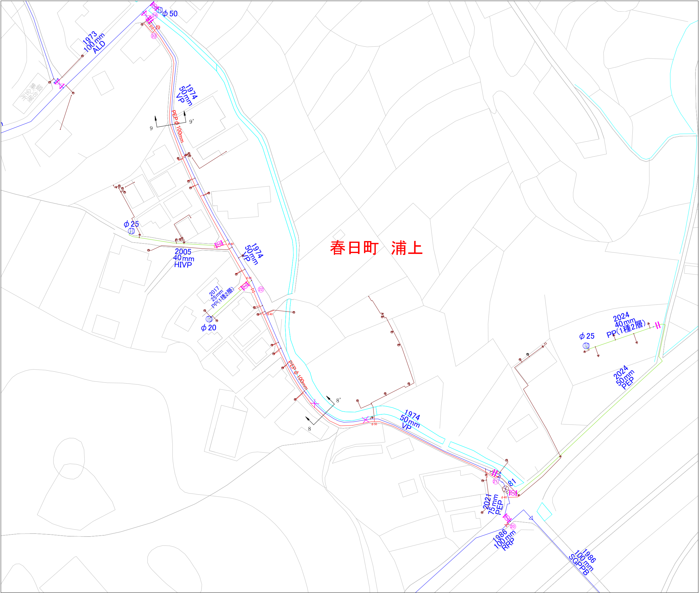
平面図 S=1/500
