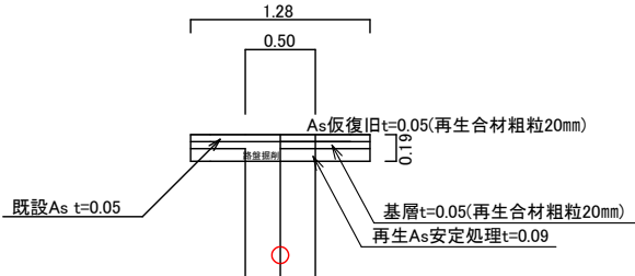
基層工・安定処理工
