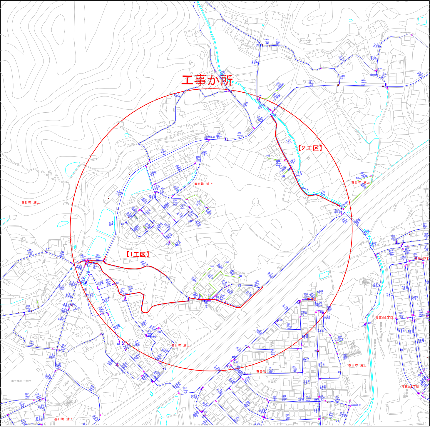
配管図 S:1/2500
