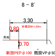
横断面図 S=1/100
