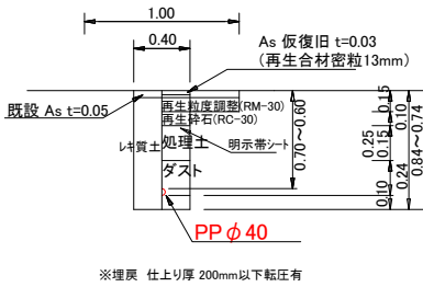
消火栓土工図
