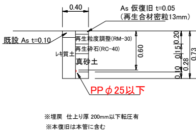
ALDφ100撤去土工図
