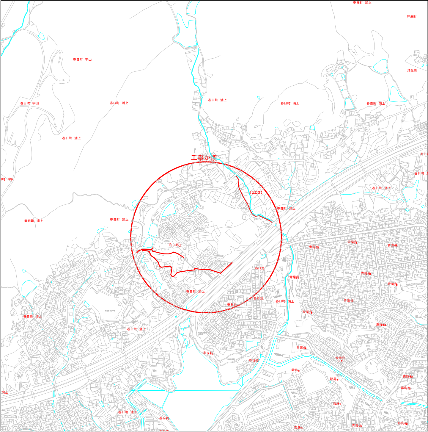
位置図 S:1/5000
