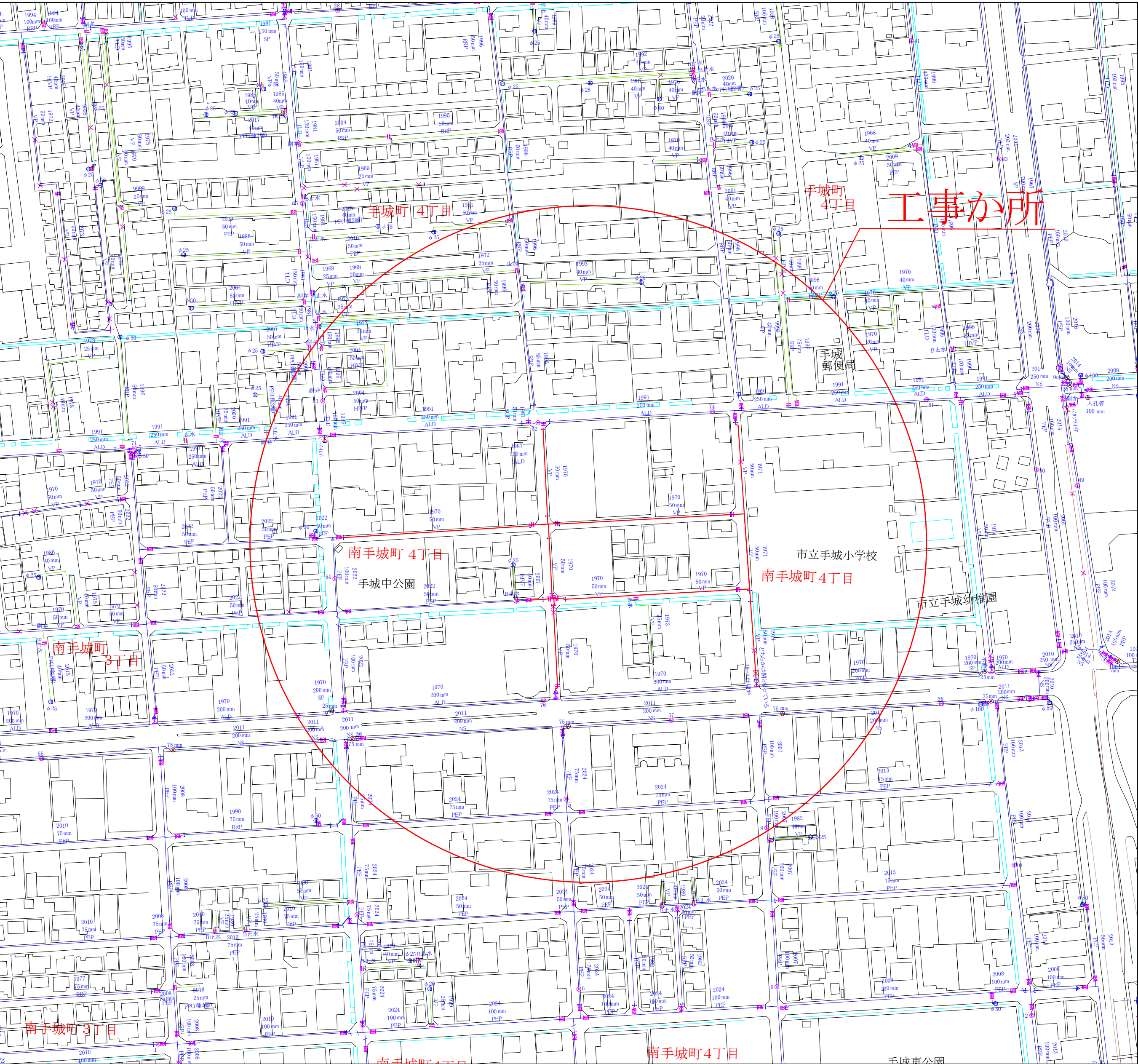
配管図
