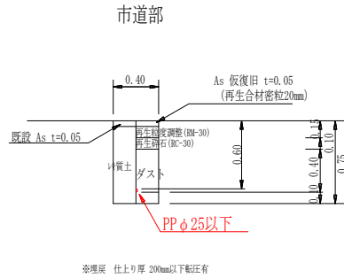
給水管 φ 25以下土工図②
