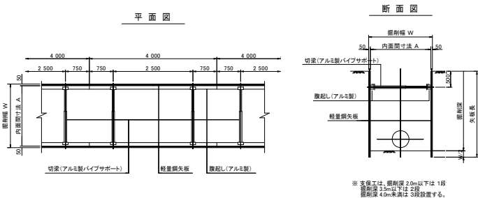
復旧断面図 S=1/30
