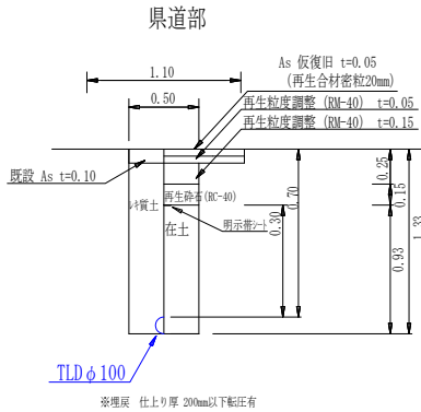
TLD φ 100撤去土工図
