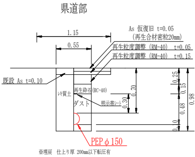
PEP φ 150土工図②
