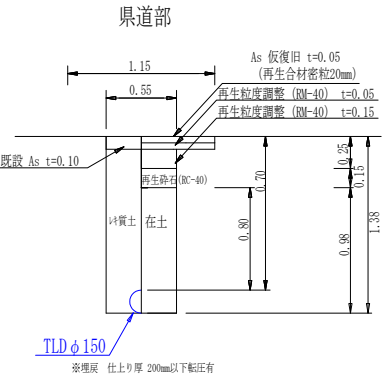
TLD φ 150撤去土工図
