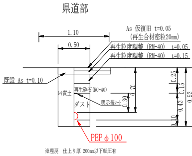
PEP φ 100土工図①
