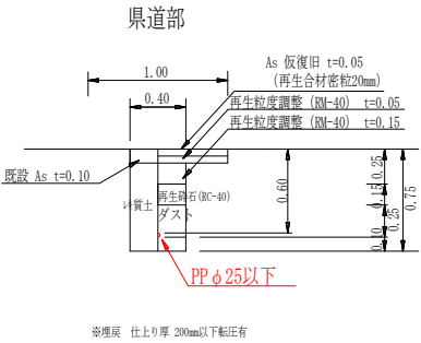
給水管 φ 25以下土工図①
