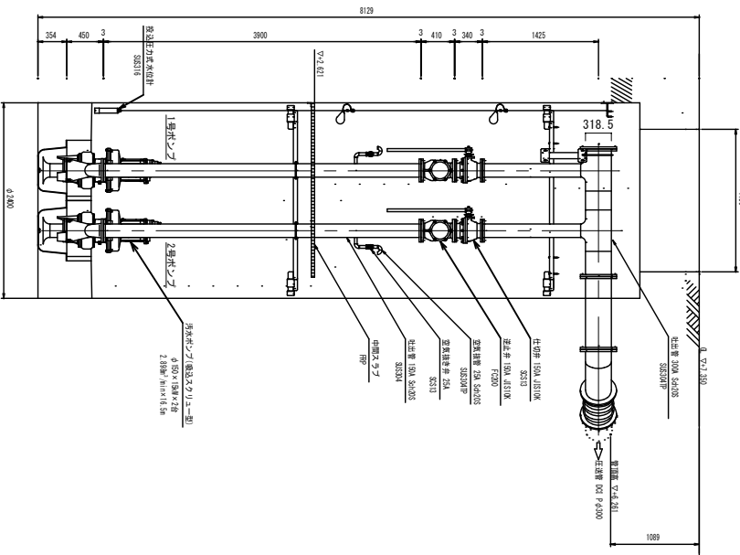
A-A 断面図
