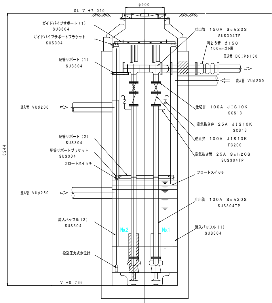
マンホール断面図
