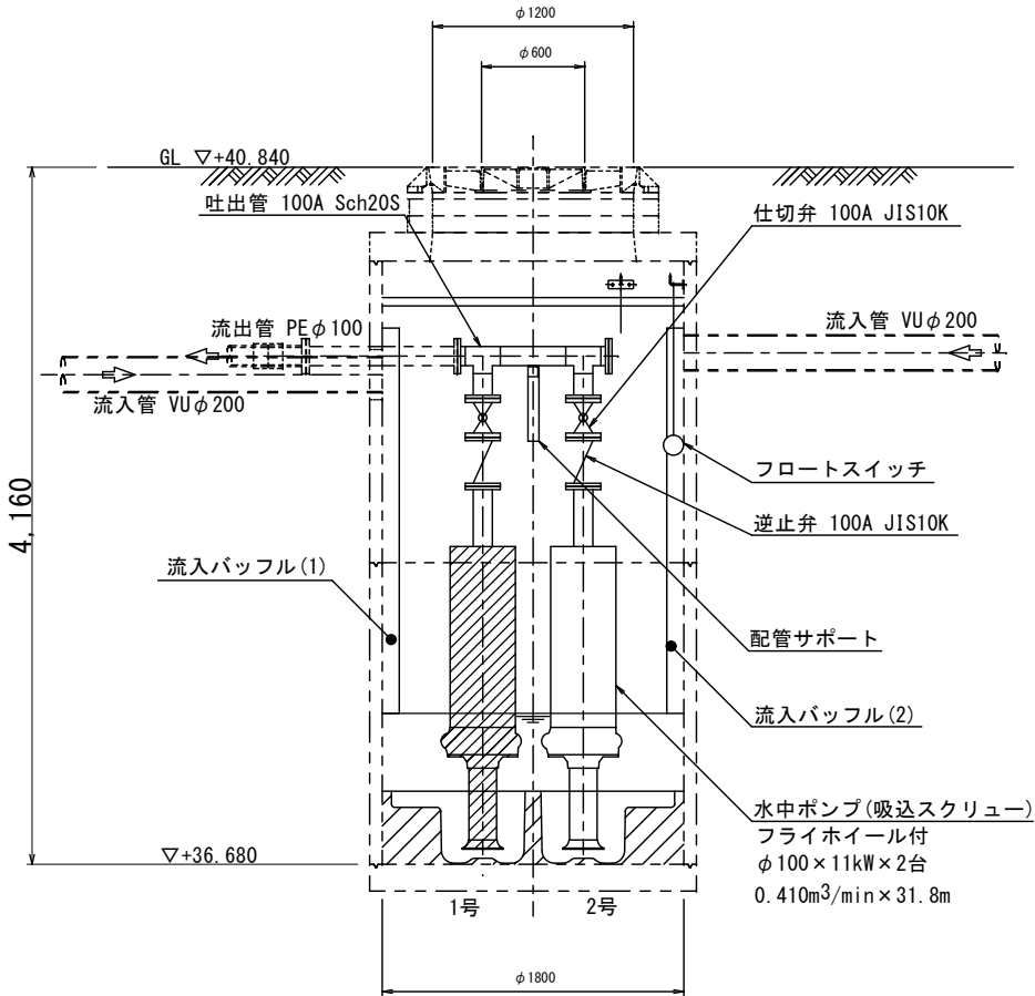
マンホール断面図
