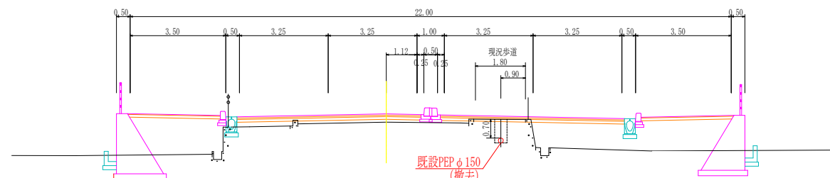
\underline{2 - 2'}
