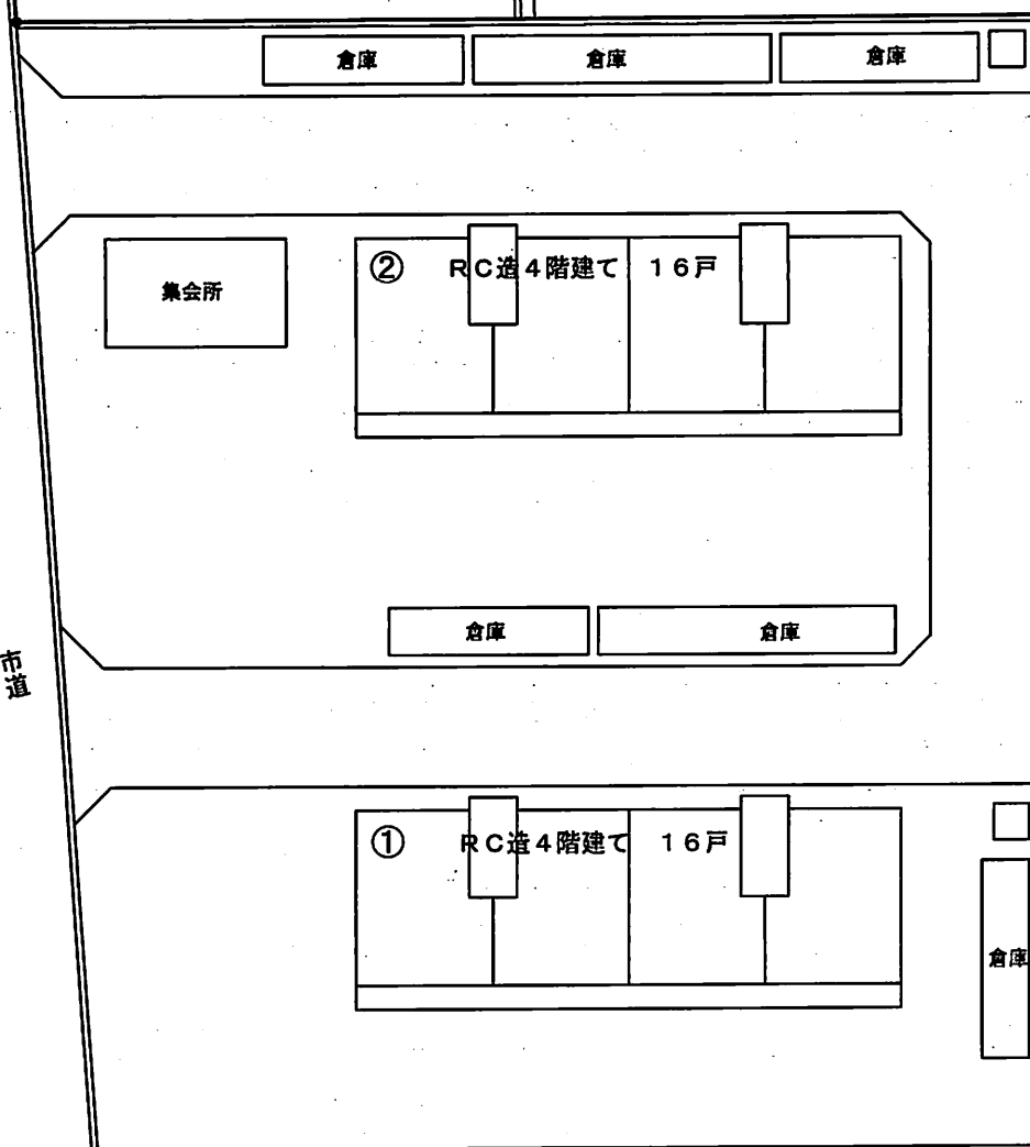
配置図 1:500
