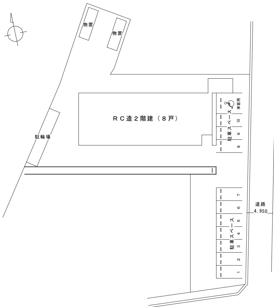
配置図 Non Scale
