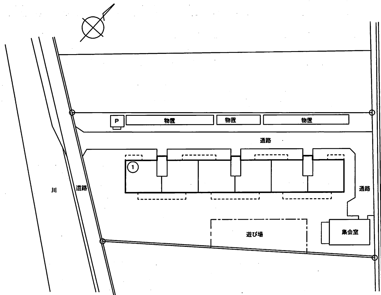
配置図
