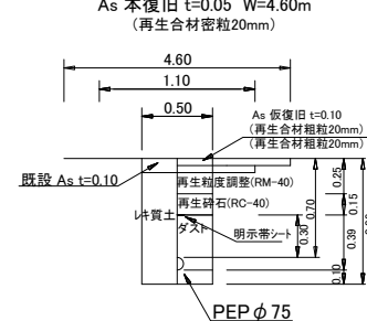
県道部PEPφ75土工図⑤
