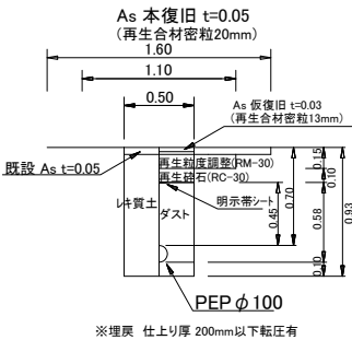
PEPφ100土工図②
