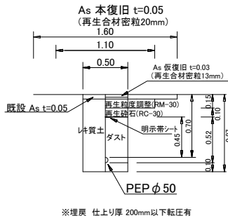
PEP・トレンφ50土工図⑥
