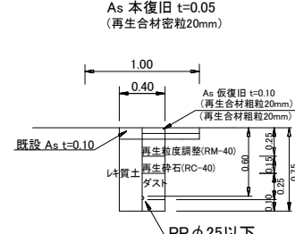
県道部給水管φ25以下土工図⑨
