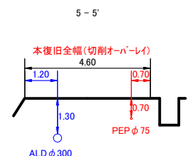
横断図 S=1/100
