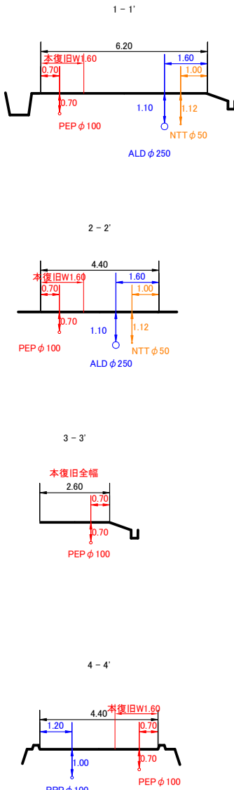
横断面 S=1/100
