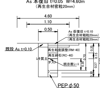
県道部レンφ50土工図⑦
