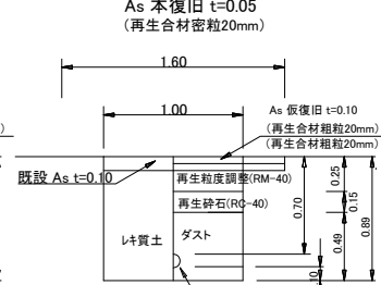
県道部消火栓土工図⑫
