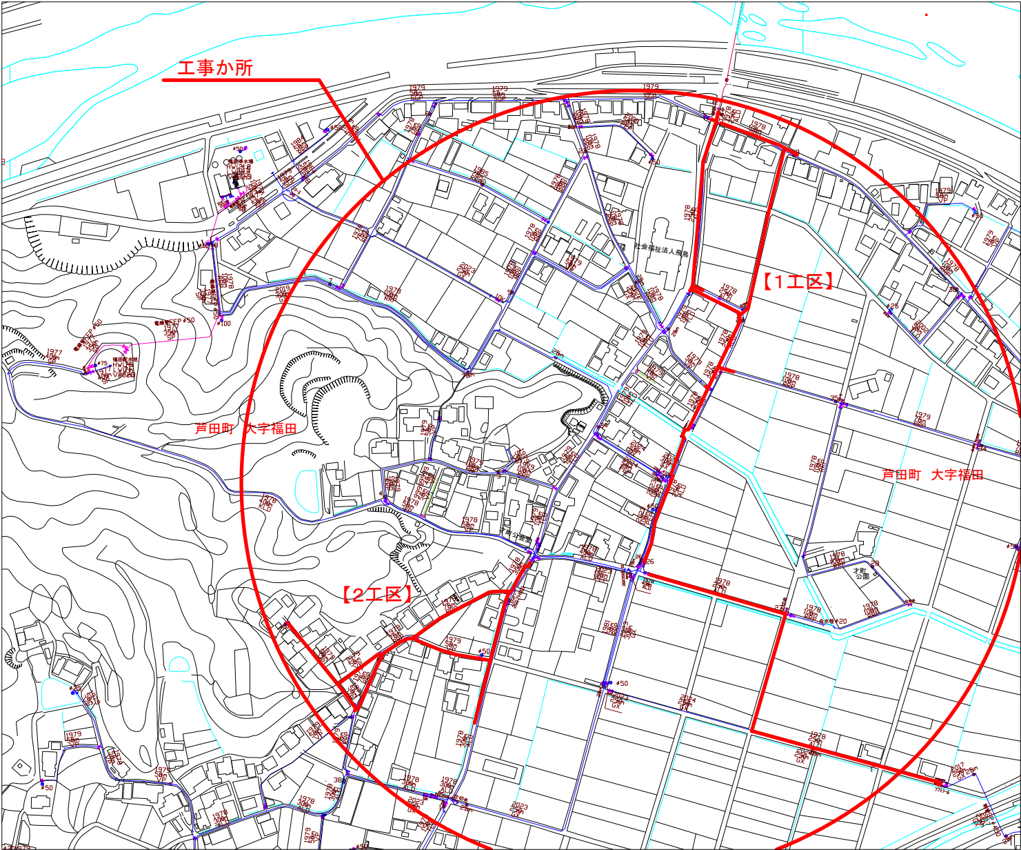
位置図 S=1/5000
