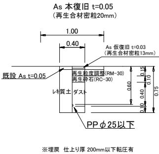
給水管φ25以下土工図⑧
