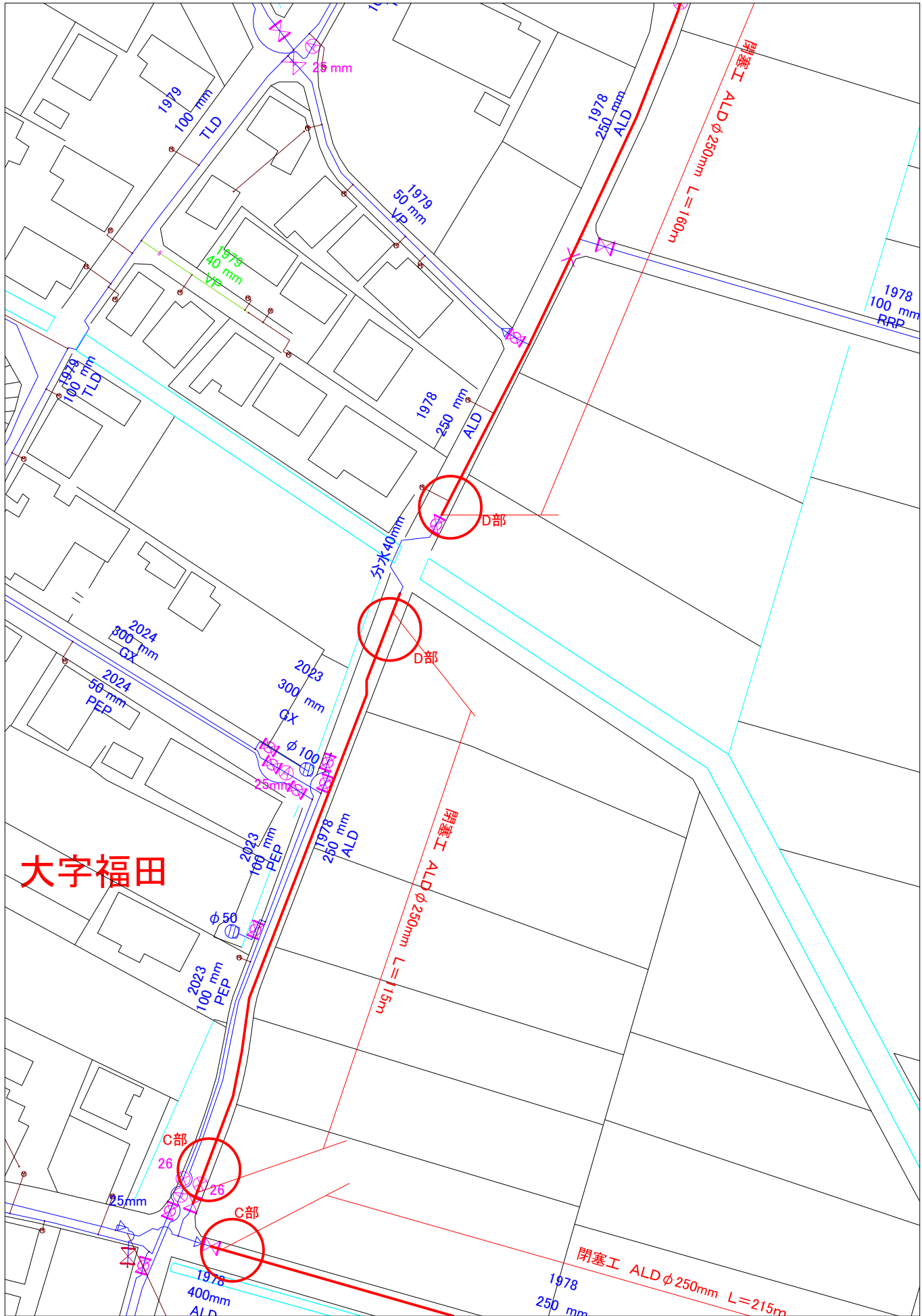
工 事 名 配水管布設工事(配整7-13) 工 事 場 所 福山市芦田町地内 図 面 平面図・土工図・閉塞詳細図 図面番号 6/6 縮 尺 図示 福 山 市 上 下 水 道 局 設計年月：2025年6月 原図サイズ：A1
