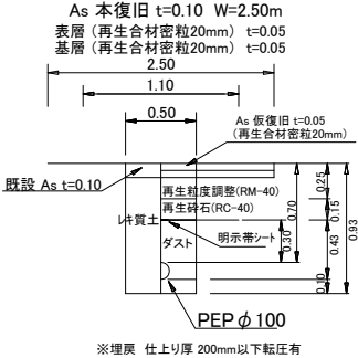
県道部PEPφ100土工図③
