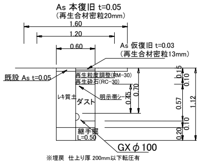
GXφ100土工図①
