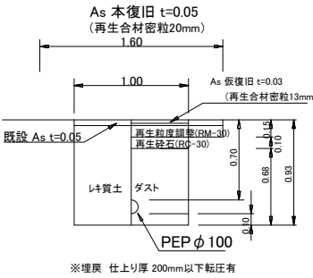
消火栓土工図⑩
