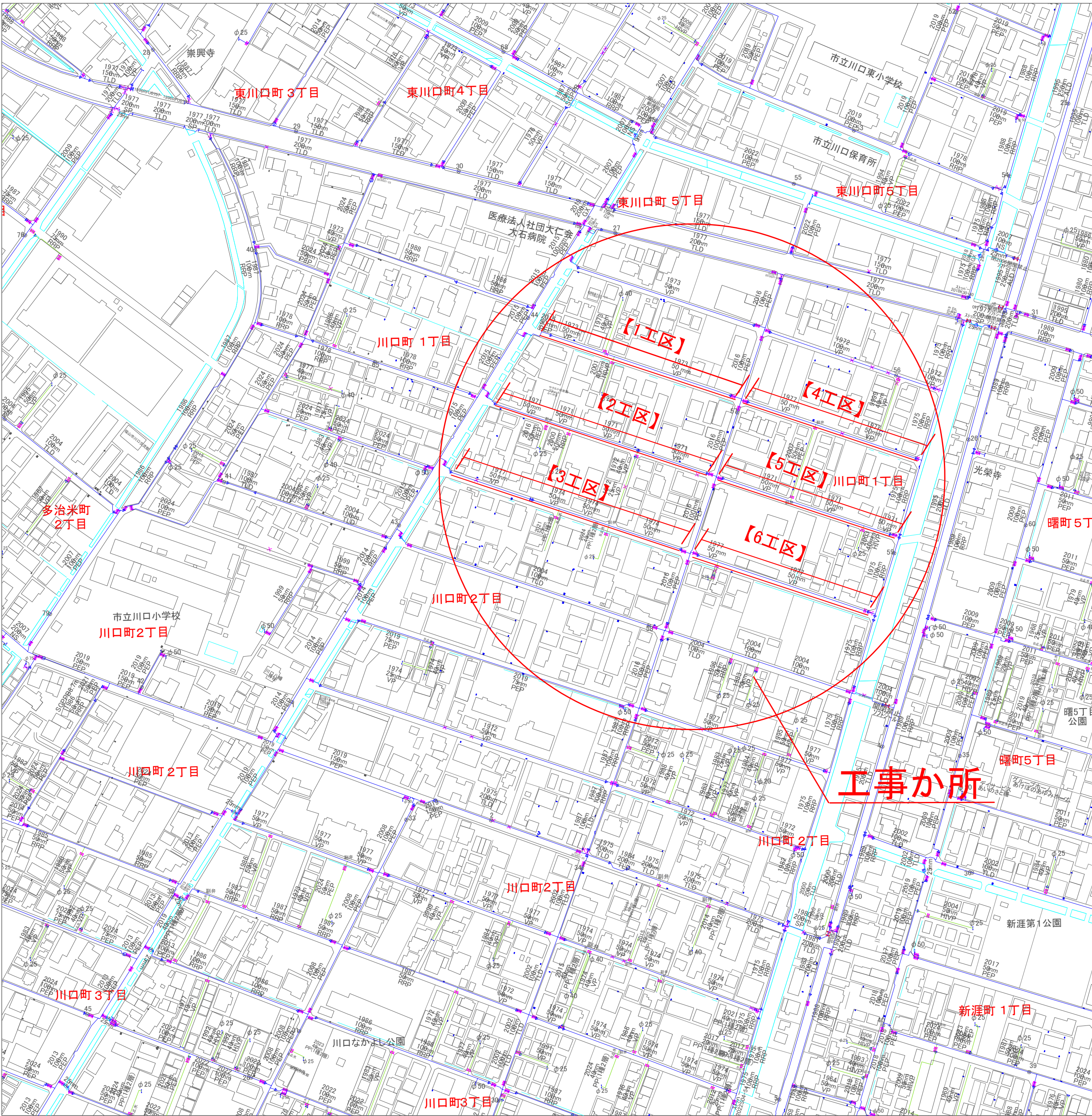
配管図 S=1/2500
