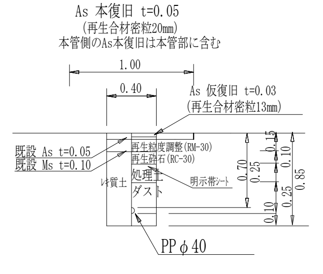
給水管 φ 40土工図②
