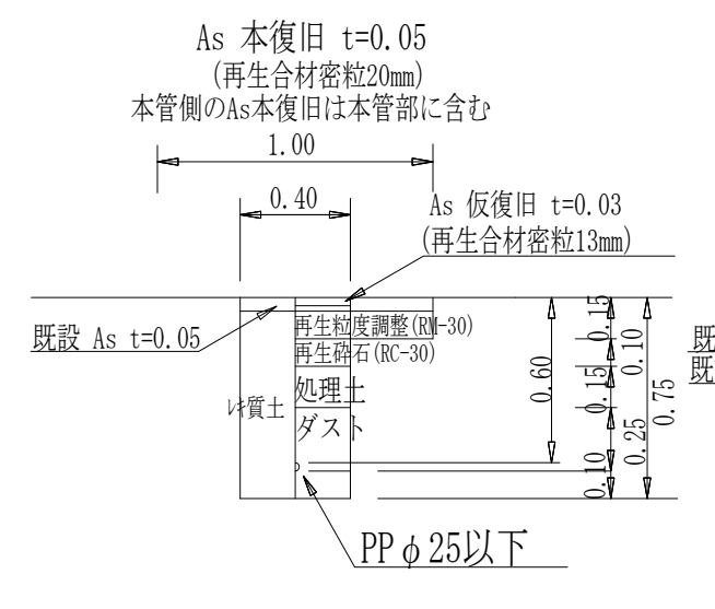
給水管 φ 25以下土工図①
