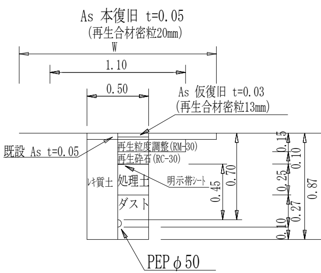
PEP φ 50土工図①
