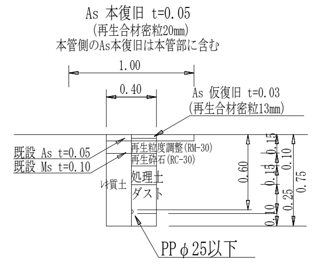
給水管 φ 25以下土工図②
