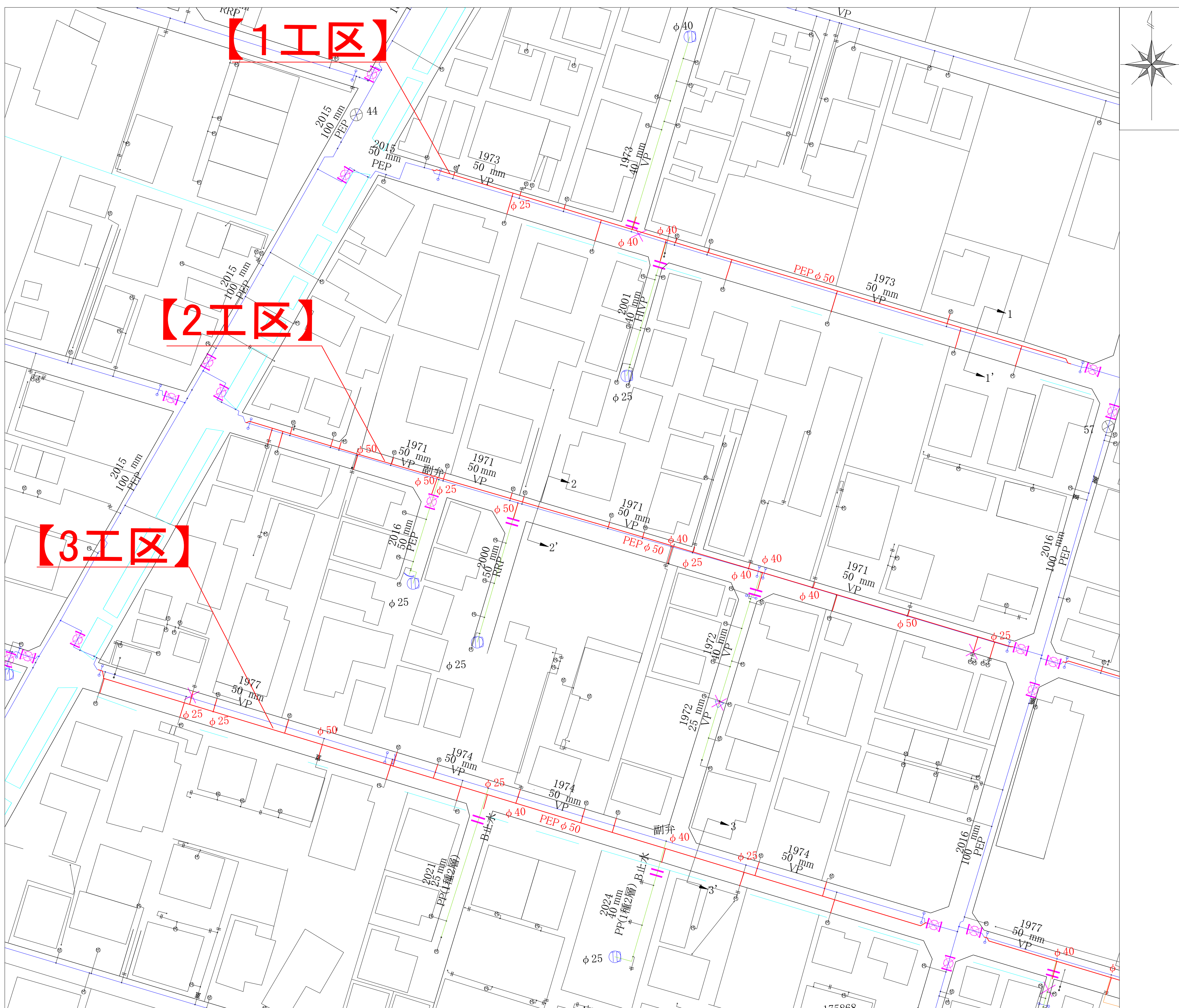
平面図 S=1/500 【1、2、3工区】
