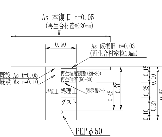
PEP φ 50土工図②
