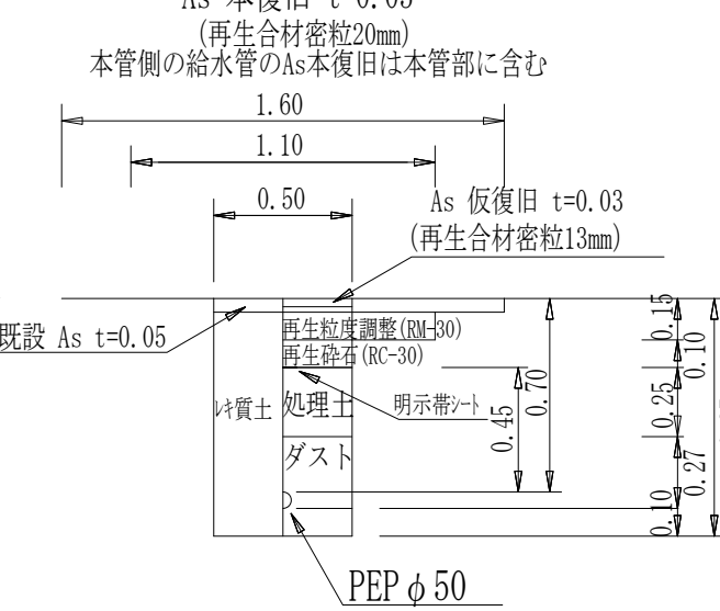
給水管 φ 50土工図①
