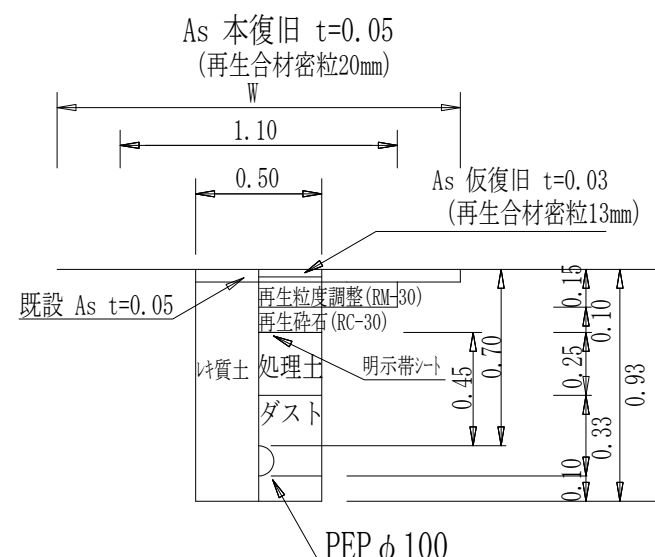
PEP φ 100土工図
