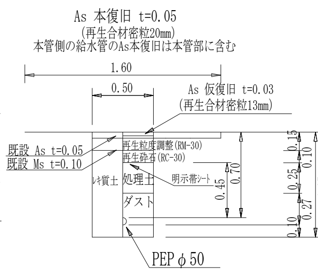
給水管 φ 50土工図②
