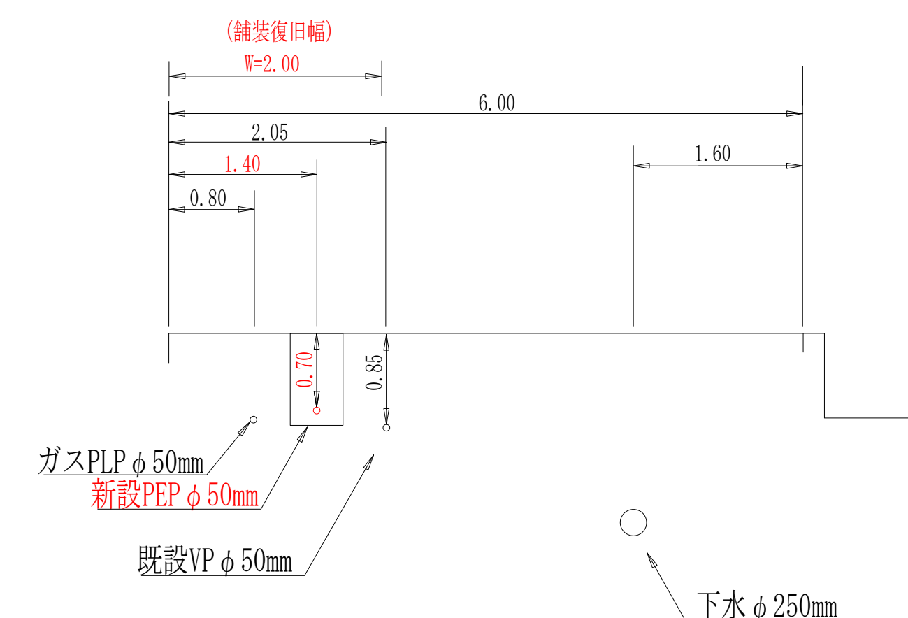
横断図 S=1/50 【1、2、3工区】
