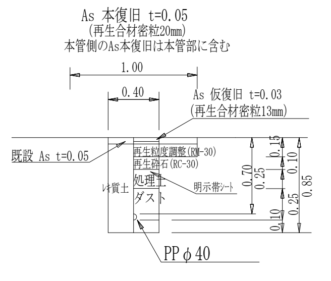
給水管 φ 40土工図①
