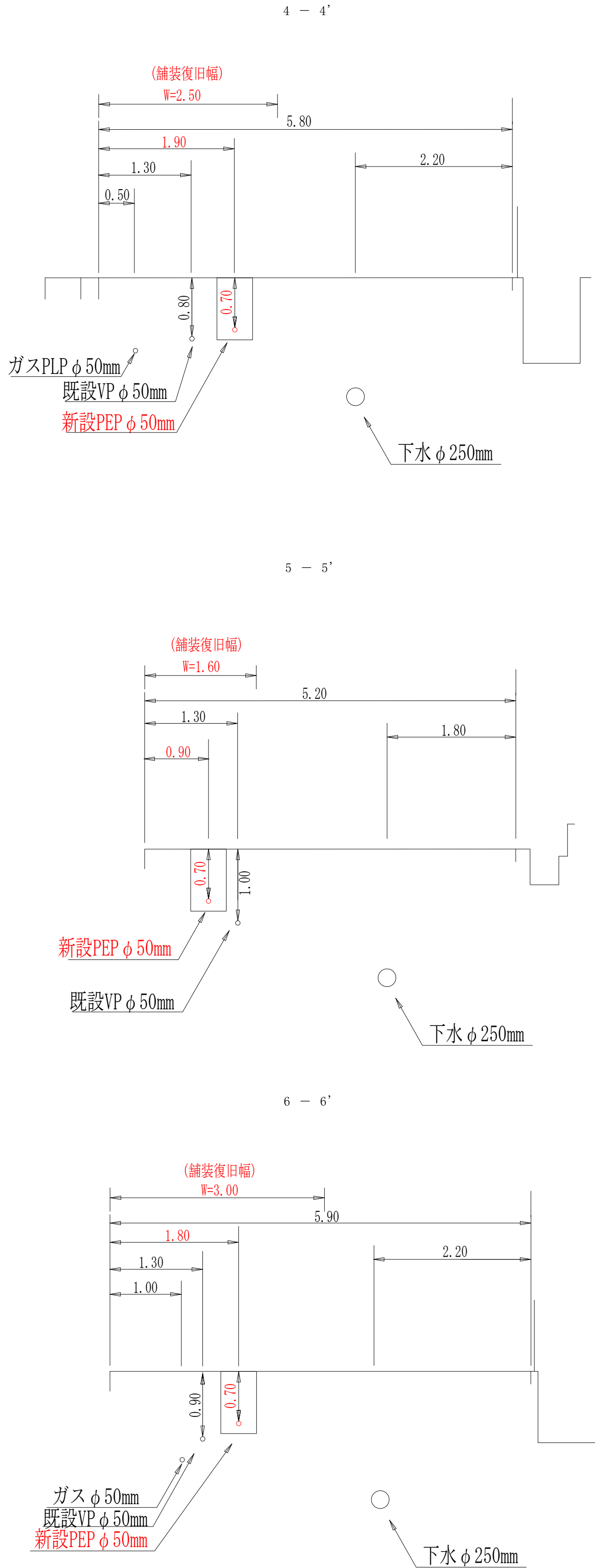
横断面 S=1/50【4、5、6工区】
