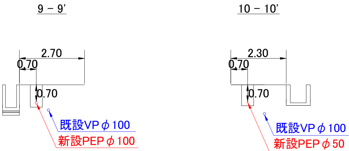
横断面図(2) S=1/100
