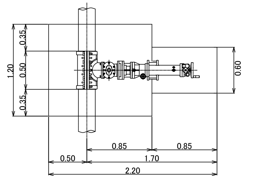
不断水分岐土工図 200×100 S=1/30
